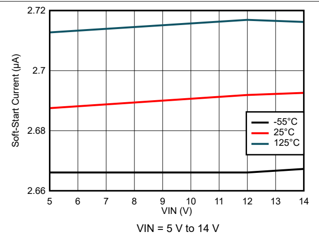
图 7-10. Soft-Start Current Variation
