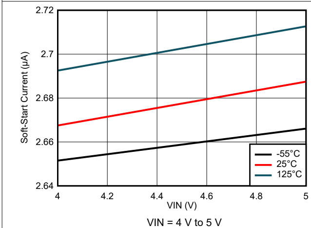
图 7-9. Soft-Start Current Variation
