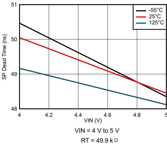
图 7-51. SP Dead Time Variation
