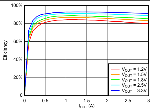
图 6-38. 在 VIN = 7V, fSW = 500kHz, 温度 = 25°C 条件下, 通道 1 在不同 VOUT 下的效率与负载间的关系
