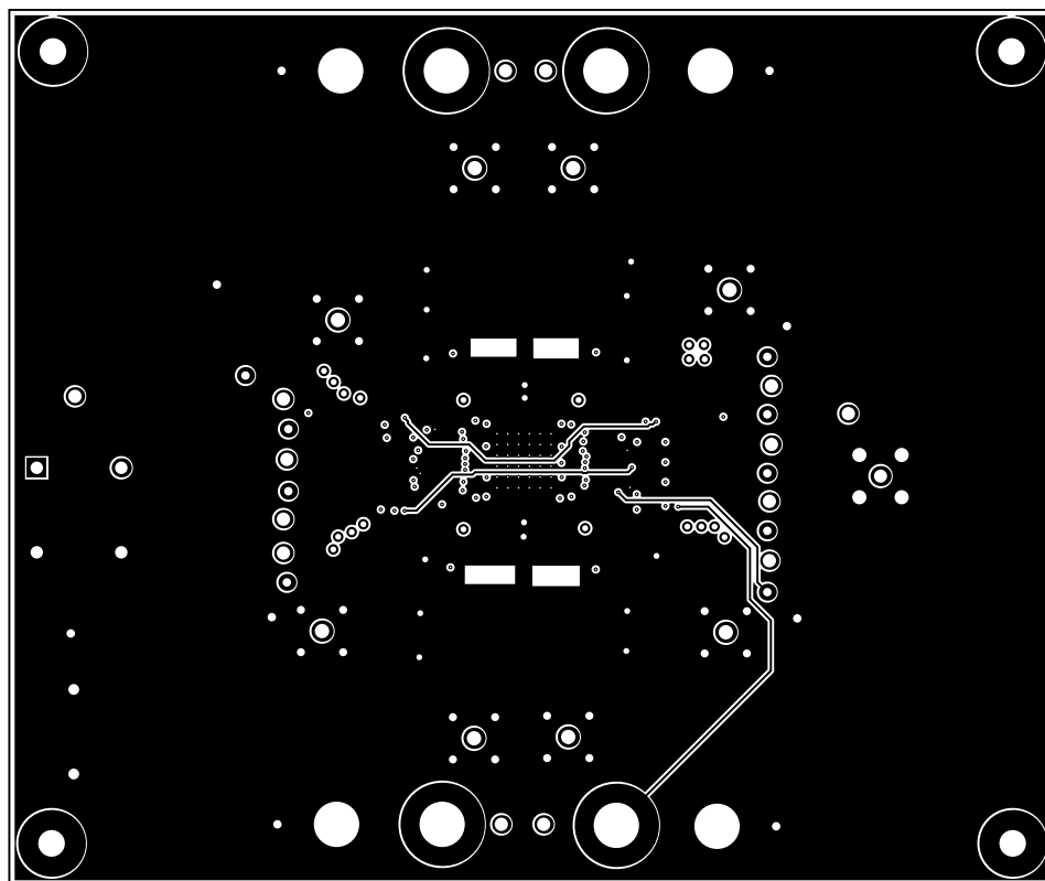
图 9-19. PCB 布局示例 (内层) 3
