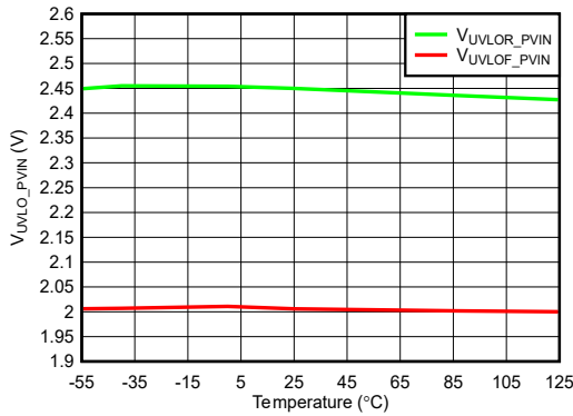
图 6-53. 上升与下降 PVIN UVLO 与温度之间的关系
