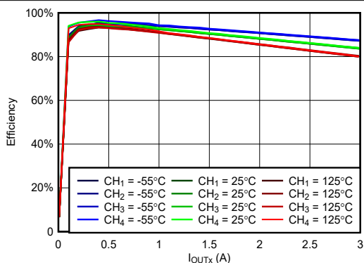
图 6-3. VIN = 3.3V, VOUTx = 1.5V, fSW = 100kHz 时, 效率与负载间的关系
