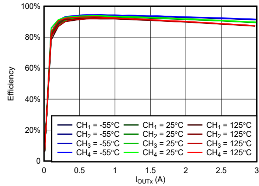
图 6-30. VIN = 5V, V OUTx = 2.5V, f SW = 500kHz 时, 效率与负载间的关系
