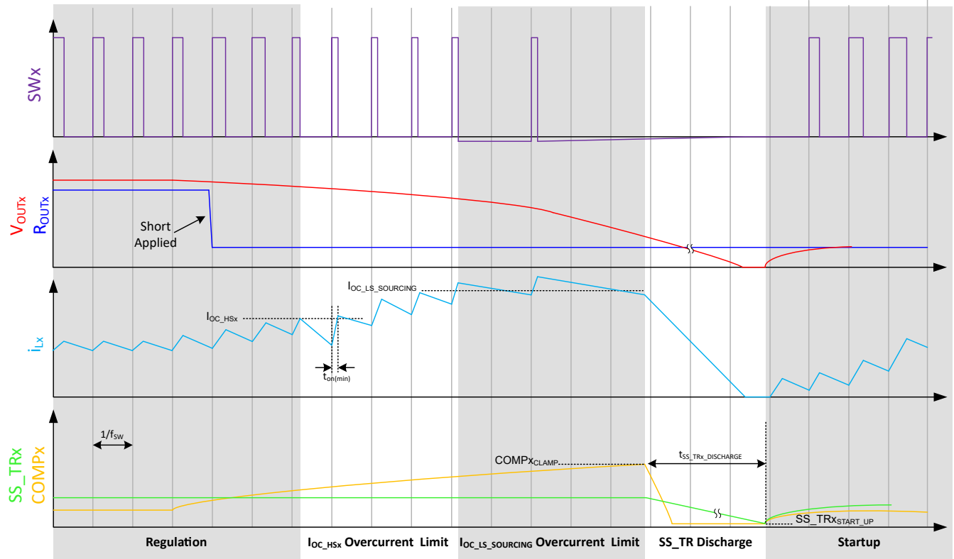
图 8-15. COMPx 钳位关断 (COMPx_CLAMP)
