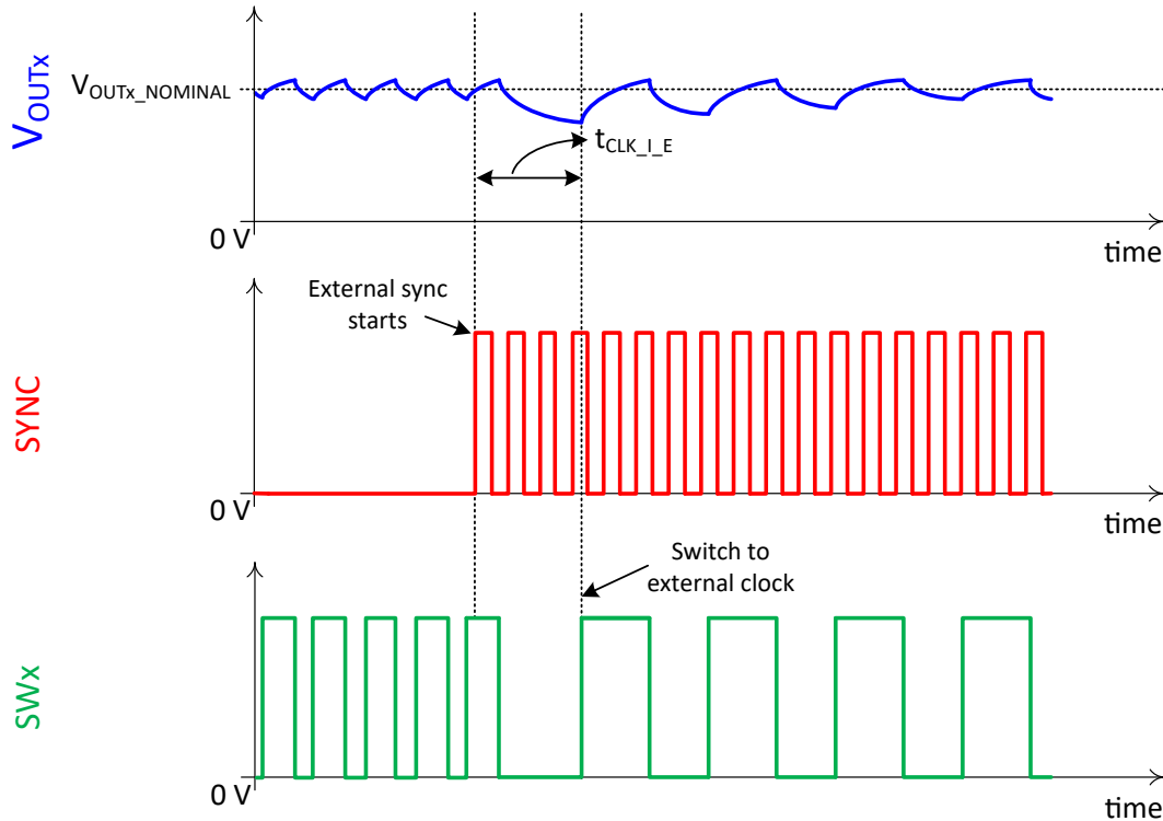
图 8-8. 内部至外部时钟转换
