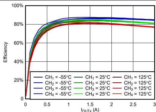
图 6-14. VIN = 7V, V OUTx = 1.2V, f SW = 100kHz 时, 效率与负载间的关系
