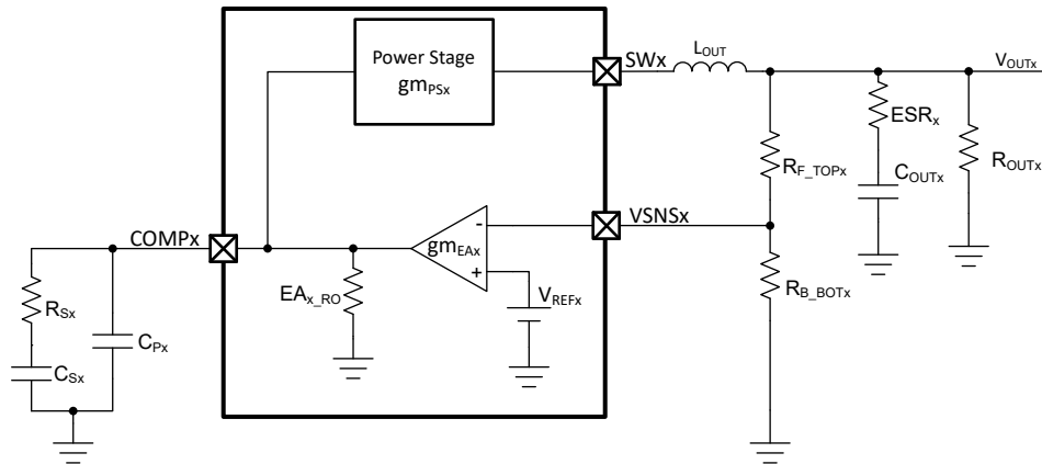
图 8-16. 闭环响应的简化小信号模型
