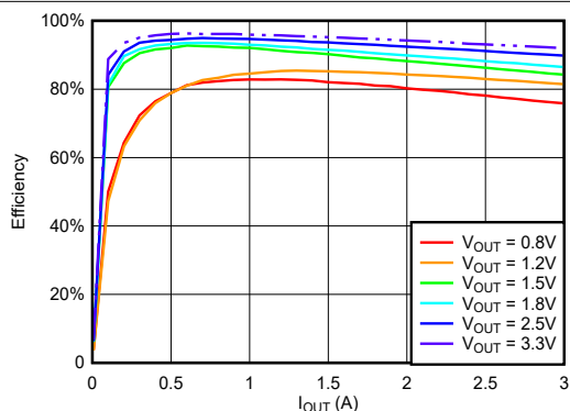
图 6-13. 在 VIN = 5V, f SW = 100kHz, 温度 = 25°C 条件下, 通道 1 在不同 V OUT 下的效率与负载间的关系
