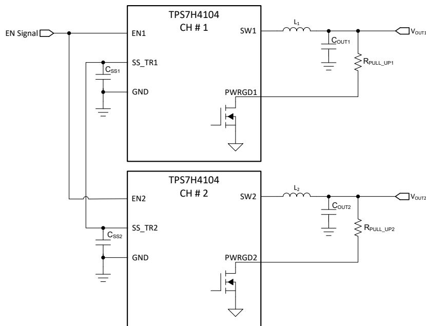
图 8-11. 比例式启动序列
