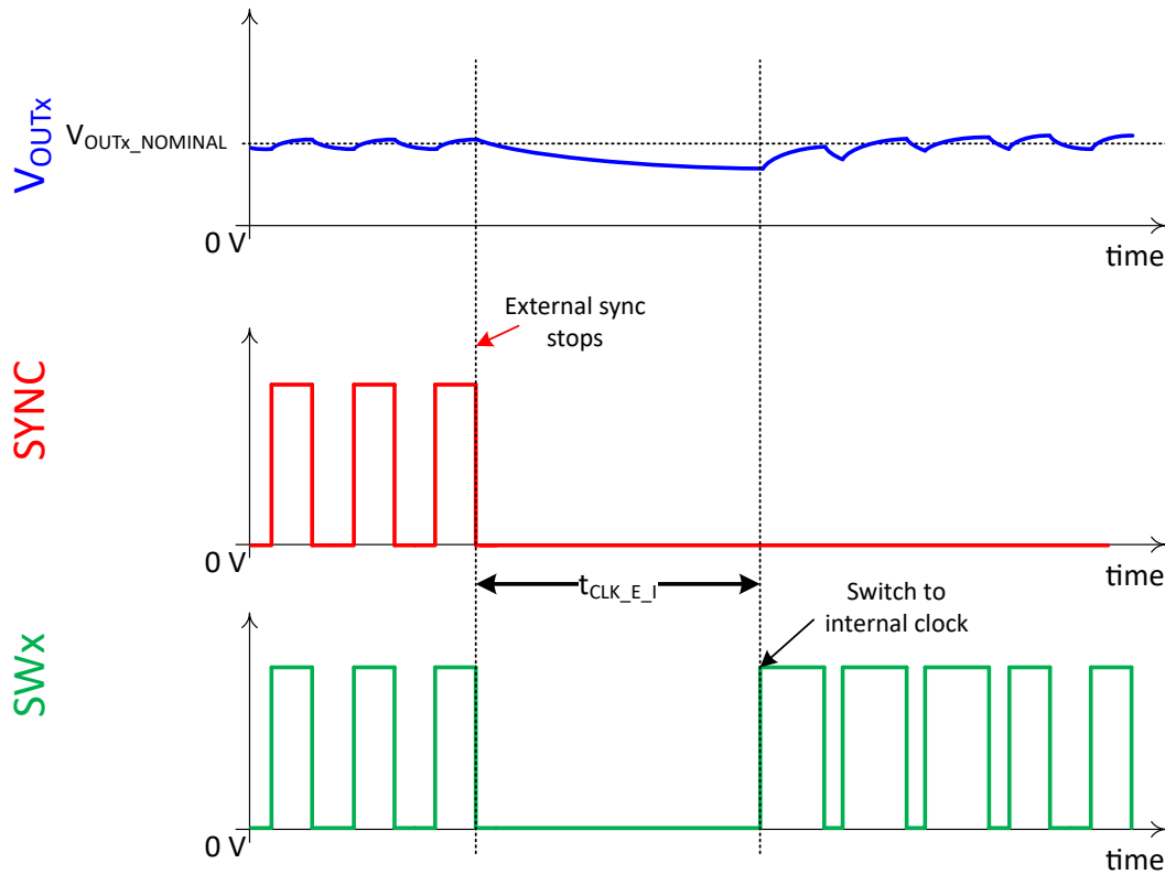
图 8-9. 外部至内部时钟转换
