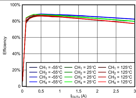
图 6-40. VIN = 3.3V, VOUTx = 1.5V, fSW = 1MHz 时, 效率与负载间的关系
