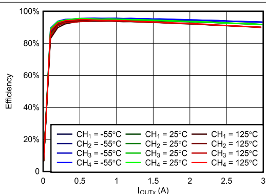
图 6-31. VIN = 5V, VOUTX = 3.3V, fSW = 500kHz 时, 效率与负载间的关系
