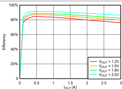
图 6-43. 在 V_{IN} = 3.3V , f_{SW} = 1MHz , 温度 = 25^{\circ}C 条件下, 通道 1 在不同 V_{OUT} 下的效率与负载间的关系
