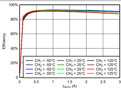
图 6-47. V_{IN} = 5V , V_{OUTX} = 3.3V , f_{SW} = 1MHz 时, 效率与负载间的关系
