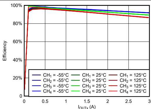
图 6-5. VIN = 3.3V, VOUTx = 2.5V, fSW = 100kHz 时, 效率与负载间的关系
