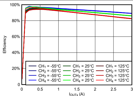
图 6-4. VIN = 3.3V, VOUTx = 1.8V, fSW = 100kHz 时, 效率与负载间的关系
