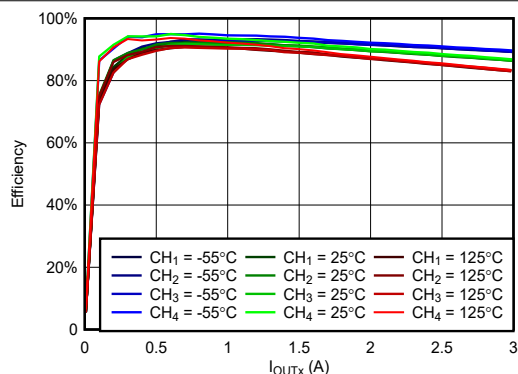
图 6-16. VIN = 7V, V OUTx = 1.8V, f SW = 100kHz 时, 效率与负载间的关系
