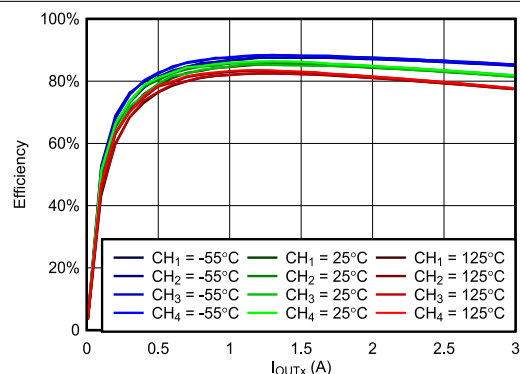
图 6-8. VIN = 5V, VOUTx = 1.2V, fSW = 100kHz 时, 效率与负载间的关系
