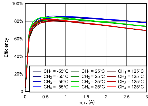
图 6-26. VIN = 5V, V OUTx = 0.8V, f SW = 500kHz 时, 效率与负载间的关系
