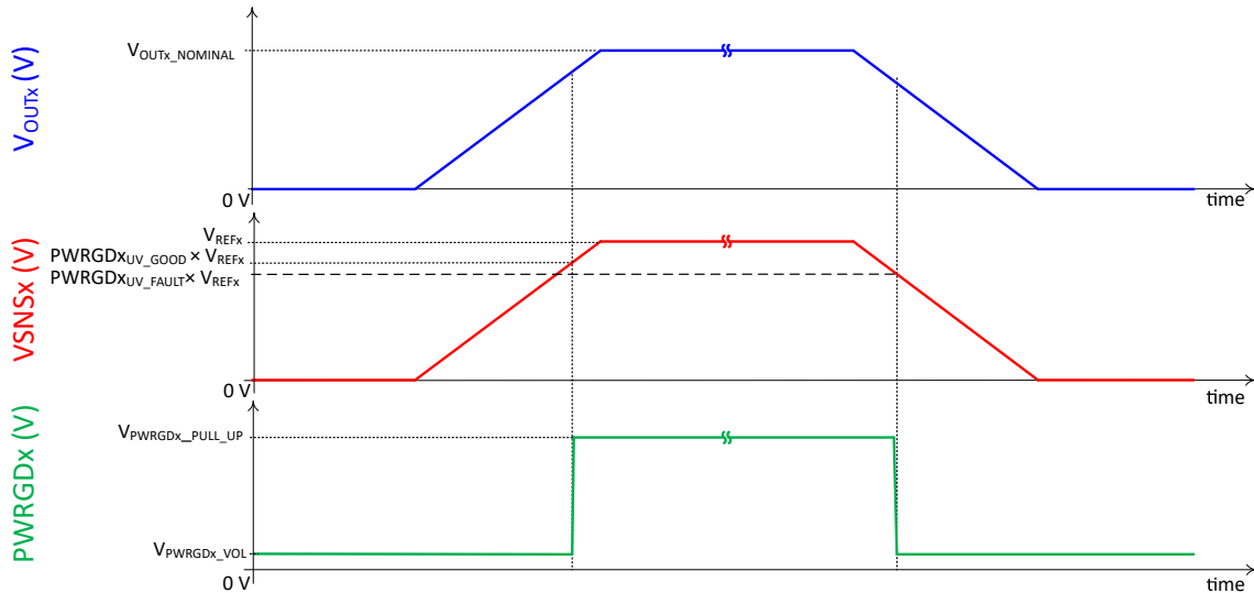
图 8-4. PWRGDx 欠压 (UV) 阈值
