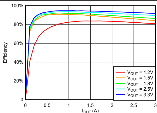
图 6-19. 在 V_{IN} = 7V , f_{SW} = 100kHz , 温度 = 25^{\circ}C 条件下, 通道 1 在不同 V_{OUT} 下的效率与负载间的关系
