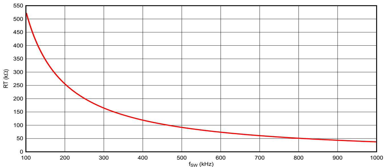
图 8-7. 标称 RT 与开关频率间的关系
