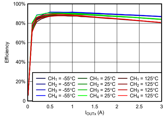
图 6-28. VIN = 5V, V OUTx = 1.5V, f SW = 500kHz 时, 效率与负载间的关系
