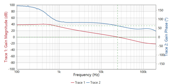
图 9-12. V_{OUT2} 完整环路波德图
