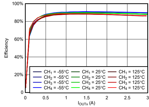
图 6-50. VIN = 7V, VOUTx = 3.3V, fSW = 1MHz 时, 效率与负载间的关系
