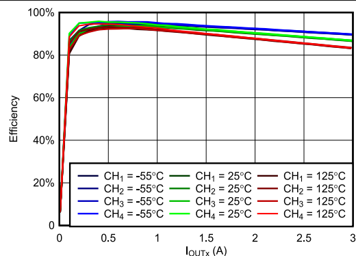
图 6-10. VIN = 5V, VOUTx = 1.8V, fSW = 100kHz 时, 效率与负载间的关系
