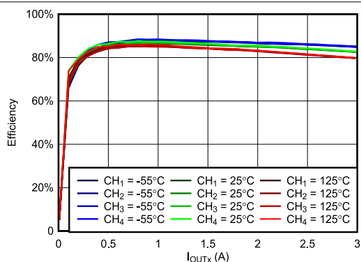
图 6-45. V_{IN} = 5V , V_{OUTX} = 1.8V , f_{SW} = 1MHz 时, 效率与负载间的关系
