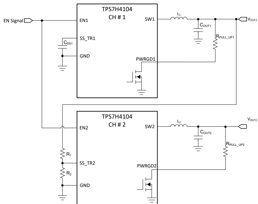
图 8-12. 比例式与同步启动序列
