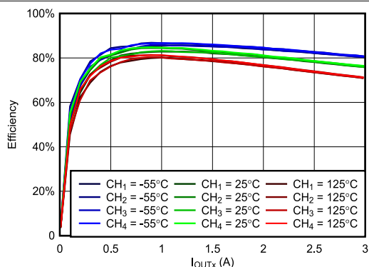
图 6-7. VIN = 5V, VOUTx = 0.8V, fSW = 100kHz 时, 效率与负载间的关系
