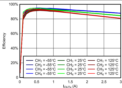
图 6-9. VIN = 5V, VOUTx = 1.5V, fSW = 100kHz 时, 效率与负载间的关系
