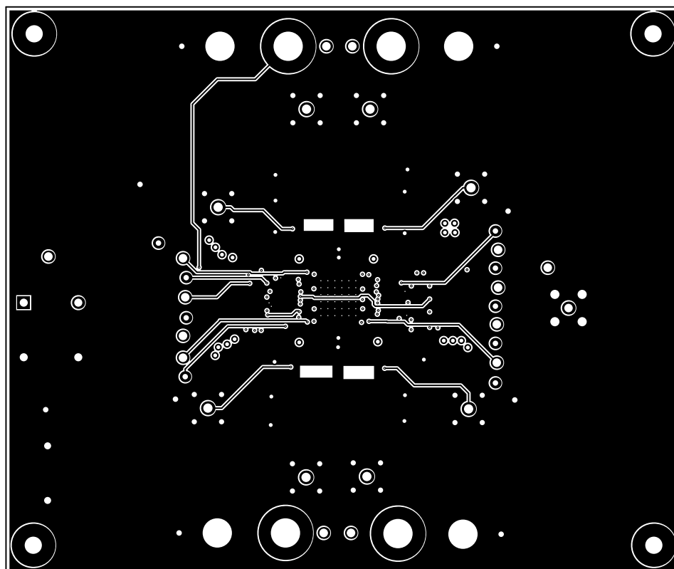
图 9-18. PCB 布局示例 ( 内层 ) 2
