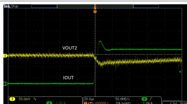
图 9-5. V_{OUT2} 满负载阶跃上升
