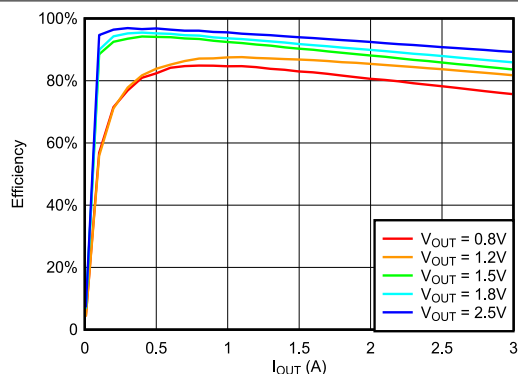
图 6-6. 在 VIN = 3.3V, fSW = 100kHz, 温度 = 25°C 条件下, 通道 1 在不同 VOUT 下的效率与负载间的关系
