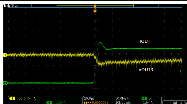
图 9-7. V_{OUT3} 满负载阶跃上升
