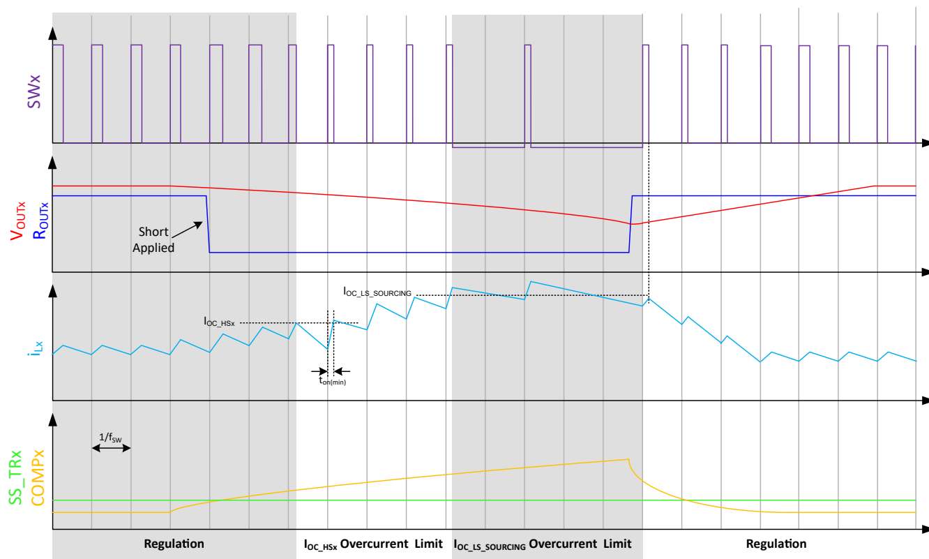
图 8-14. 低侧拉电流过流保护 ( I_{OC\_LS\_SOURCINGx} )
