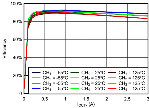
图 6-29. VIN = 5V, V OUTx = 1.8V, f SW = 500kHz 时, 效率与负载间的关系
