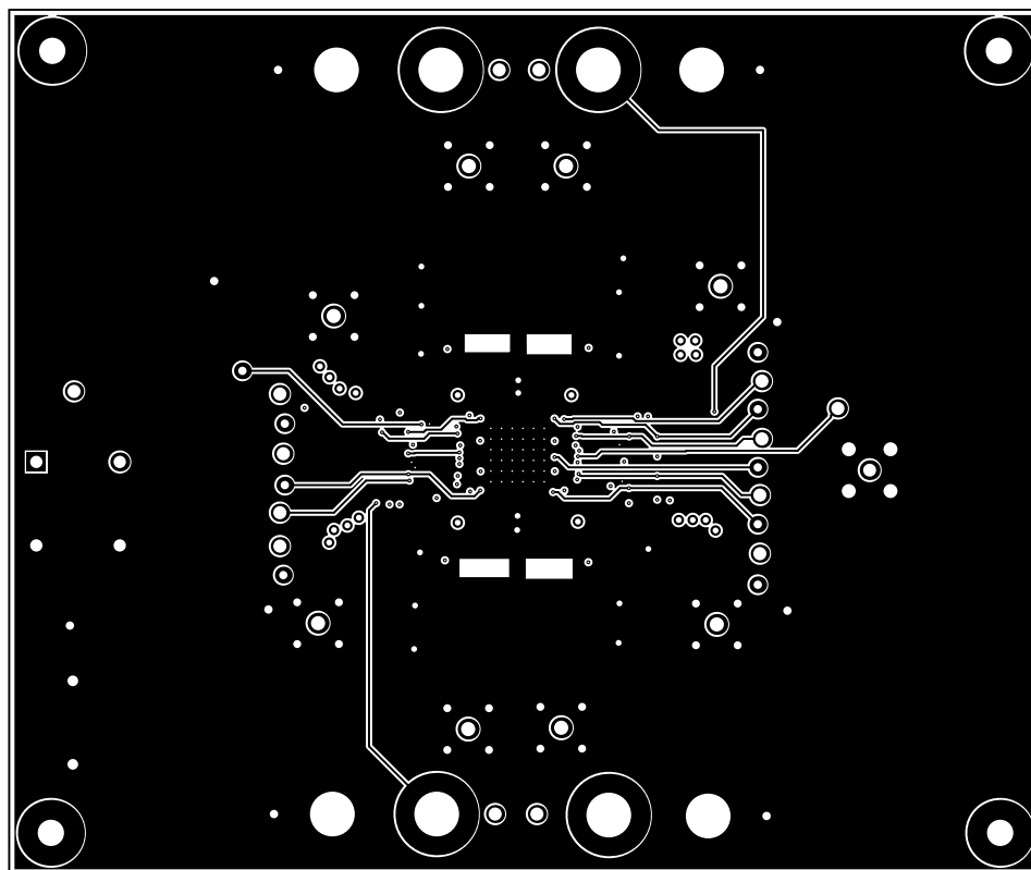
图 9-17. PCB 布局示例 ( 内层 ) 1
