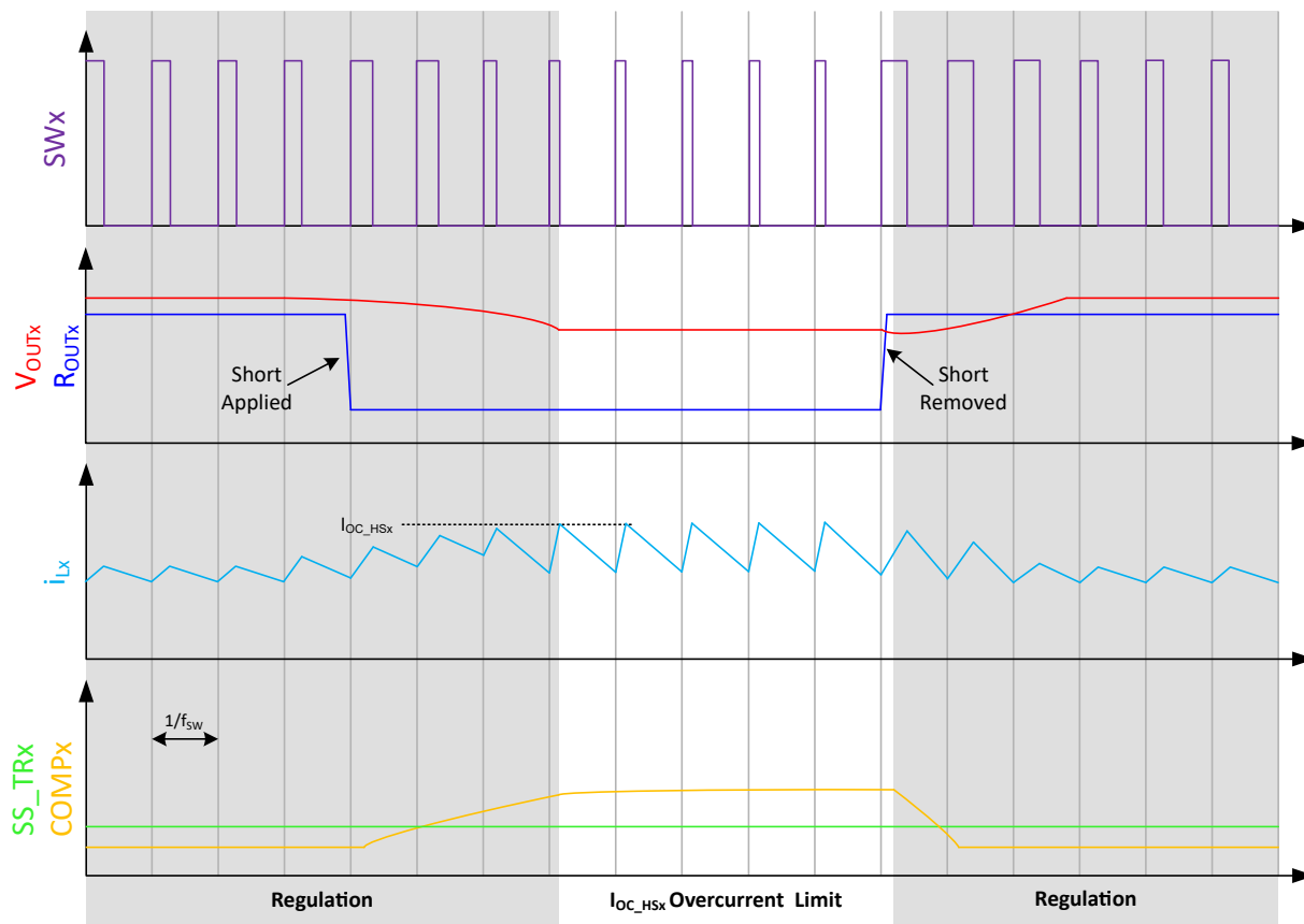
图 8-13. 高侧逐周期过流保护 ( I_{OC\_HSx} )
