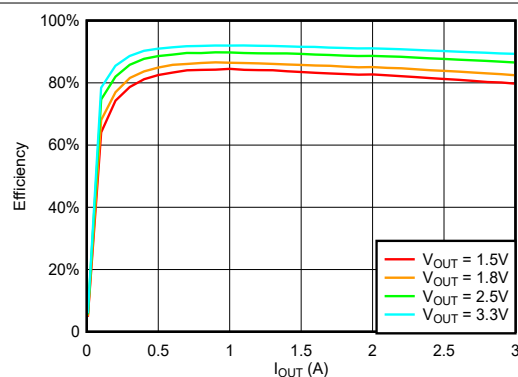
图 6-48. 在 V_{IN} = 5V , f_{SW} = 1MHz , 温度 = 25^{\circ}C 条件下, 通道 1 在不同 V_{OUT} 下的效率与负载间的关系
