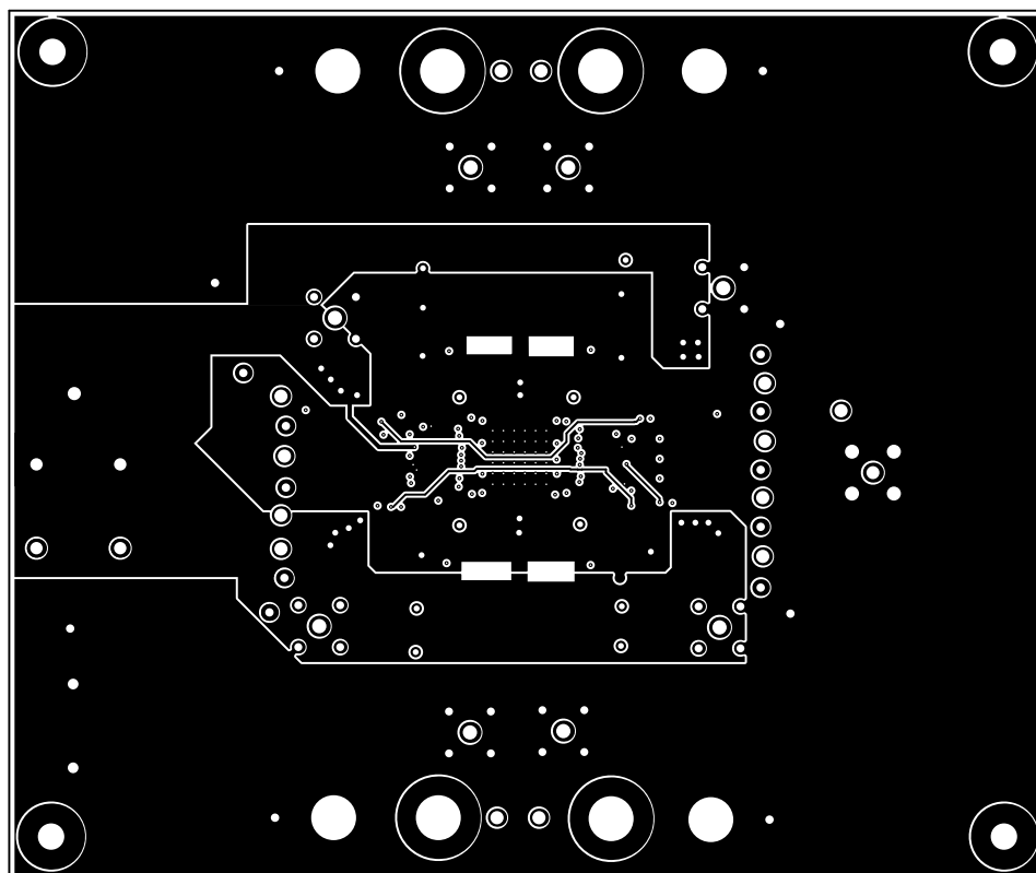
图 9-20. PCB 布局示例 (内层) 4
