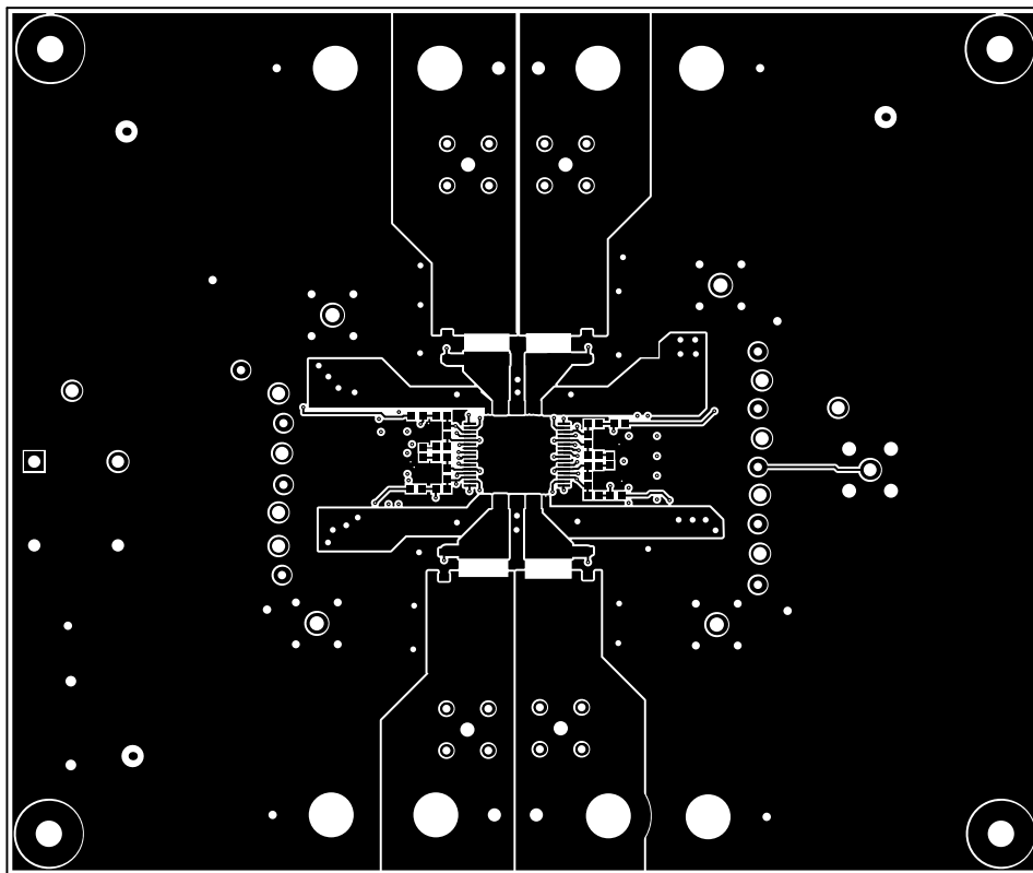
图 9-16. PCB 布局示例 ( 顶层 )
