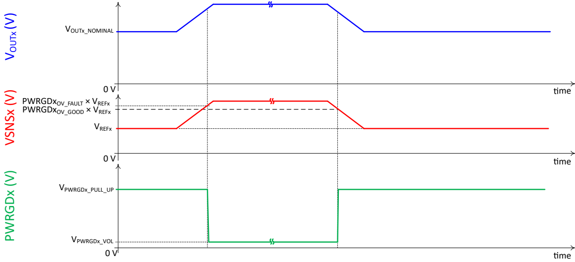
图 8-5. PWRGDx 过压 (OV) 阈值
