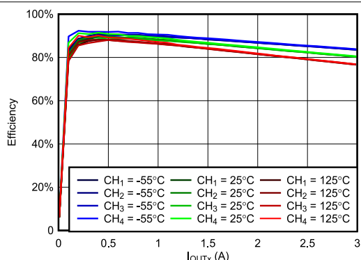
图 6-21. V_{IN} = 3.3V , V_{OUTX} = 1.2V , f_{SW} = 500kHz 时, 效率与负载间的关系
