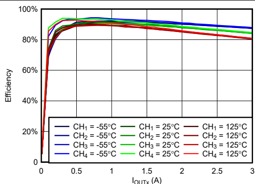
图 6-15. VIN = 7V, V OUTx = 1.5V, f SW = 100kHz 时, 效率与负载间的关系
