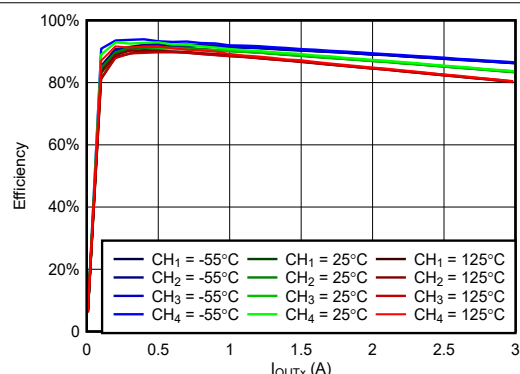
图 6-22. V_{IN} = 3.3V , V_{OUTX} = 1.5V , f_{SW} = 500kHz 时, 效率与负载间的关系
