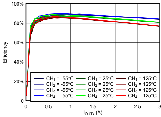
图 6-27. VIN = 5V, V OUTx = 1.2V, f SW = 500kHz 时, 效率与负载间的关系
