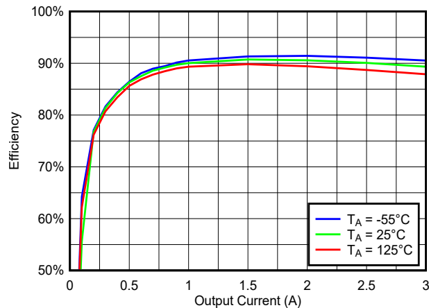
图 7-23. 500kHz、 V_{IN} = 12V 、 V_{OUT} = 5V 时 整个温度范围内的低电流效率与负载间的关系
