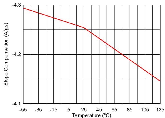
图 7-44. 500kHz 下斜率补偿与温度间的关系
