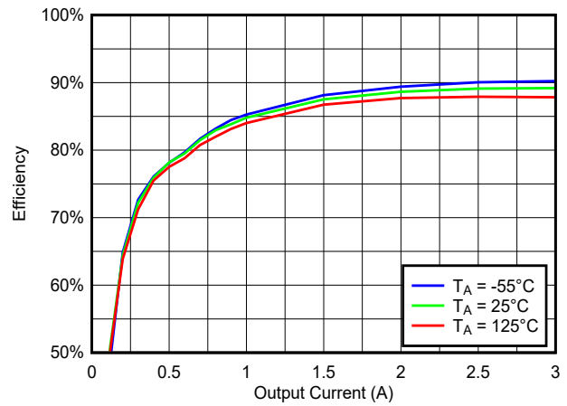
图 7-24. 500kHz、 V_{IN} = 12V 、 V_{OUT} = 2.5V 时 整个温度范围内的低电流效率与负载间的关系
