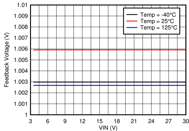
图 6-3. Feedback Voltage
