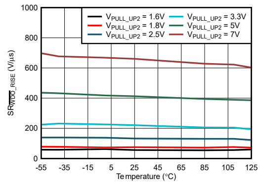
图 6-22. 不同 V_{PULL\_UP2} 下 S_{WDO\_RISE} 与温度间的关系
