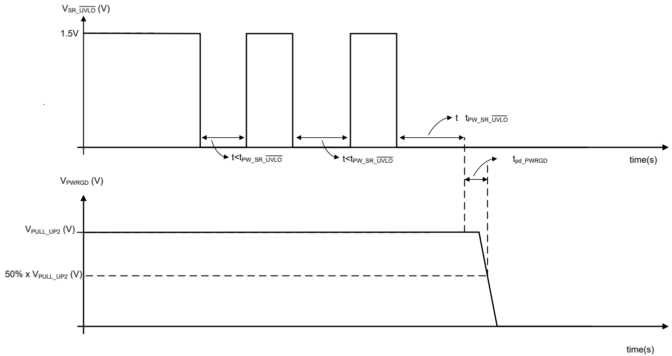
图 7-12. \overline{\text{SR\_UVLO}} 脉冲宽度 ( t_{\text{PW\_SR\_UVLO}} )
