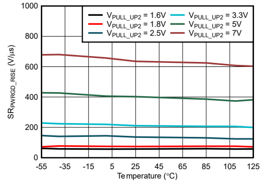
图 6-20. 不同 V_{PULL\_UP2} 下 S_{PWRGD\_RISE} 与温度间的关系
