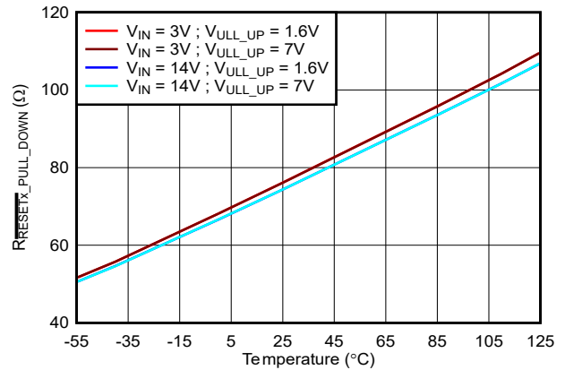
图 6-34. 对于 TPS7H3124, I_{LOAD} = 2mA 时, 不同 V_{PULL\_UP} 和 V_{IN} 下 RESET1 下拉电阻与温度间的关系
