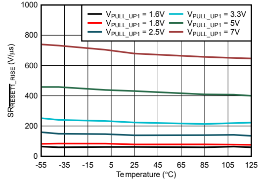
图 6-18. 不同 V_{PULL\_UP1} 下 S_{RESET1\_RISE} 与温度间的关系
