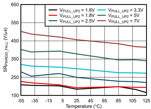
图 6-21. 不同 V_{PULL\_UP2} 下 S_{PWRGD\_FALL} 与温度间的关系
