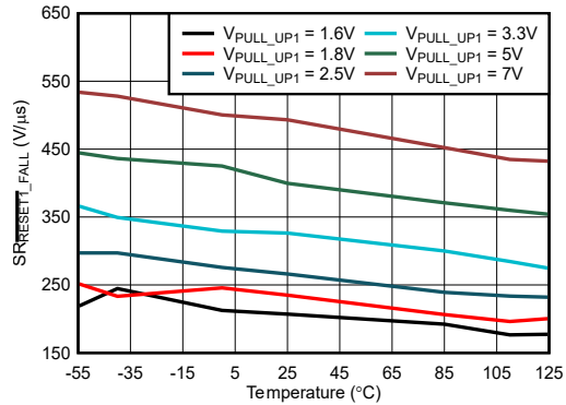
图 6-19. 不同 V_{PULL\_UP1} 下 S_{RESET1\_FALL} 与温度间的关系
