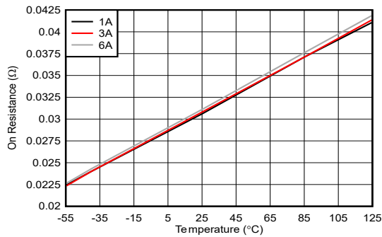
图 6-1. VIN = 1.5V 时 CFP 和 KGD 封装不同负载下导通电阻与温度间的关系
