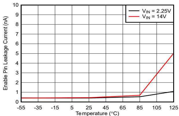
图 6-12. 使能引脚漏电流与温度间的关系
