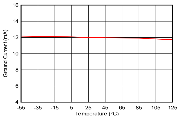
图 6-8. 接地电流与温度间的关系
