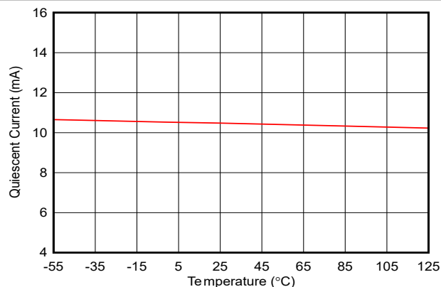
图 6-7. 静态电流与温度间的关系
