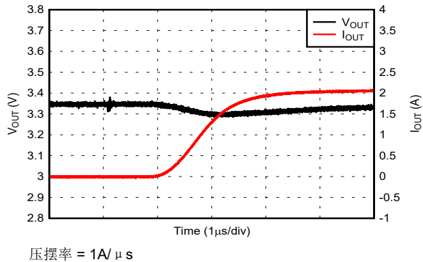
图 6-23. 负载阶跃: 0A 至 2A 且 V_{IN} = 5V
