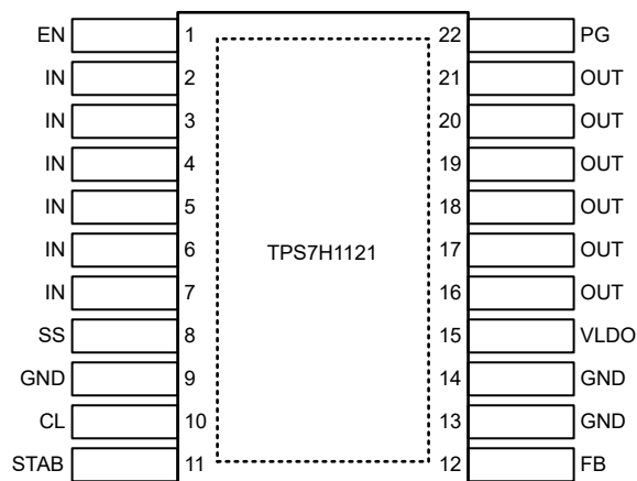
图 5-1. HFT 封装 22 引脚 CFP 顶视图
