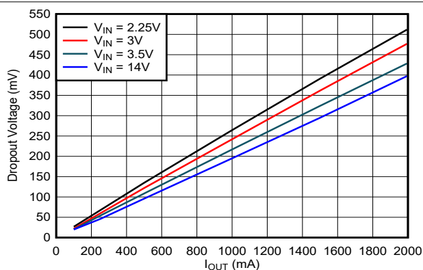
图 6-1. 压降电压与电流间的关系
