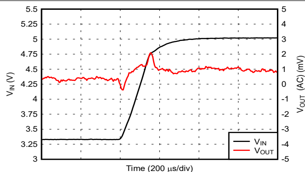
图 6-25. 线路阶跃：3.3V 至 5V，其中 I_{OUT} = 1.8A
