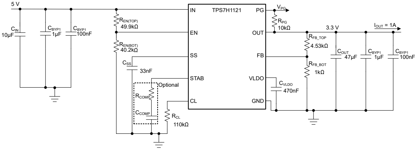
图 9-1. 应用原理图
