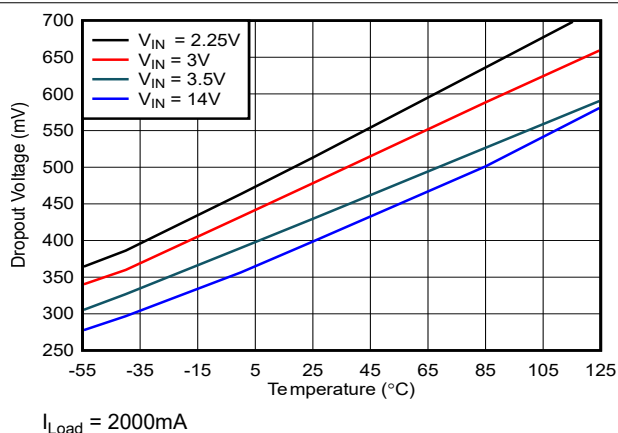
图 6-2. 压降电压与温度间的关系
