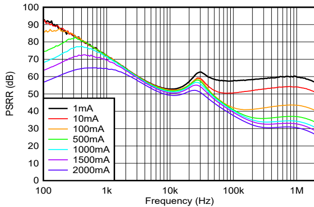
图 6-21. 不同电流下 PSRR 与频率间的关系
