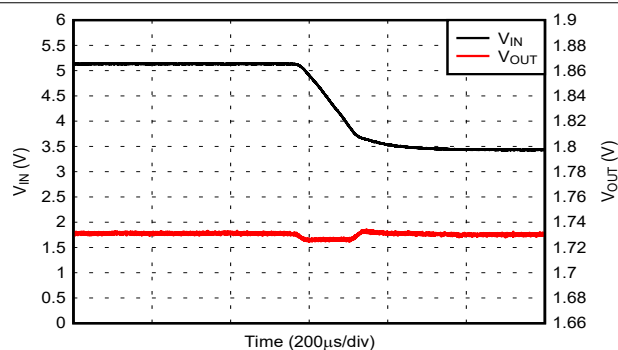
图 6-26. 线路阶跃：5V 至 3.3V，其中 I_{OUT} = 1.8A
