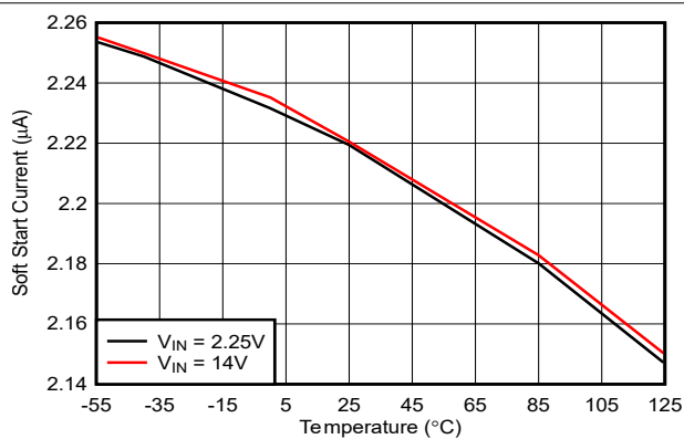
图 6-14. 软启动电流与温度间的关系
