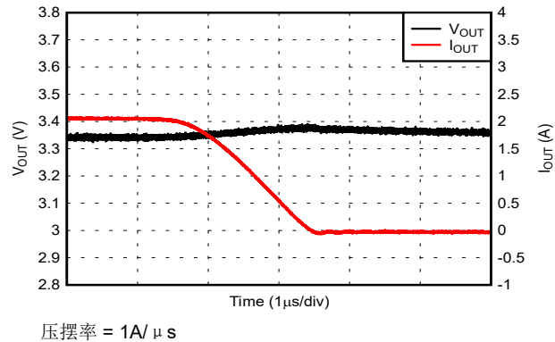
图 6-24. 负载阶跃 2A 至 0A 且 V_{OUT} = 5V
