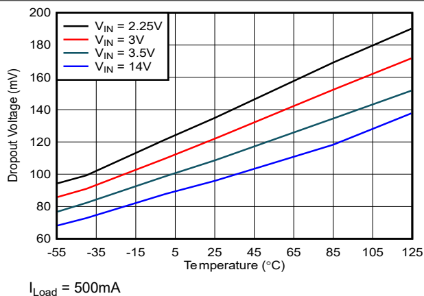
图 6-5. 压降电压与温度间的关系
