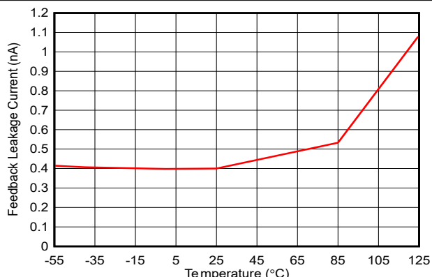
图 6-10. 反馈引脚漏电流与温度间的关系
