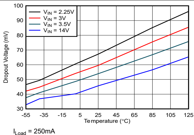
图 6-6. 压降电压与温度间的关系
