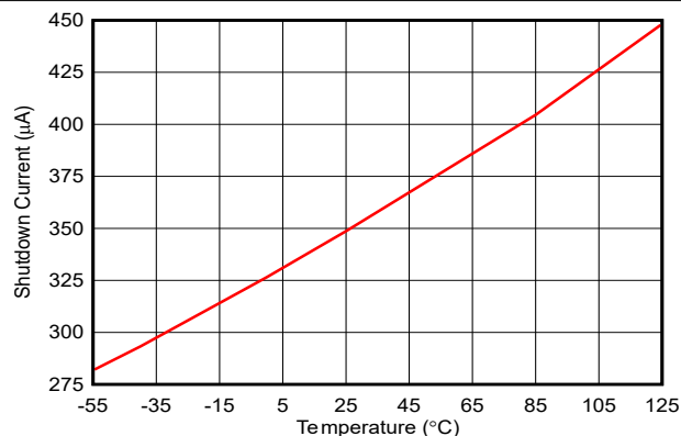
图 6-9. 关断电流与温度间的关系
