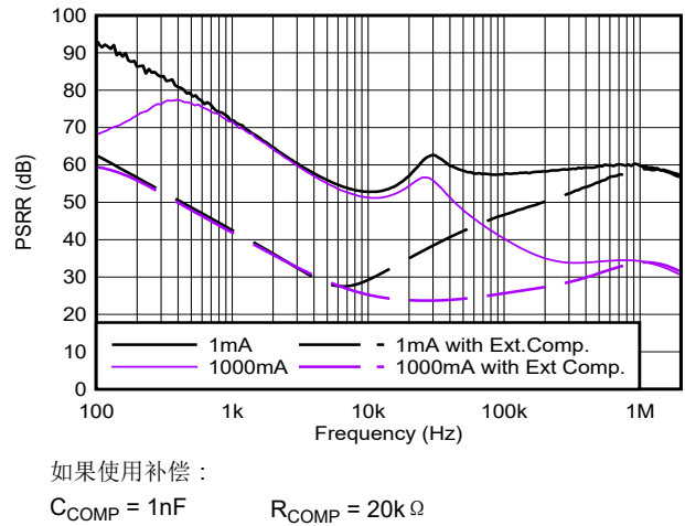
图 6-22. PSRR 与频率间的关系, 外部补偿比较
