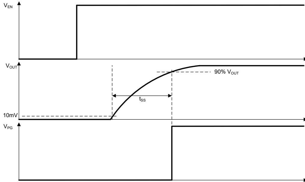
图 7-5. 软启动时间
