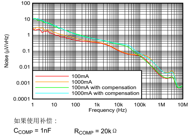
图 6-20. 输出噪声与频率间的关系, 外部补偿比较 (噪声频谱密度)
