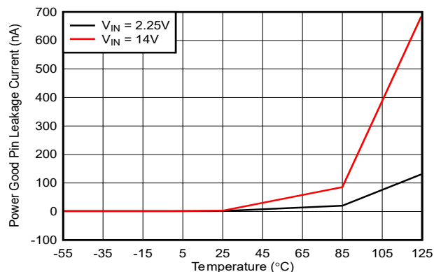
图 6-11. 电源正常引脚漏电流与温度间的关系
