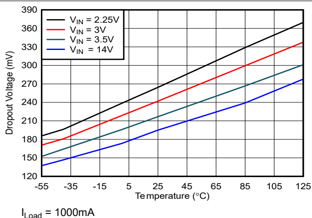
图 6-4. 压降电压与温度间的关系
