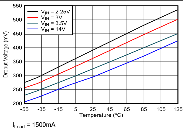
图 6-3. 压降电压与温度间的关系
