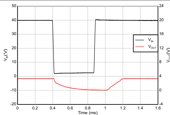
图 5-40. 压降恢复
