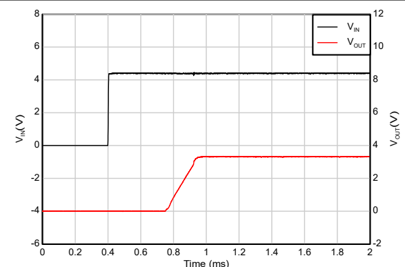
图 5-46. 按时序启动 (IN 在 EN 之后)
