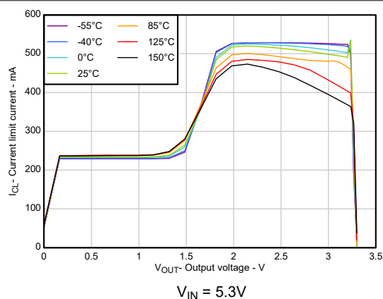
图 5-10. 电流限制与输出电压间的关系
