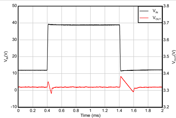
图 5-31. 线路瞬态
