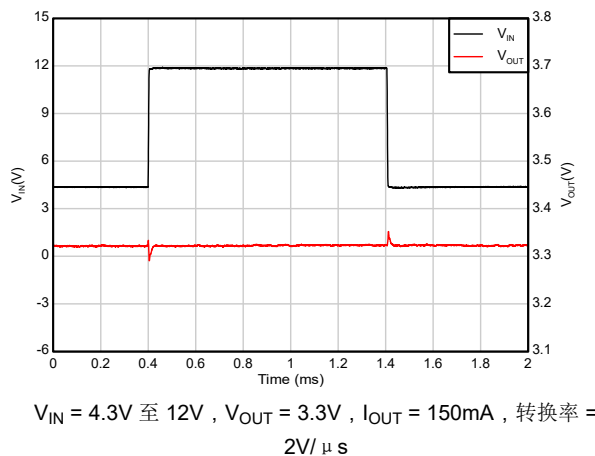
图 5-30. 线路瞬态
