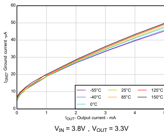
图 5-12. 接地电流与输出电流间的关系
