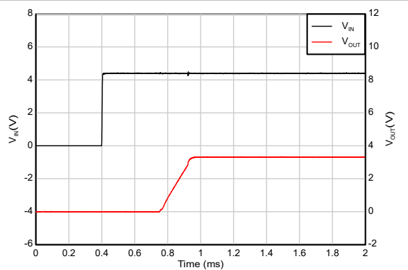
图 5-49. IN 与 EN 引脚短接启动
