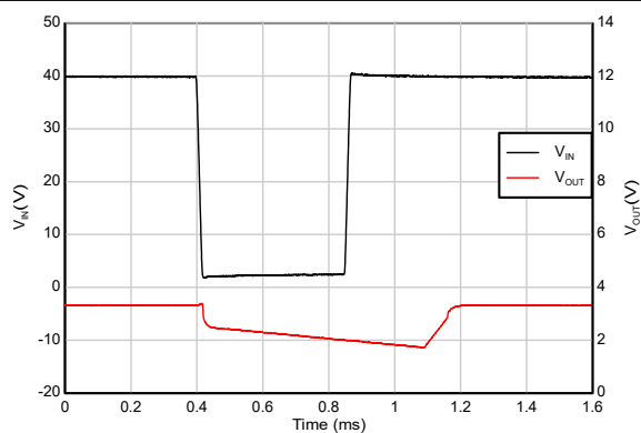
图 5-41. 欠压恢复
