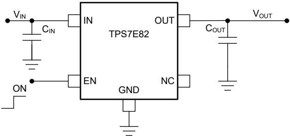
图 7-4. TPS7E82 典型应用电路（固定电压版本）
