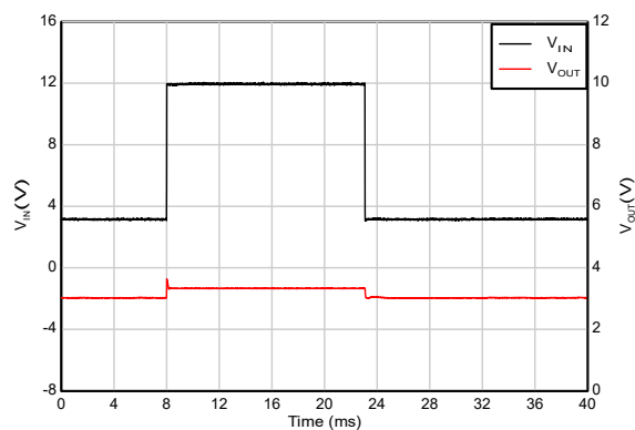
图 5-33. 冷启动恢复
