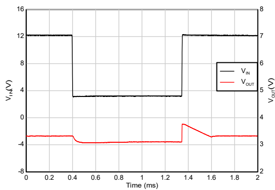
图 5-39. 压降恢复
