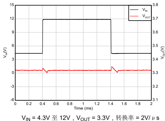
图 5-29. 线路瞬态
