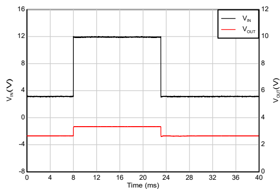
图 5-32. 线路瞬态
