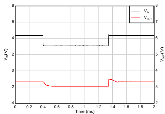
图 5-37. 压降恢复
