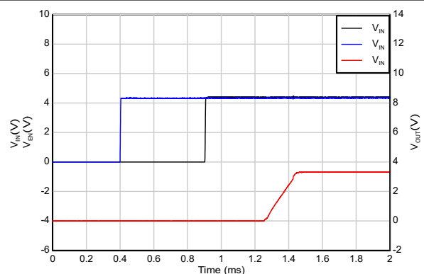
图 5-45. 按时序启动 (EN 在 IN 之后)
