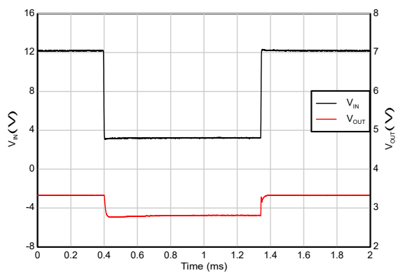
图 5-38. 压降恢复
