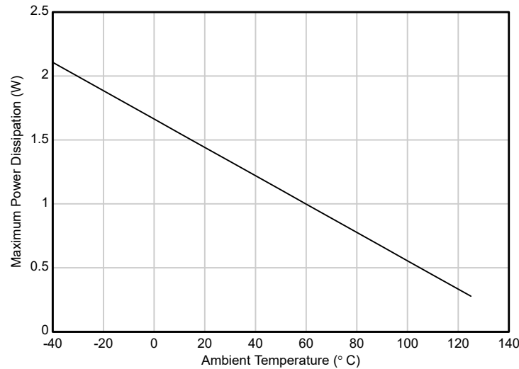
图 7-3. TPS7E82 (DRV) 允许的功率耗散
