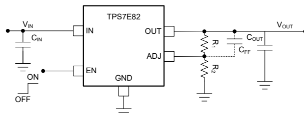
典型应用
