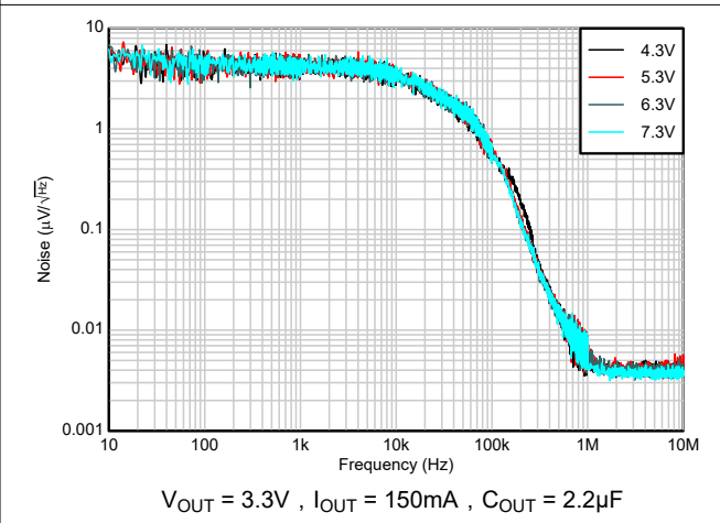
图 5-24. 噪声与 V_{IN} 间的关系
