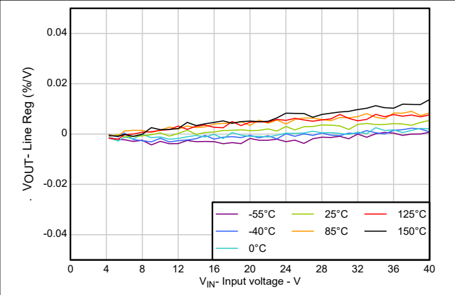
图 5-4. 线路调整率
