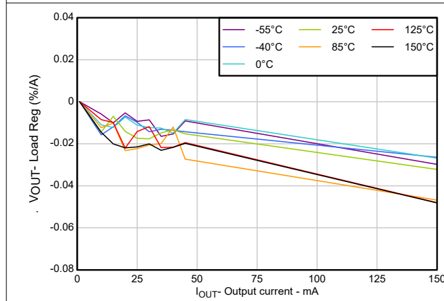
图 5-5. 负载调整率
