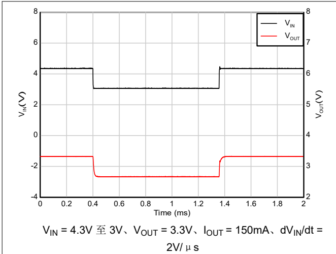
图 5-45. 压降恢复 (4.3V 至 3V)
