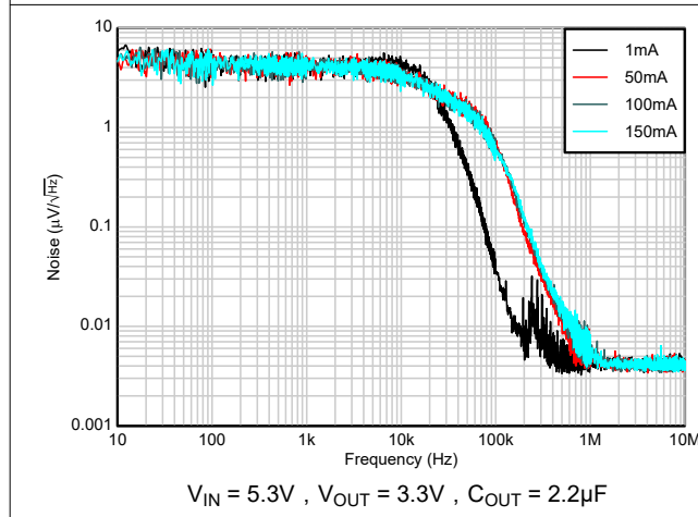
图 5-23. 噪声与 I_{OUT} 间的关系
