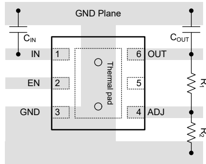
图 7-22. DRV 封装的布局示例
