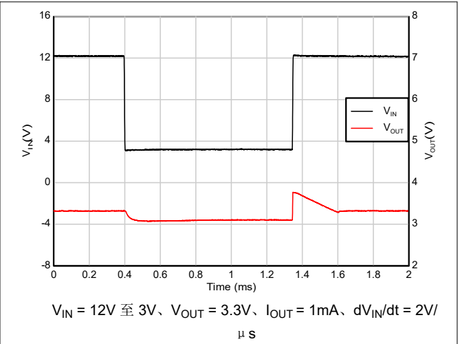
图 5-46. 压降恢复 (12V 至 3V)
