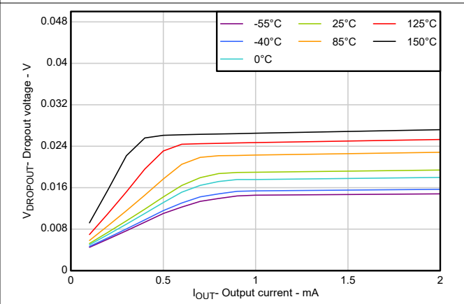
图 5-6. V_{DO} 与 I_{OUT} (mA) 间的关系
