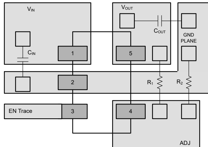
图 7-20. DBV 封装的布局示例
