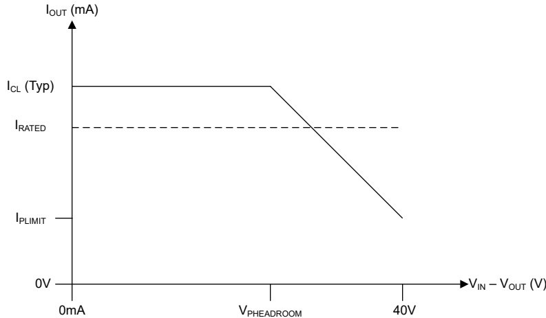
图 6-6. 功率限制
