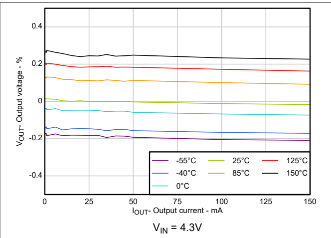
图 5-2. V_{OUT} 精度与 I_{OUT} 间的关系
