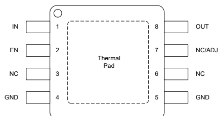
图 4-5. DGN 封装 (固定/ADJ), 8-引脚 HVSSOP (顶视图)
