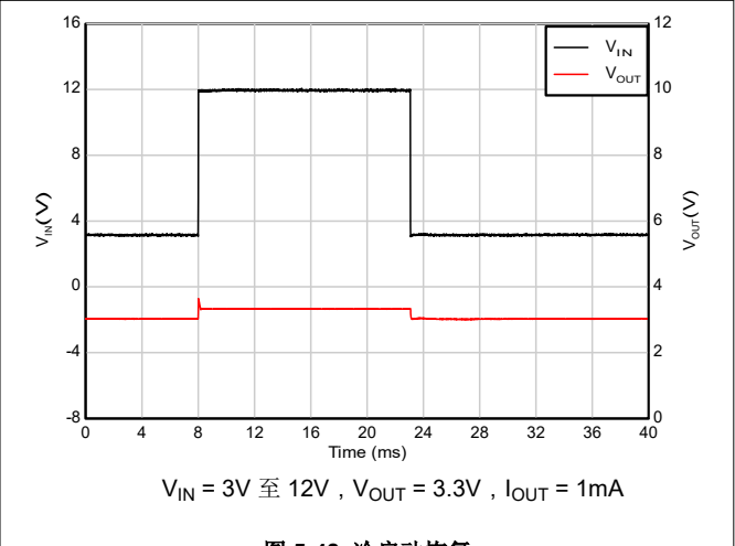
图 5-48. 冷启动恢复
