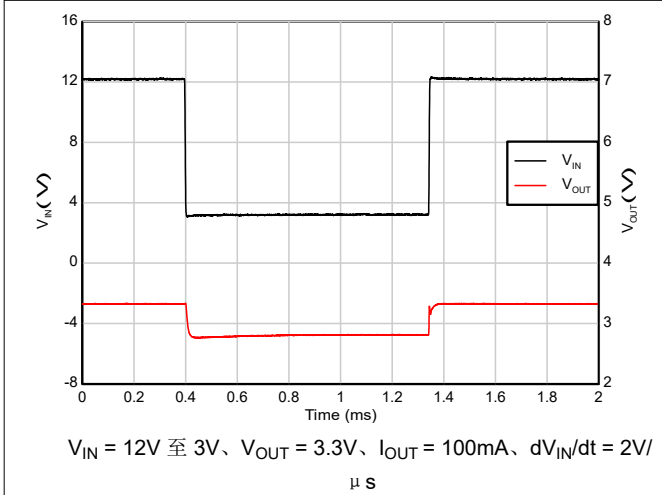
图 5-47. 压降恢复 (12V 至 3V)
