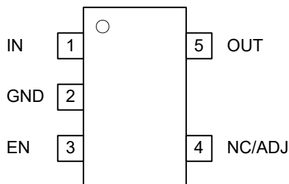
图 4-3. DBV 封装 (固定/ADJ), 5 引脚 SOT-23 (顶视图)
