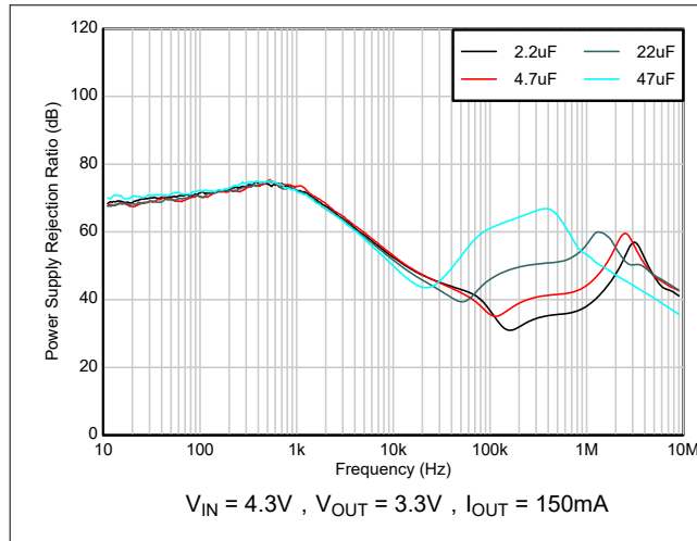
图 5-21. PSRR 与 C_{OUT} 间的关系
