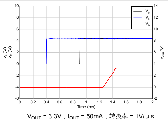
图 7-9. 时序启动 (IN 在 EN 之后)
