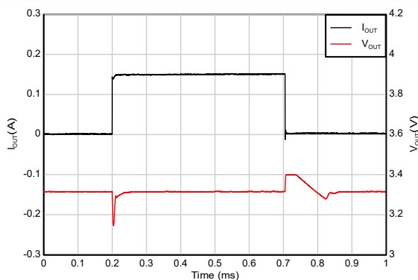
图 5-35. 负载瞬态
