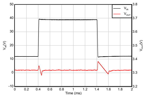
图 5-31. 线路瞬态
