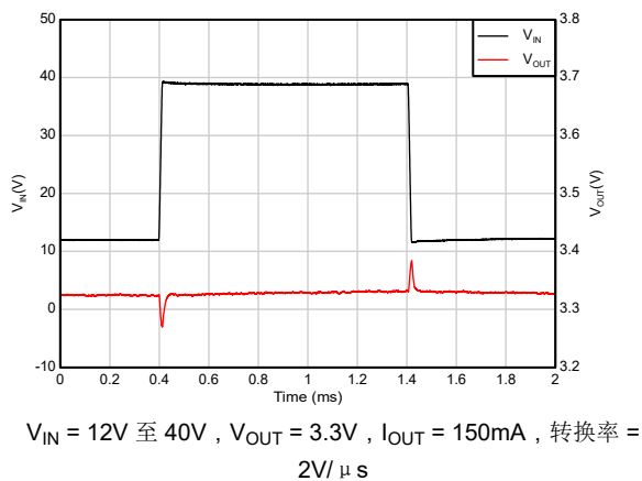
图 7-6. 线路瞬态
