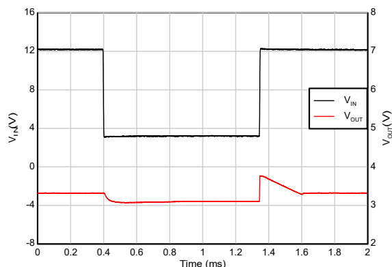
图 5-39. 压降恢复
