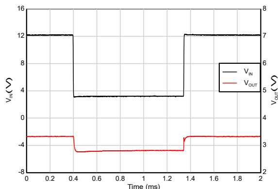
图 5-38. 压降恢复
