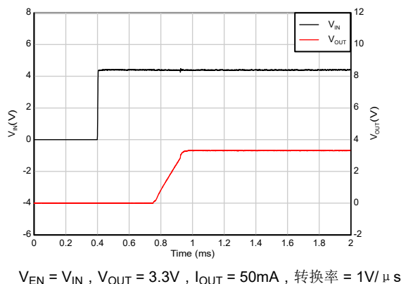
图 7-10. IN 与 EN 引脚短接启动
