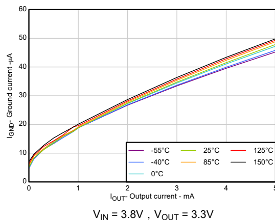
图 5-12. 接地电流与输出电流间的关系
