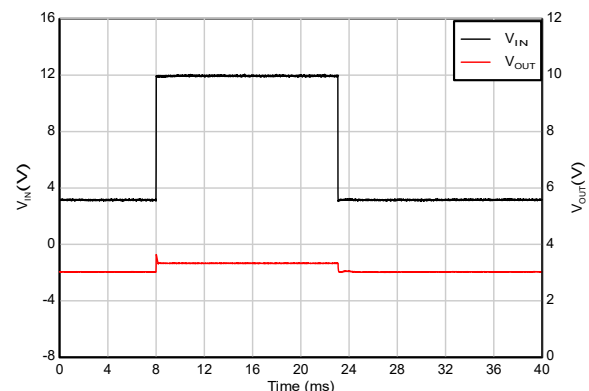
图 5-33. 冷启动恢复
