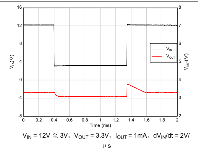
图 5-48. 压降恢复 (12V 至 3V)
