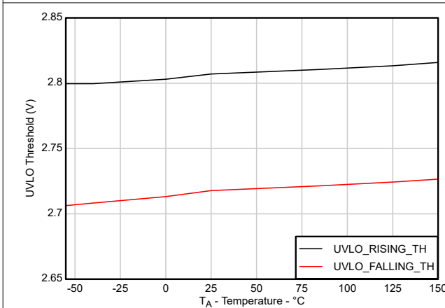
图 5-17. UVLO 阈值 ( V_{UVLO+}/V_{UVLO-} ) 与温度间的关系
