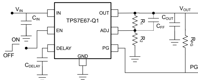
图 7-4. TPS7E67-Q1 可调节 LDO 稳压器编程
