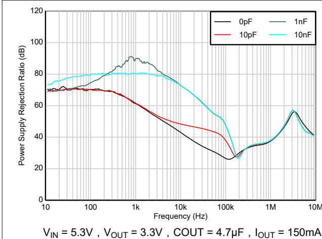
图 5-25. PSRR 与 C_{FF} 间的关系
