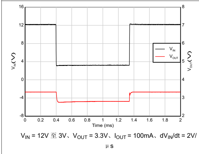
图 5-49. 压降恢复 (12V 至 3V)
