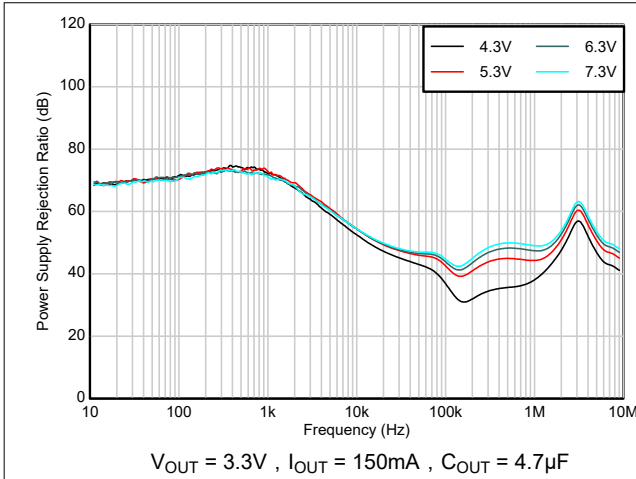
图 5-23. PSRR 与 V_{IN} 间的关系
