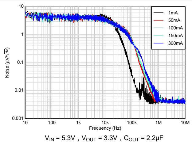
图 5-26. 噪声与 I_{OUT} 间的关系
