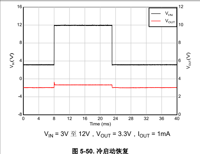
图 5-50. 冷启动恢复
