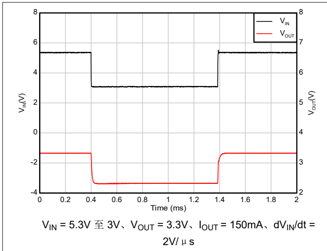
图 5-47. 压降恢复 (5.3V 至 3V)
