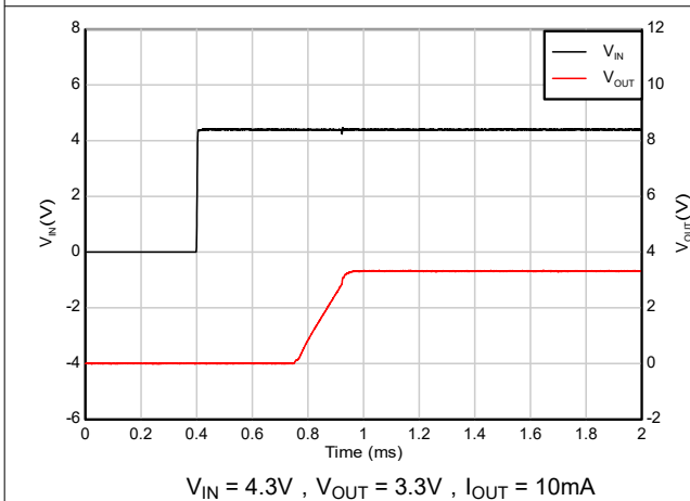
图 5-33. EN 与 V_{IN} 引脚短接启动
