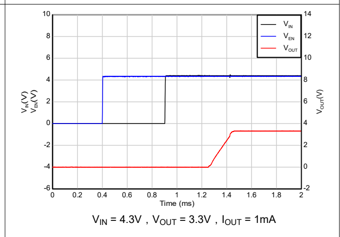
图 5-38. 时序启动 ( V_{IN} 在 EN 之后)
