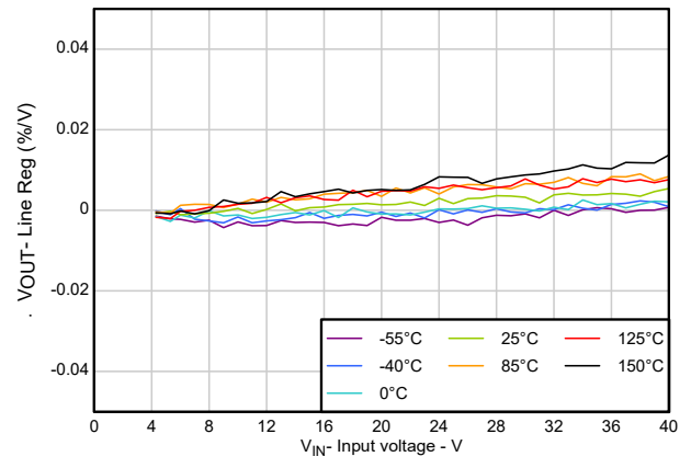
图 5-4. 线性调整率
