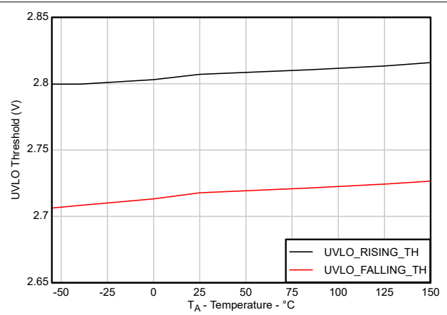
图 5-14. UVLO 阈值 ( V_{UVLO+}/V_{UVLO-} ) 与温度间的关系
