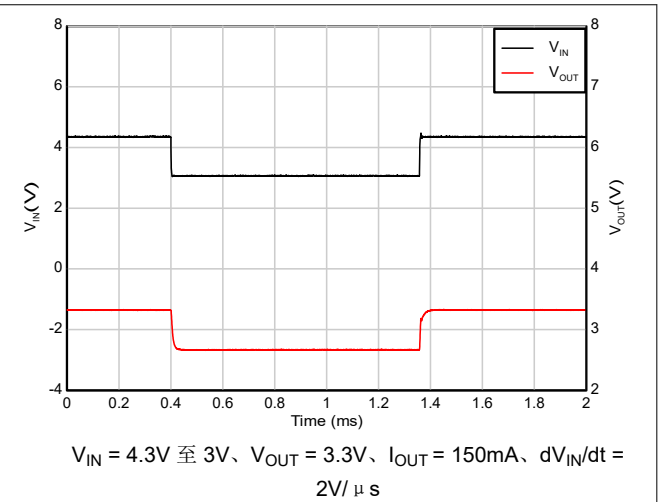
图 5-50. 压降恢复 (4.3V 至 3V)
