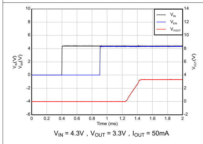
图 5-37. 时序启动 (EN 在 V_{IN} 之后)
