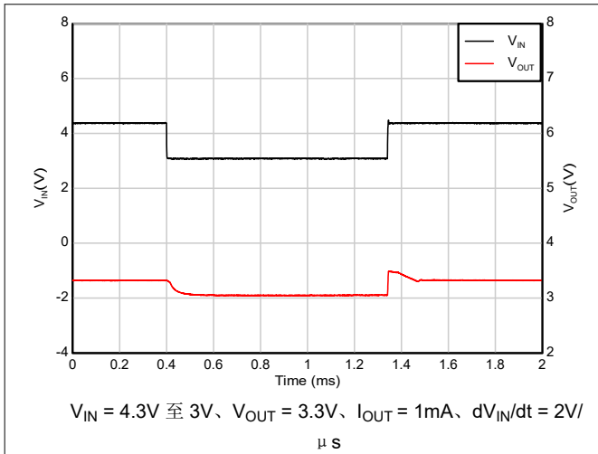
图 5-49. 压降恢复 (4.3V 至 3V)
