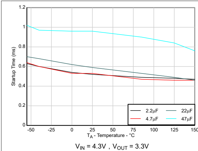
图 5-21. 启动时间与 C_{OUT} 间的关系
