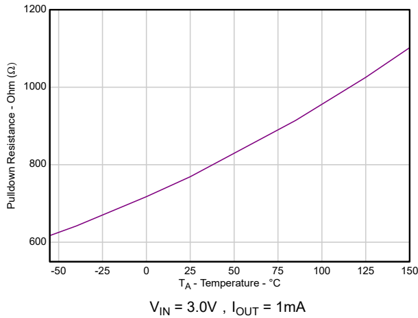
图 5-17. 输出端的下拉电阻 ( R_{\text{Discharge}} ) 与温度间的关系
