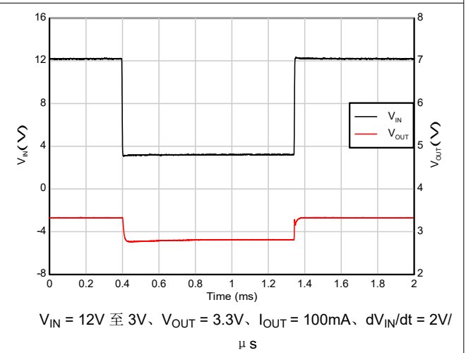
图 5-52. 压降恢复 (12V 至 3V)
