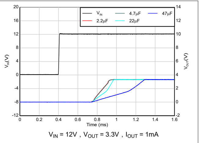
图 5-30. 启动与 C_{OUT} 间的关系
