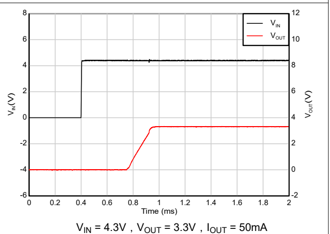
图 5-34. EN 与 V_{IN} 引脚短接启动
