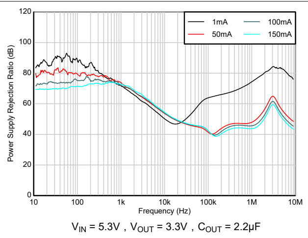
图 5-22. PSRR 与 I_{OUT} 间的关系
