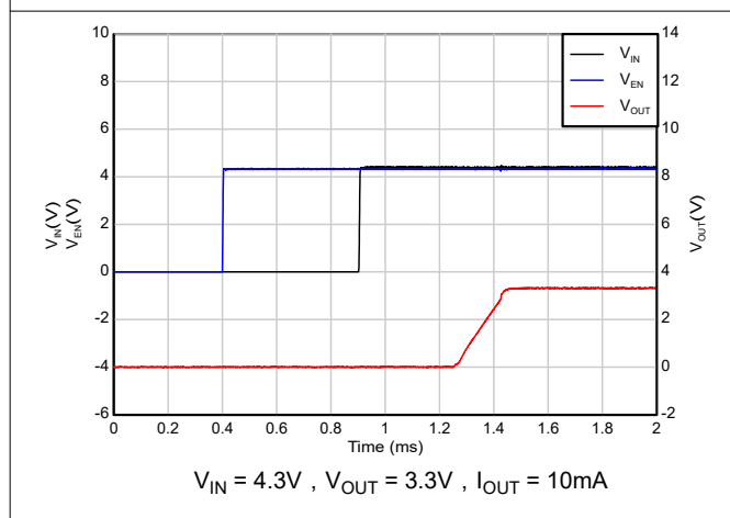
图 5-39. 时序启动 ( V_{IN} 在 EN 之后)
