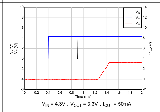
图 5-40. 时序启动 ( V_{IN} 在 EN 之后)
