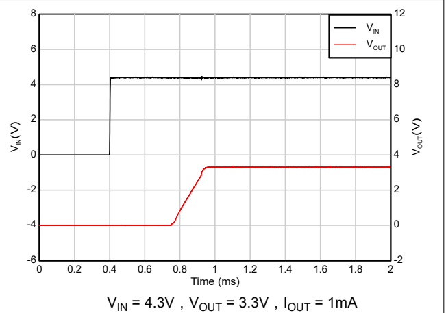
图 5-32. EN 与 V_{IN} 引脚短接启动
