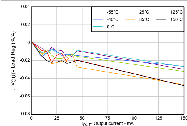
图 5-5. 负载调整率
