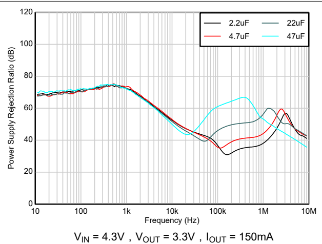
图 5-24. PSRR 与 C_{OUT} 间的关系
