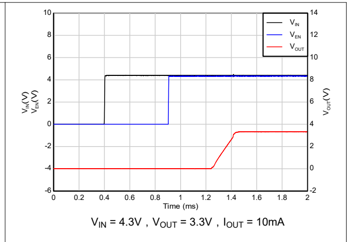
图 5-36. 时序启动 (EN 在 V_{IN} 之后)
