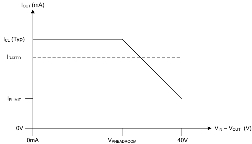
图 6-5. 功率限制
