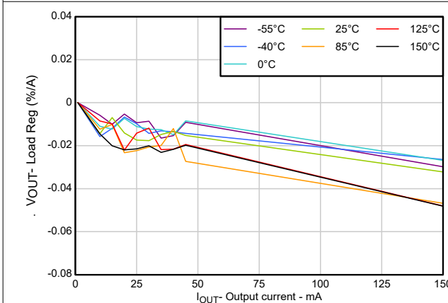
图 5-5. 负载调整率
