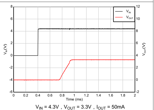
图 5-34. EN 与 V_{IN} 引脚短接启动
