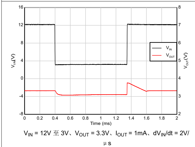
图 5-51. 压降恢复 (12V 至 3V)
