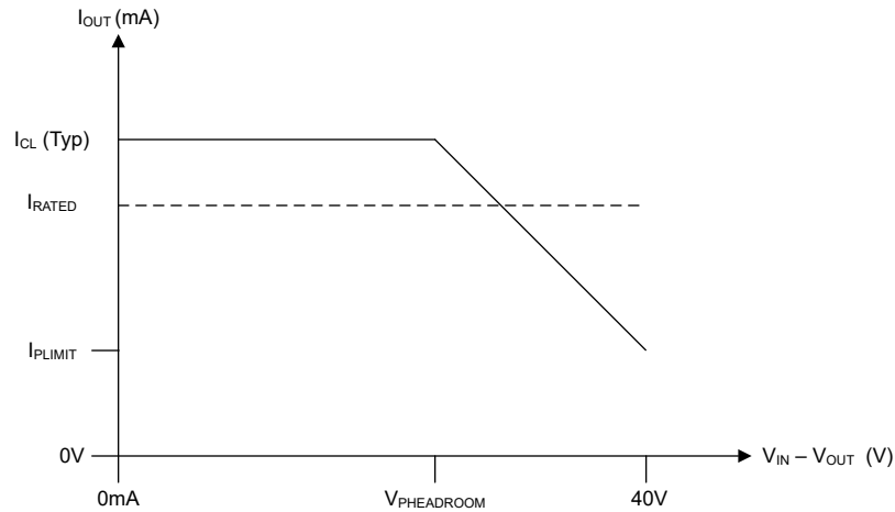
图 6-5. 功率限制
