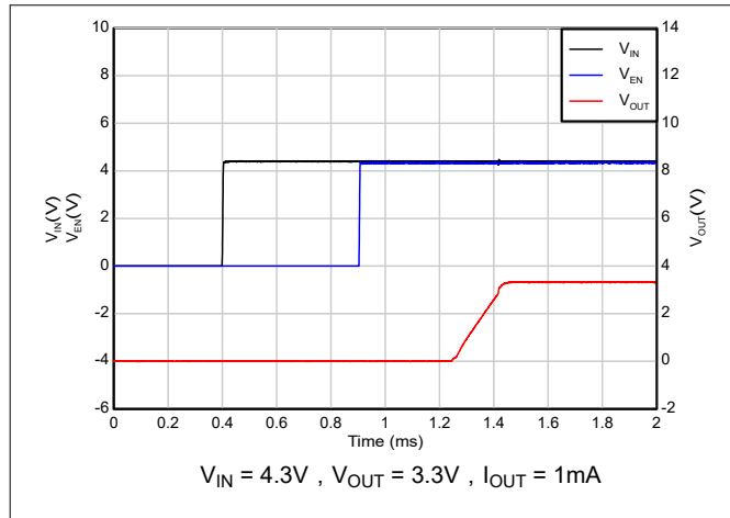
图 5-35. 时序启动 (EN 在 V_{IN} 之后)
