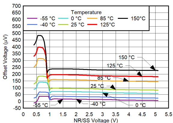
图 6-52. V_{OS} vs V_{NR/SS} and Temperature
