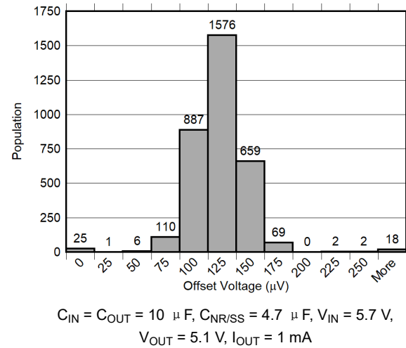
图 6-46. V_{OS} Distribution
