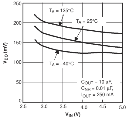
图 6-31. TPS794 压降电压与输入电压间的关系
