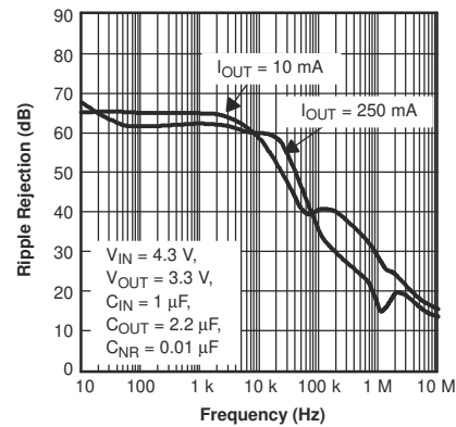
图 6-18. TPS794 波纹抑制与频率
