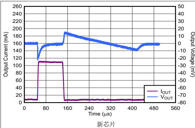
图 5-31. TPS792 负载瞬态响应
