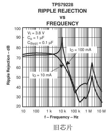
图 5-24. TPS792 波纹抑制与频率
