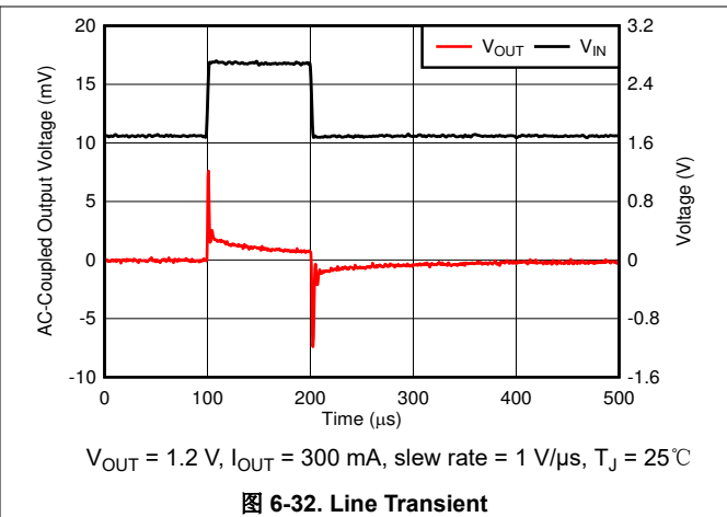
图 6-32. Line Transient
