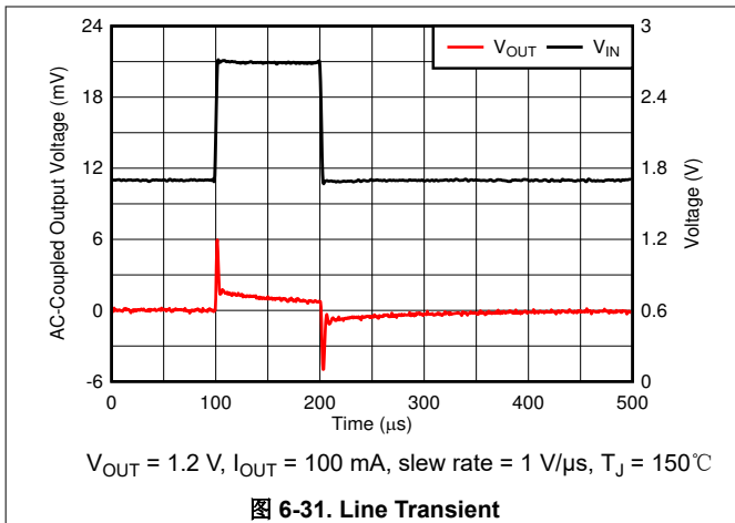
图 6-31. Line Transient
