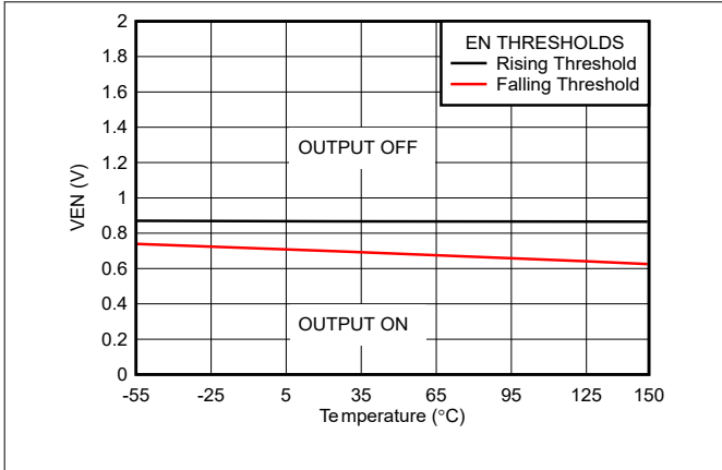
图 5-19. TPS76933 EN 阈值与自然通风温度间的关系 (新芯片)
