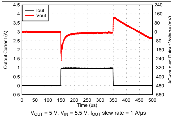
图 27. 1-mA to 1-A Load Transient (5 V)
