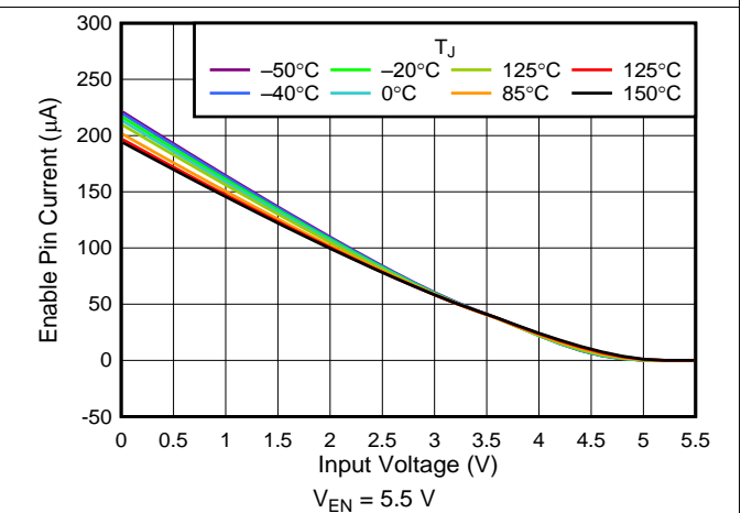
图 22. I_{EN} vs V_{IN}
