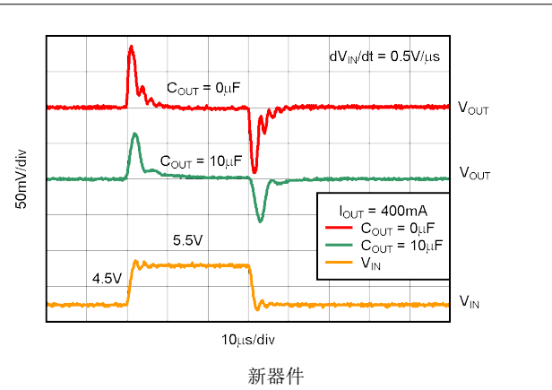
图 5-38. TPS73633 线路瞬态响应
