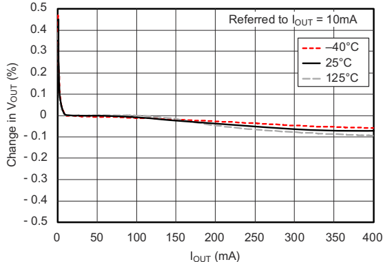
图 5-1. 负载调整率
