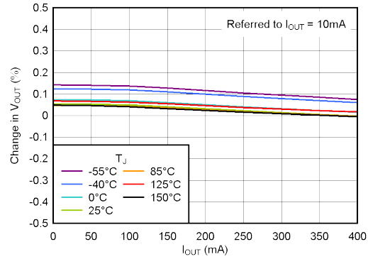
图 5-2. 负载调整率
