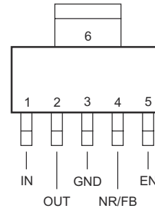
图 4-2. DCQ 封装，6 引脚 SOT-223 (顶视图)
