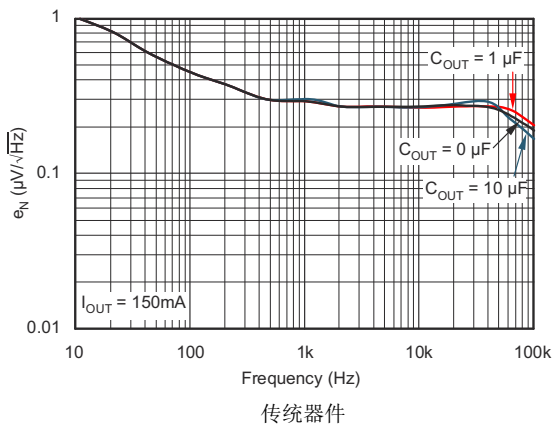
图 5-27. 噪声谱密度 C_{NR} = 0\mu\text{F}
