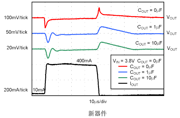
图 7-6. TPS73633 负载瞬态响应
