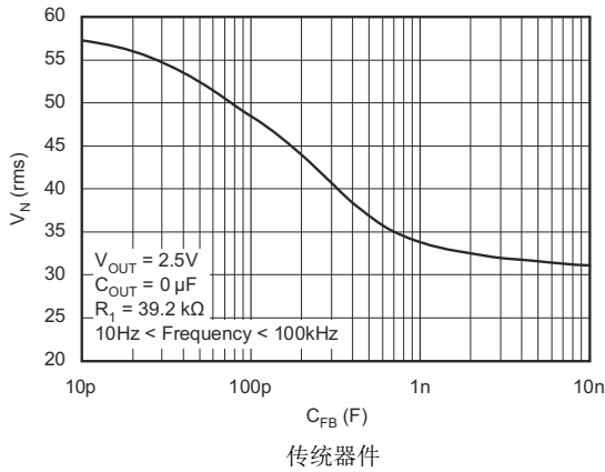
图 7-7. TPS73601 RMS 噪声电压与 C_{FB} 间的关系
