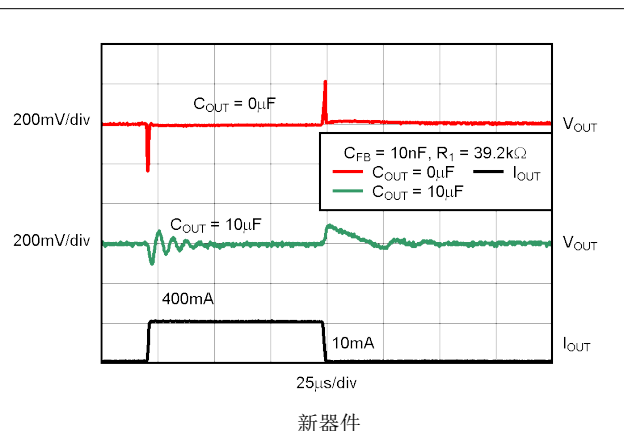
图 7-10. TPS73601 负载瞬态，可调节版本
