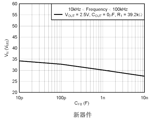
图 7-8. TPS73601 RMS 噪声电压与 C_{FB} 间的关系
