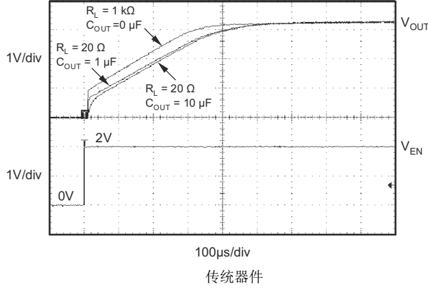
图 7-3. TPS73633 导通响应
