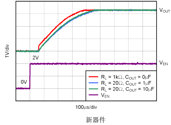
图 7-4. TPS73633 导通响应
