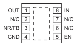
图 4-2. DRB 封装，8 引脚 VSON (俯视图)
