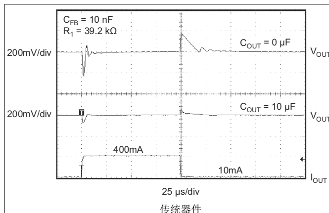
图 7-9. TPS73601 负载瞬态，可调节版本
