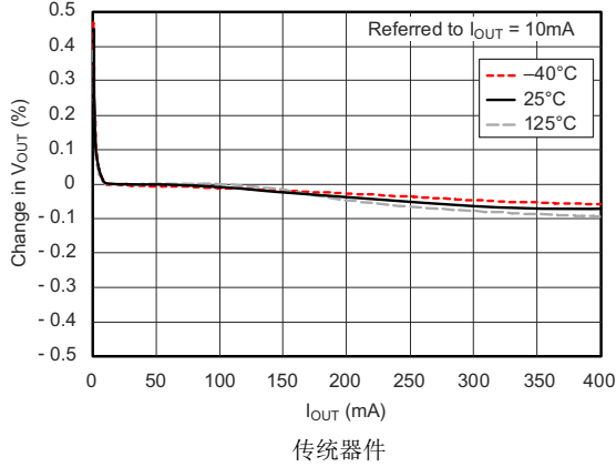
图 5-1. 负载调整率
