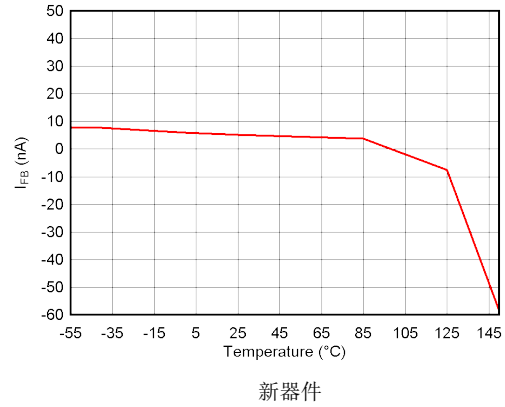
图 5-50. TPS73601 I_{FB} 与温度间的关系
