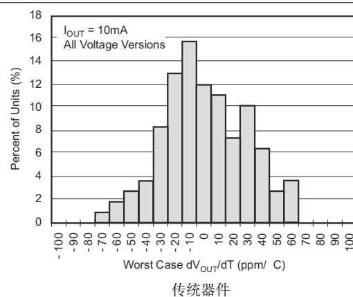
图 5-10. 输出电压漂移柱状图
