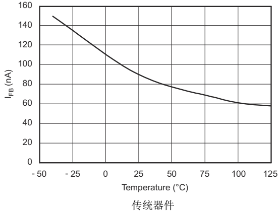
图 5-49. TPS73601 I_{FB} 与温度间的关系
