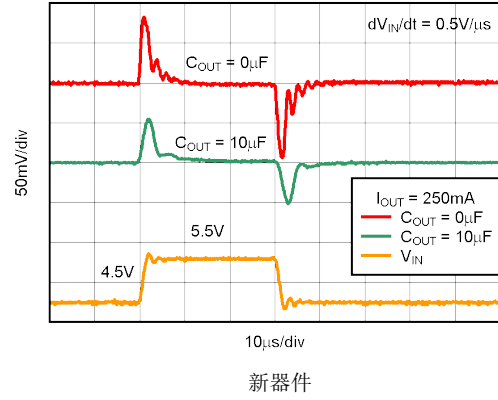
图 5-38. TPS73233-Q1 线路瞬态响应
