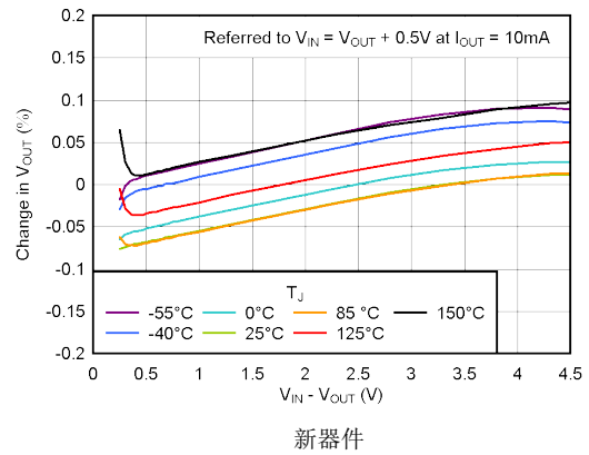
图 5-4. 线路调整
