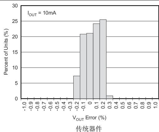
图 5-9. 输出电压精度柱状图
