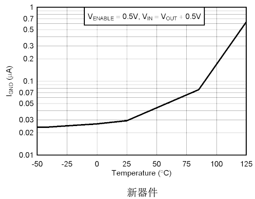
图 5-18. 关断时的接地引脚电流与温度间的关系
