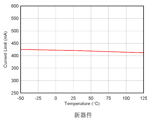
图 5-22. 电流限制与温度间的关系
