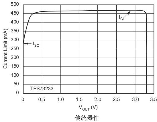
图 5-15. 电流限值与 V_{OUT} (折返) 间的关系
