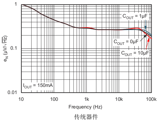
图 5-27. 噪声谱密度与 C_{NR} = 0\mu\text{F} 间的关系
