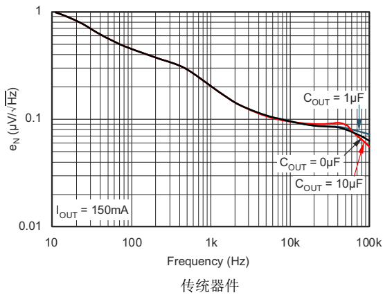
图 5-29. 噪声谱密度与 C_{NR} = 0.01\mu\text{F} 间的关系
