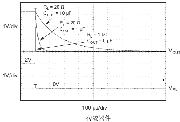
图 5-41. TPS73233-Q1 - 关断响应
