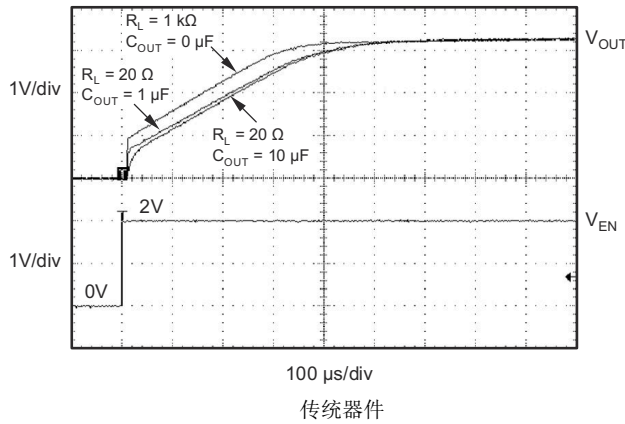
图 5-39. TPS73233-Q1 - 导通响应
