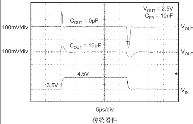
图 5-53. TPS73201-Q1 - 线路瞬态, 可调节版本
