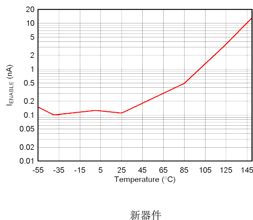
图 5-46. I_{ENABLE} 与温度间的关系
