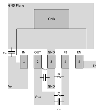
图 7-13. DCQ 封装 (可调节版本) 布局示例
