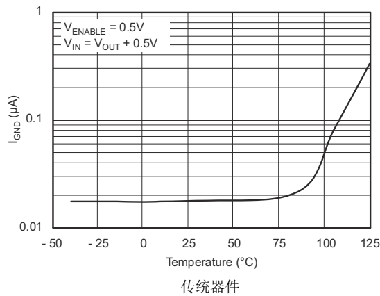
图 5-17. 关断时的接地引脚电流与温度间的关系
