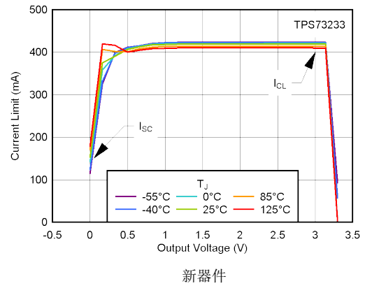
图 5-16. 电流限值与 V_{OUT} (折返) 间的关系
