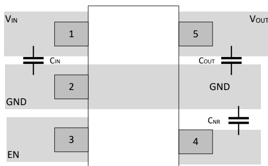
图 7-10. DBV 封装 ( 固定版本 ) 布局示例
