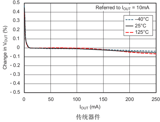
图 5-1. 负载调整率
