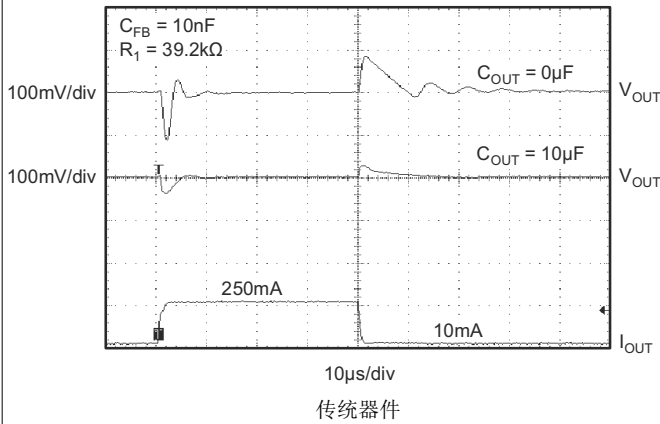
图 5-51. TPS73201-Q1 - 负载瞬态, 可调节版本
