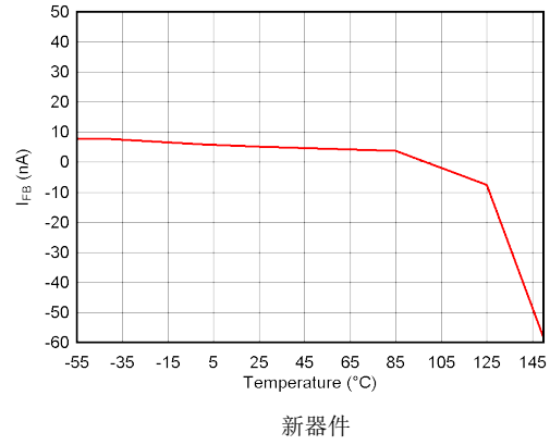
图 5-50. TPS73201-Q1 I_{FB} 与温度间的关系
