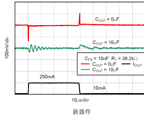
图 5-52. TPS73201-Q1 负载瞬态, 可调节版本
