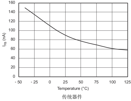
图 5-49. TPS73201-Q1 - I_{FB} 与温度间的关系
