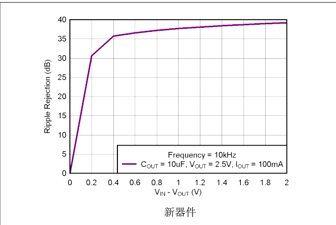
图 5-26. PSRR (纹波抑制) 与 (V_{IN} - V_{OUT}) 间的关系
