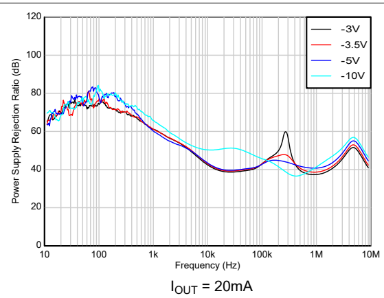
图 5-76. PSRR 与 V_{IN} 间的关系 (新芯片)
