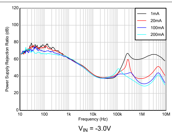
图 5-74. PSRR 与 I_{OUT} 间的关系 (新芯片)
