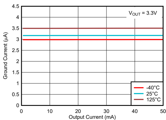
TPS715-Q1 的静态电流与负载电流之间的关系（仅限新芯片）
