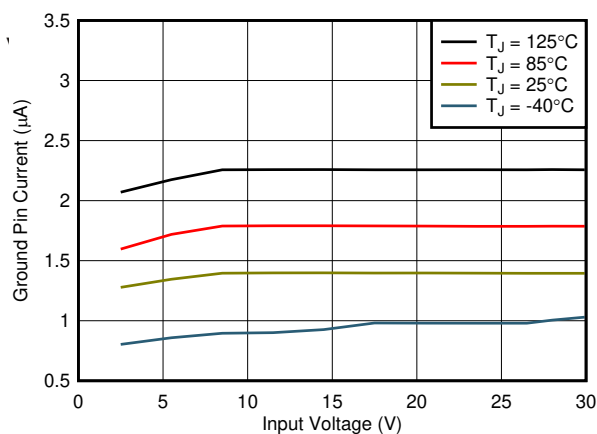
接地电流与 V_{IN} 和温度间的关系
