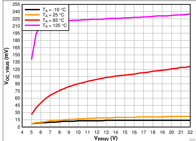
图 5. V_{OC\_VBUS} , VBUS Open Circuit Voltage versus PPHV
