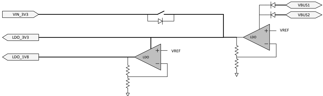
图 8-9. Power Supplies
