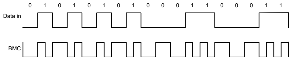
图 8-4. Biphas Mark Coding Example
