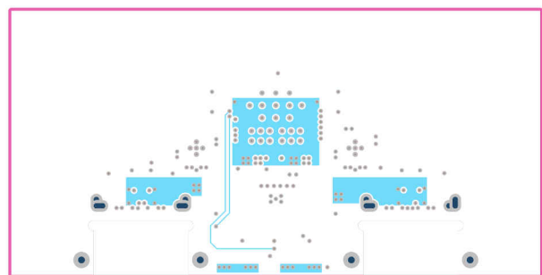
图 11-23. Power 1 Layer
