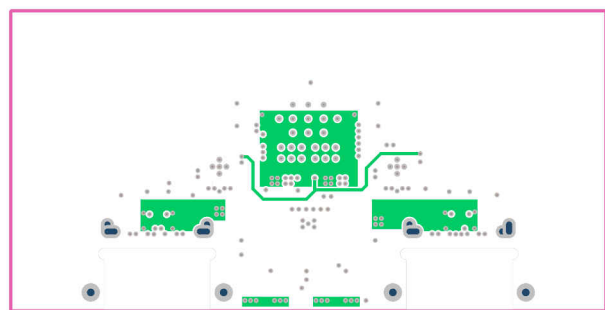
图 11-24. Power 2 Layer
