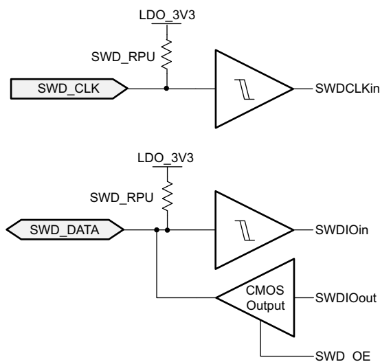
图 8-15. IOBUF_GPIOHSSWD
