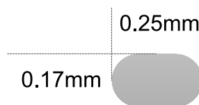
图 11-6. Oval Pad Sizing
