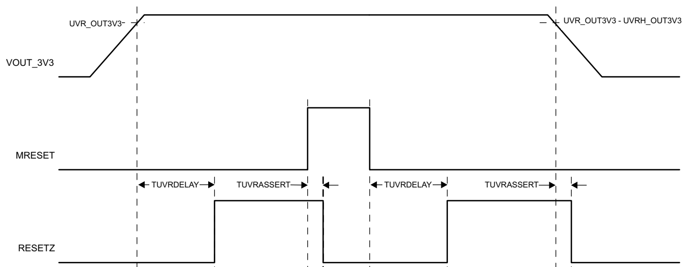
图 7-1. RESETZ Assertion Timing
