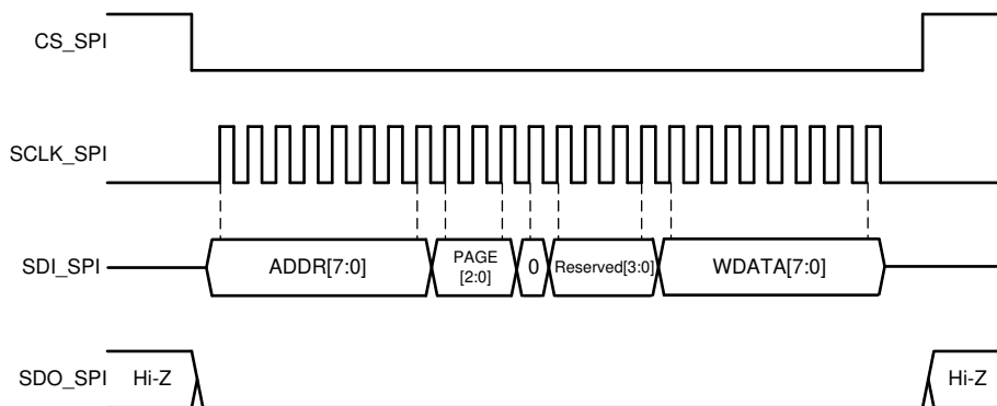
图 8-61. SPI Write Cycle
