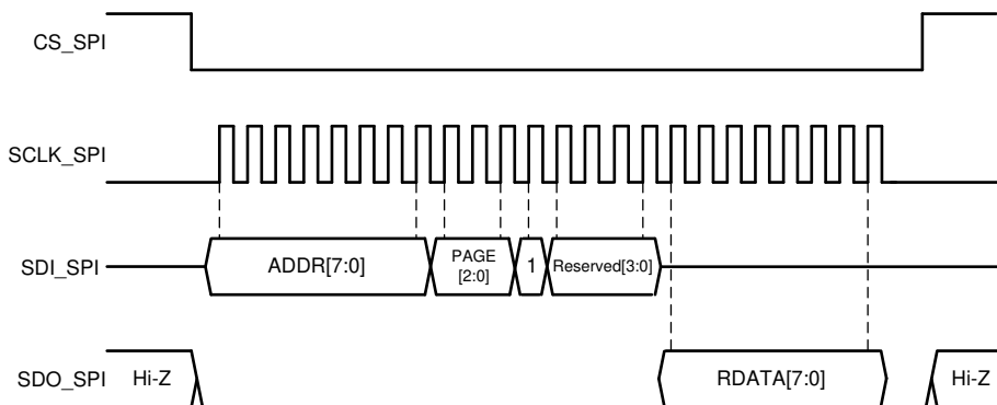
图 8-63. SPI Read Cycle
