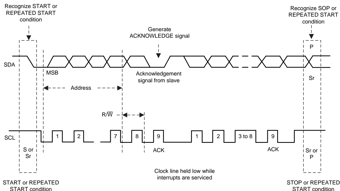
图 5-20. Bus Protocol
