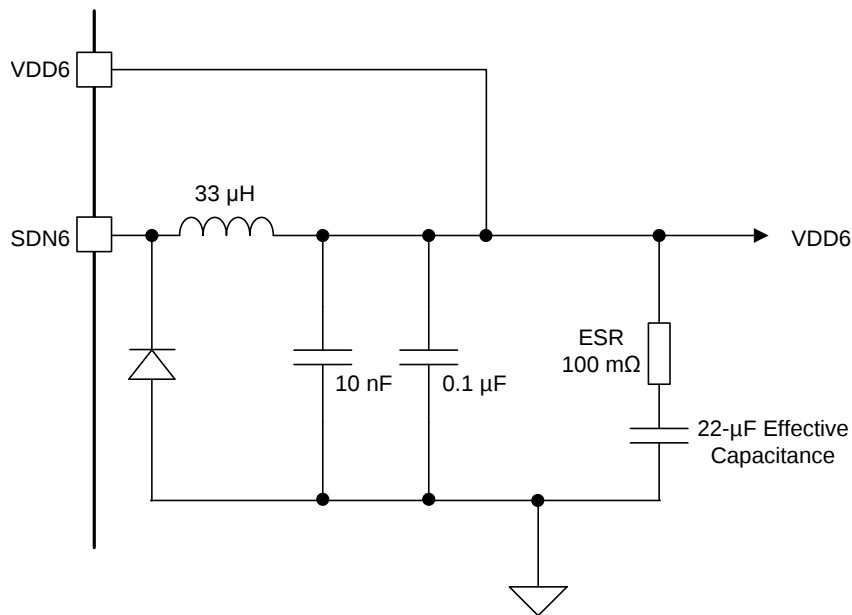
Figure 6-2. VDD6 设计
