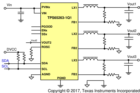
应用原理图
