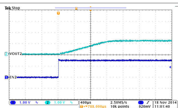
图 8-4. BUCK2, Soft Start
