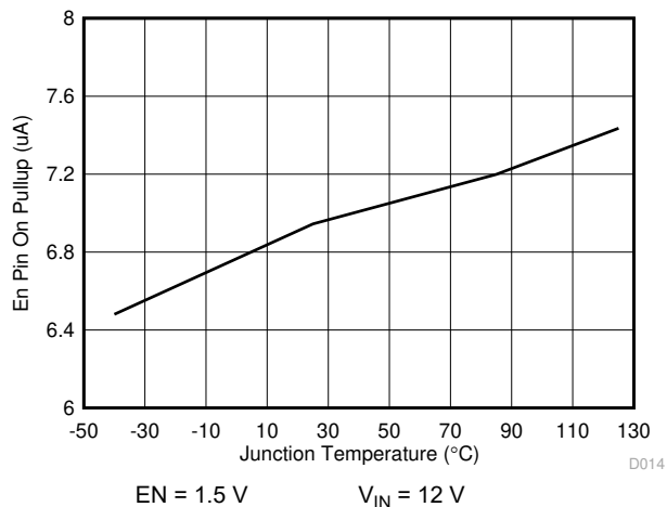
图 6-14. EN Pin Pullup Current vs Temperature, EN = 1.5 V
