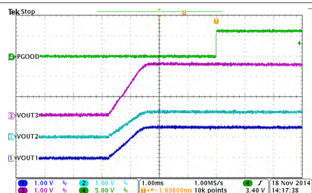
图 8-18. PGOOD
