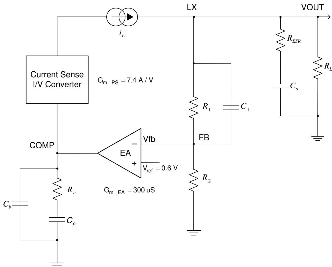
图 8-2. DC/DC Loop Compensation
