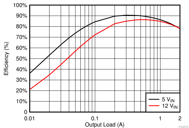
图 6-2. BUCK2 Efficiency
