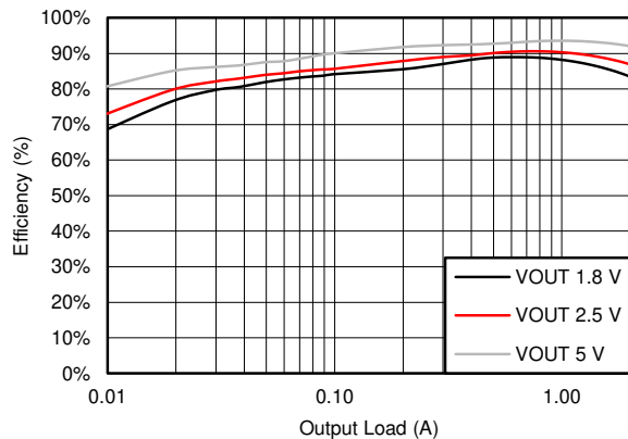
图 7-3. BUCK3 Efficiency
