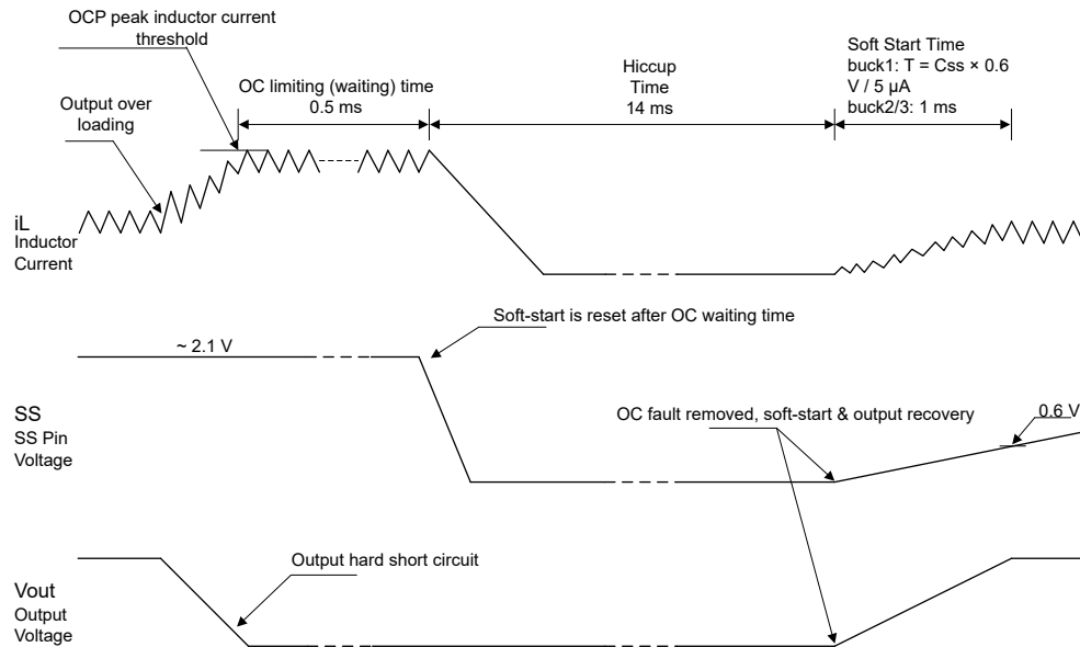
图 7-6. Overcurrent Protection
