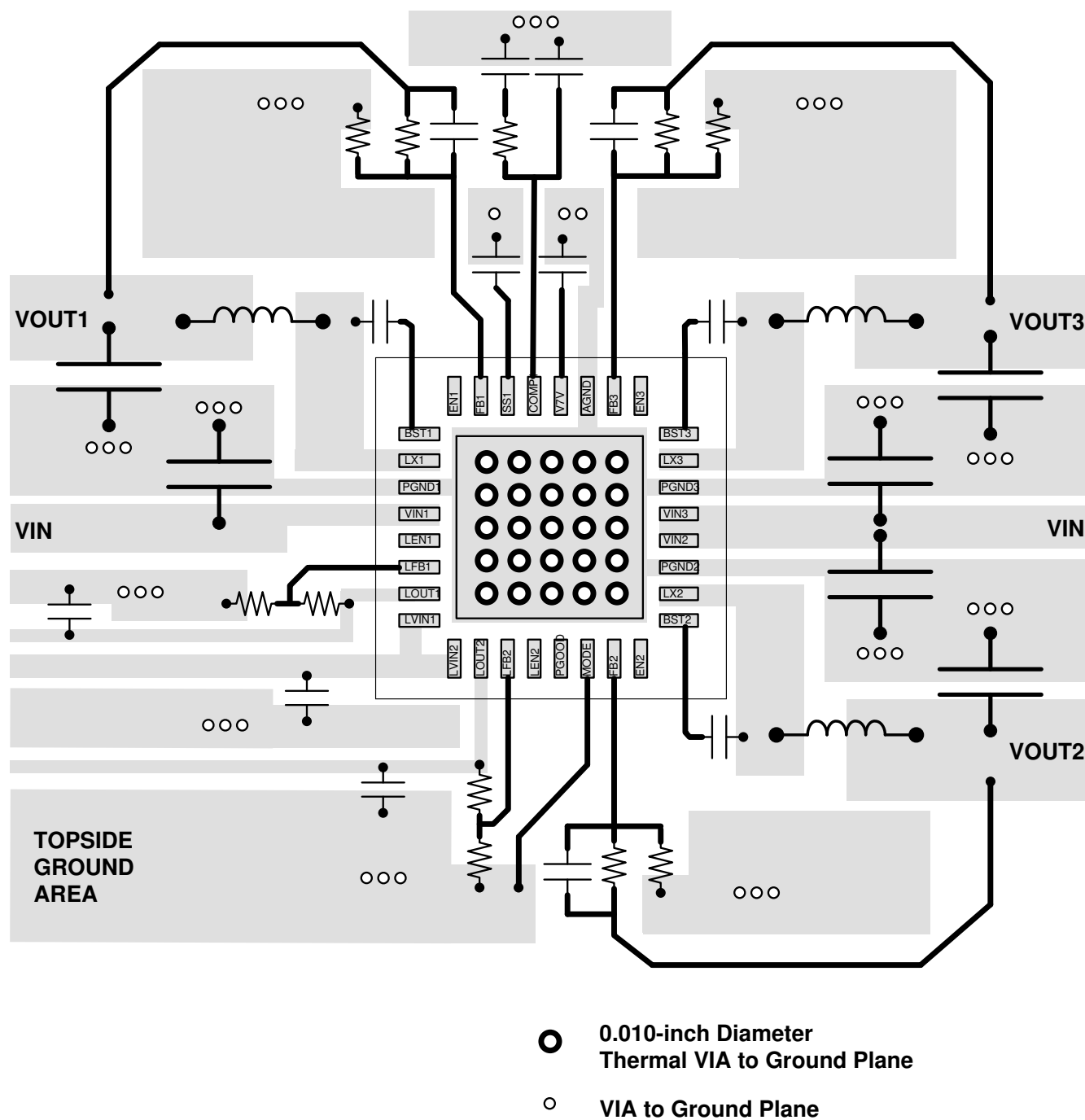
图 8-37. PCB Layout
