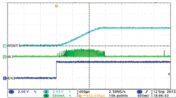
图 8-7. PSM Mode Buck3, Soft-Start With No Load
