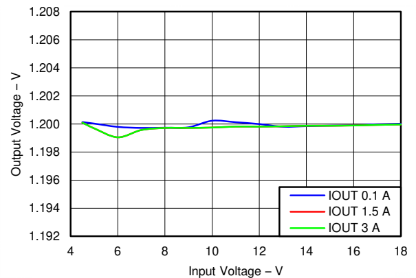
图 6-6. Buck1, PSM Mode Line Regulation
