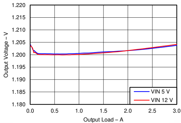
图 6-3. Buck1, PSM Mode Load Regulation
