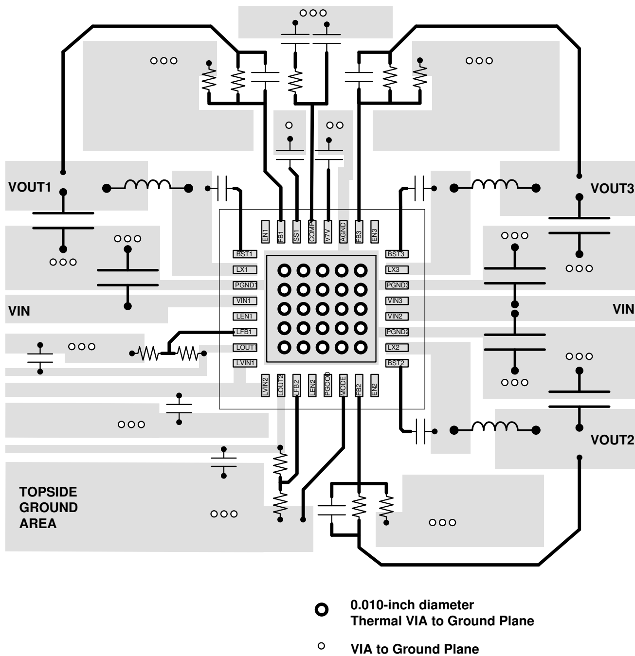
图 9-34. PCB Layout
