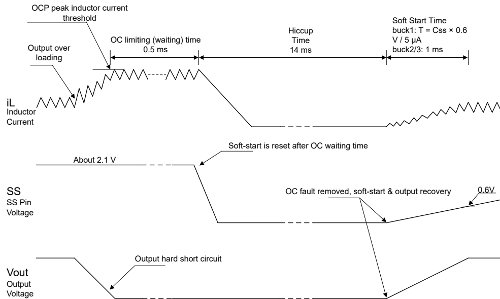
图 8-7. OCP
