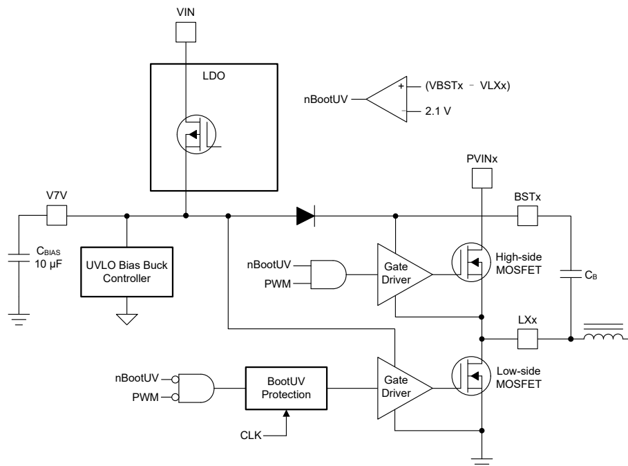
图 8-5. V7V 线性 Dropout 调节器和 Bootstrap 电压图
