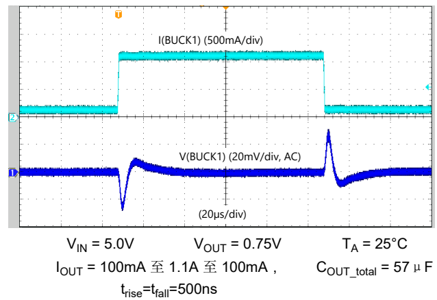
图 5-4. BUCK1 负载阶跃响应 - 高带宽, 强制 PWM
