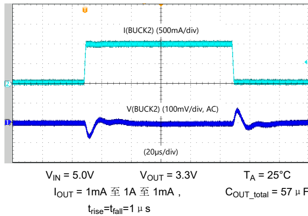
图 5-5. BUCK2 负载阶跃响应 - 低带宽, 强制 PWM
