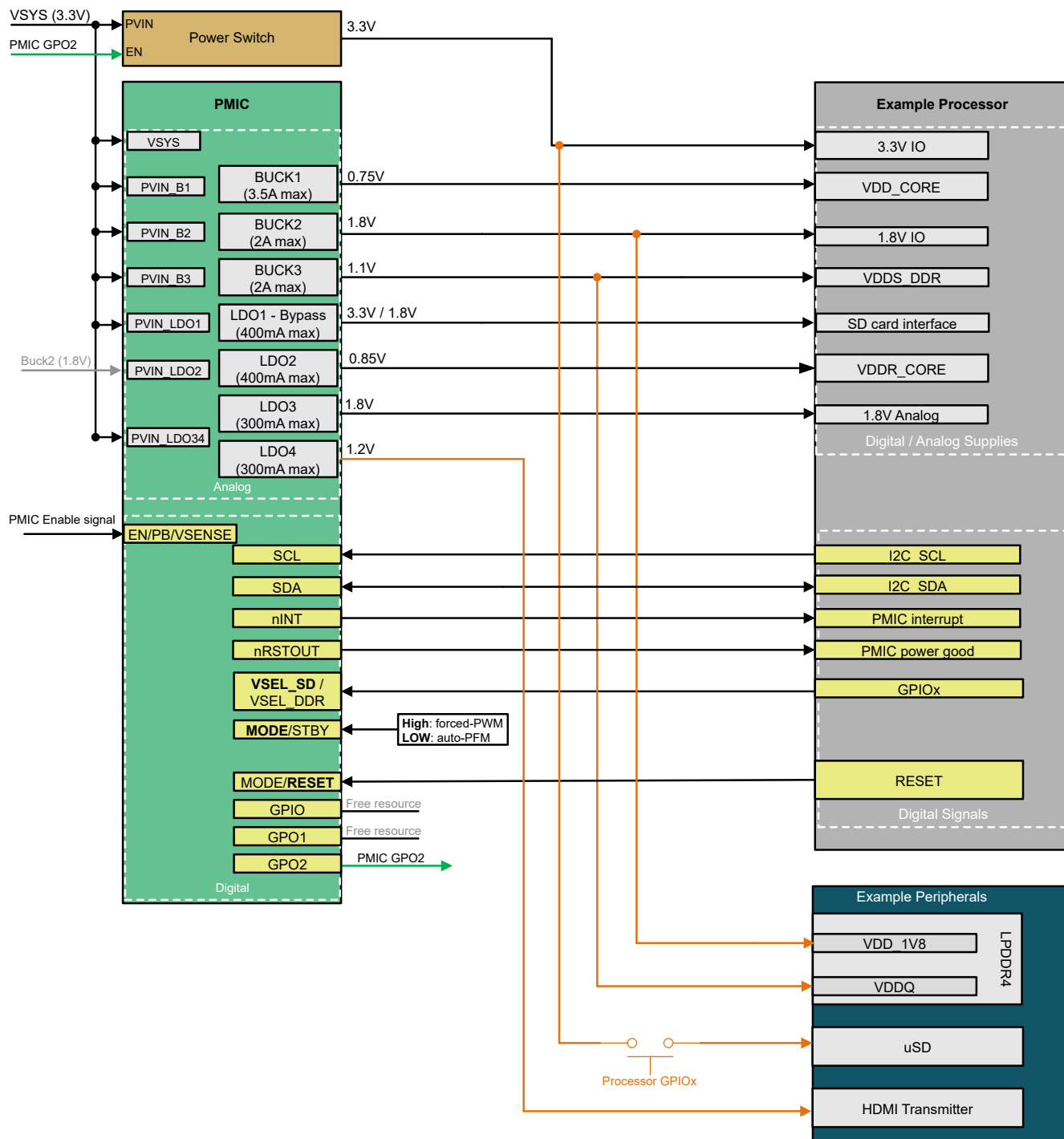
图 7-1. 示例电源图
