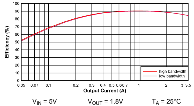
图 5-2. BUCK1 效率
