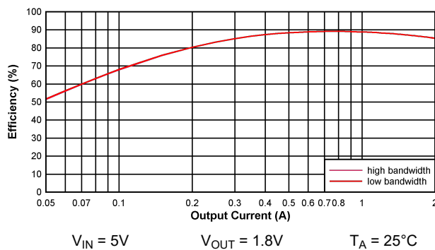
图 5-3. BUCK23 效率
