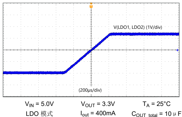
图 7-5. LDO1 斜坡
