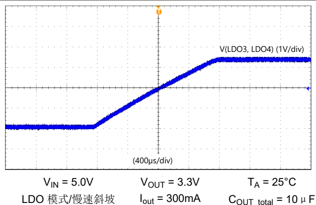
图 7-7. LDO 慢速斜坡
