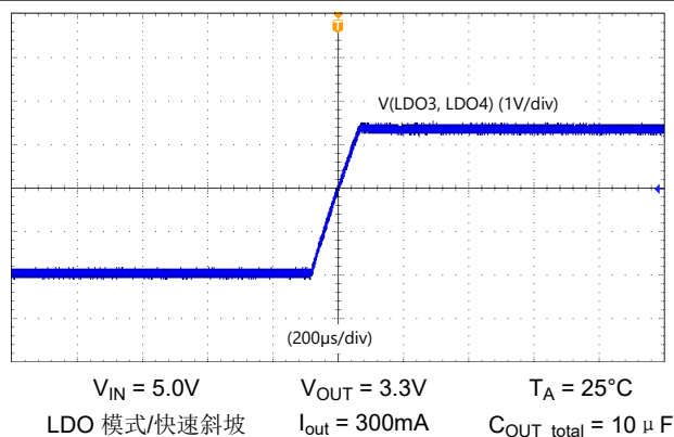
图 7-6. LDO 快速斜坡
