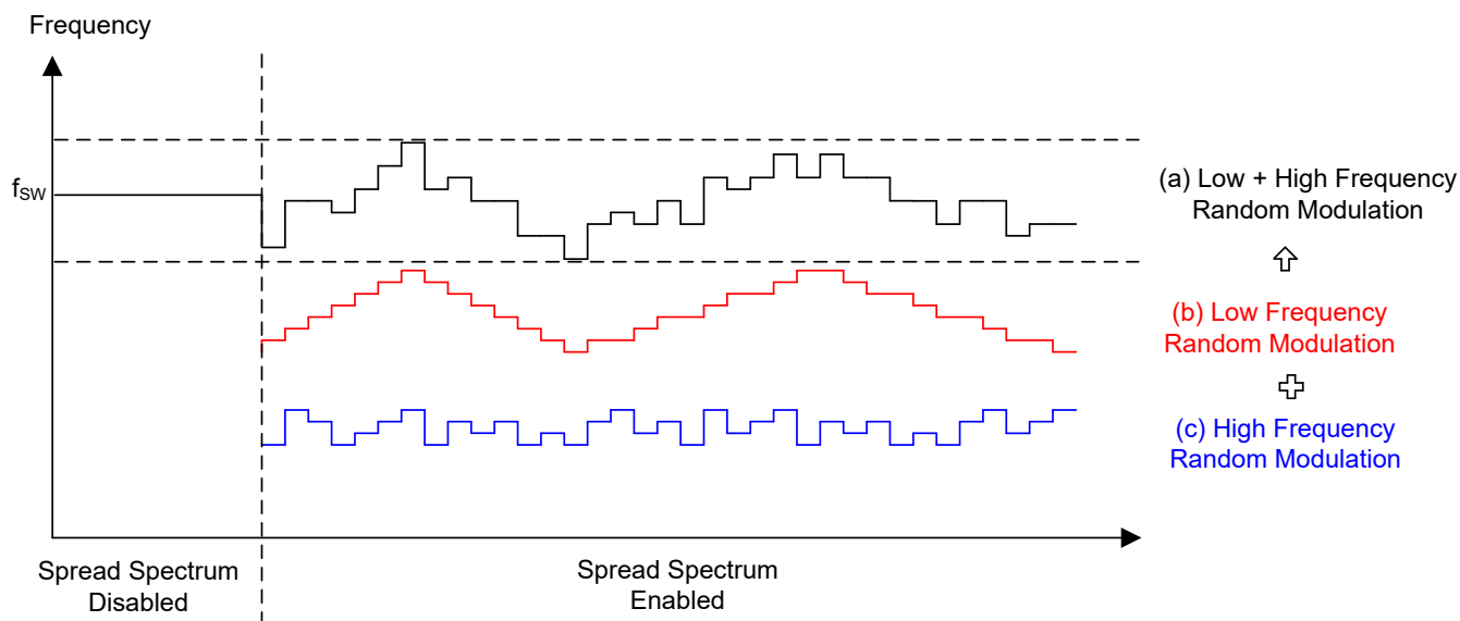
图 6-4. 双随机展频
