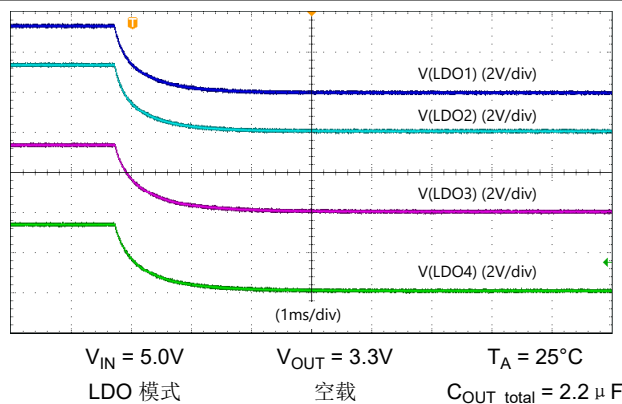
图 7-9. LDO 放电
