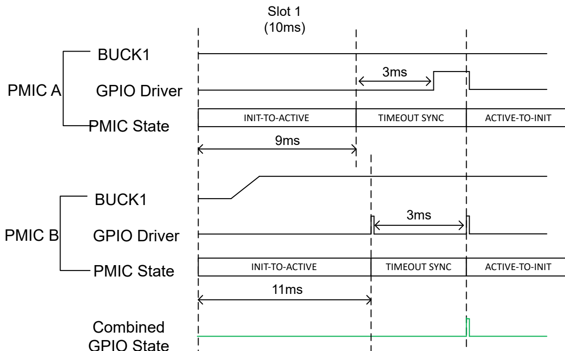
图 6-17. 超时同步
