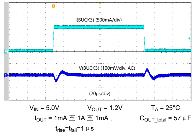
图 5-6. BUCK3 负载阶跃响应 - 低带宽, 强制 PWM
