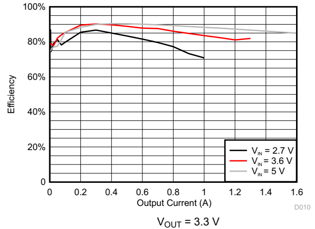
图 8-6. DCDC4 Efficiency
