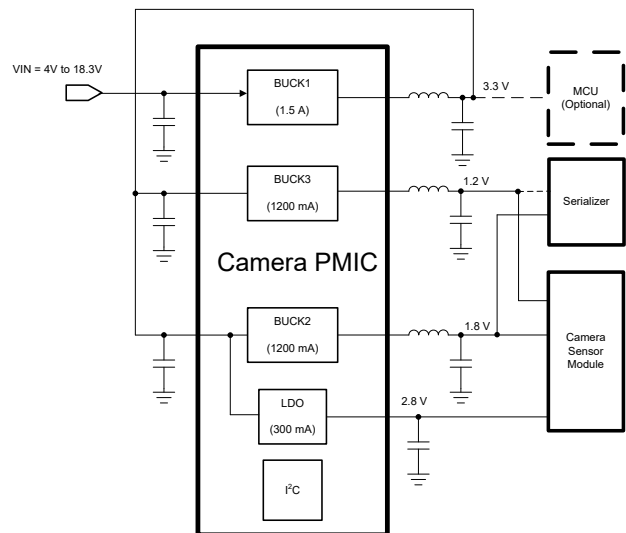
TPS650350-Q1 应用电路
