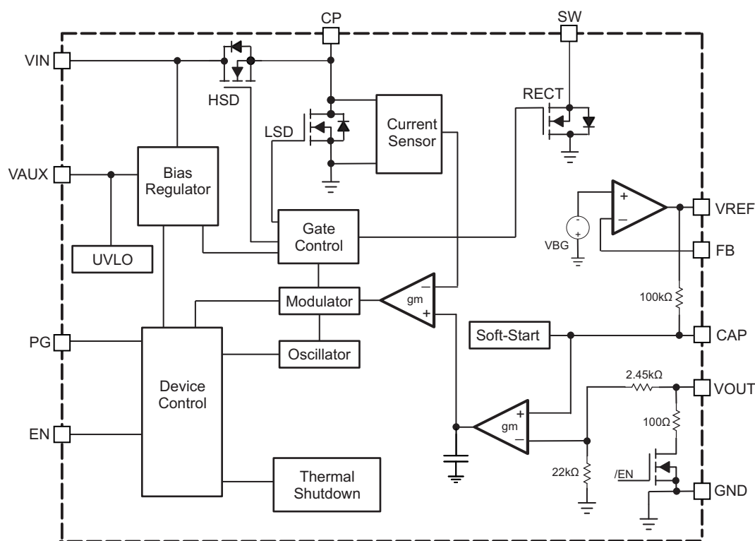
图 8. Block Diagram
