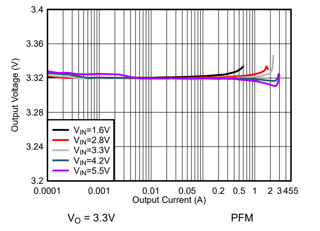
图 9-5. 负载调节 (PFM)
