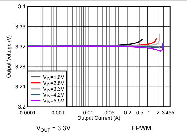
图 9-3. 负载调节 (FPWM)
