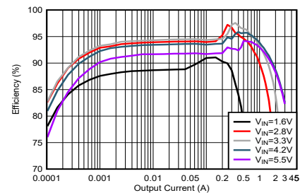
效率与输出电流间的关系 ( V_{OUT} = 3.3V )
