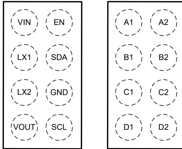
图 5-1. TPS631013A YBG 封装，8 引脚 WCSP (顶视图)
