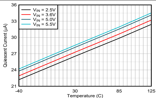
图 6-2. 静态电流与结温间的关系
