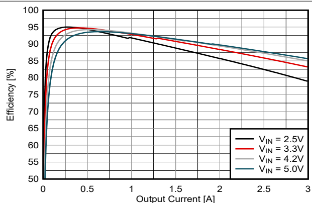
图 8-7. 1.2V 输出效率 (TPS62A03A)
