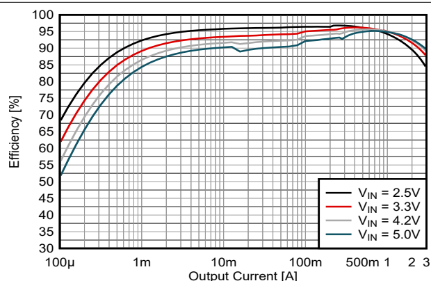
图 8-4. 1.8V 输出效率 (TPS62A03)
