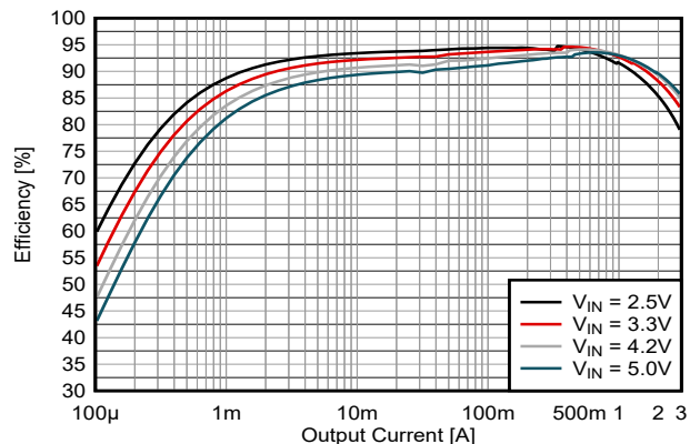
图 8-3. 1.2V 输出效率 (TPS62A03)
