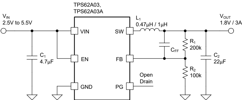
图 8-1. TPS62A03 典型应用电路
