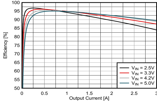
图 8-8. 1.8V 输出效率 (TPS62A03A)
