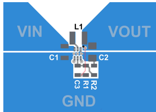
图 8-10. TPS62A0x PCB 布局建议
