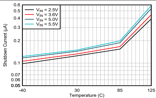
图 6-4. 关断电流与结温间的关系
