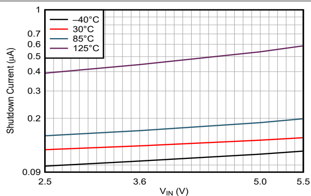
图 6-3. 关断电流与输入电压间的关系
