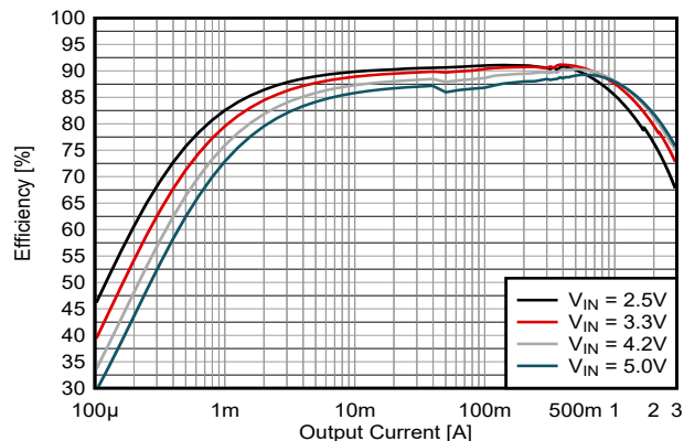
图 8-2. 0.6V 输出效率 (TPS62A03)
