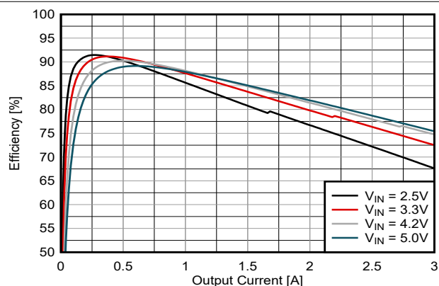
图 8-6. 0.6V 输出效率 (TPS62A03A)
