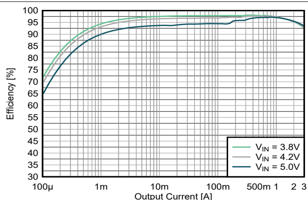
图 8-5. 3.3V 输出效率 (TPS62A03)
