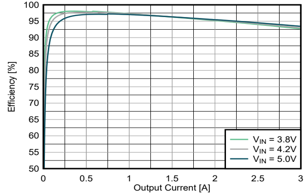
图 8-9. 3.3V 输出效率 (TPS62A03A)
