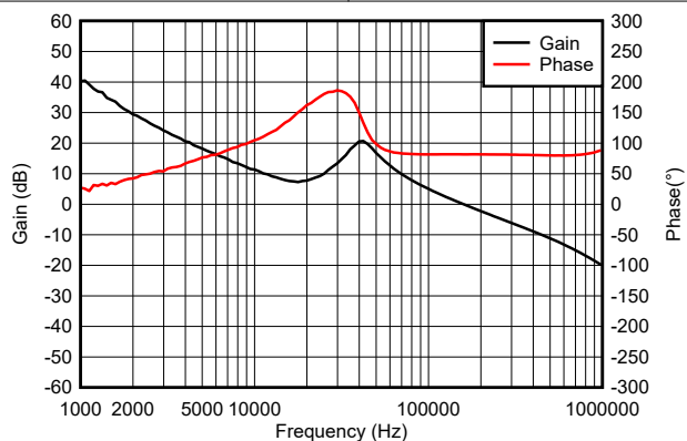
图 9-79. Input Voltage Ripple
