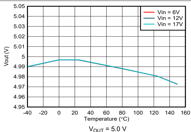
图 7-4. Output Voltage Accuracy - VSET Selected
