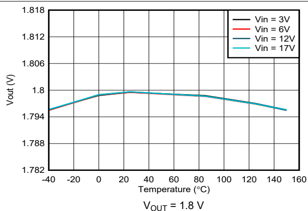
图 7-6. Output Voltage Accuracy - VSET Selected
