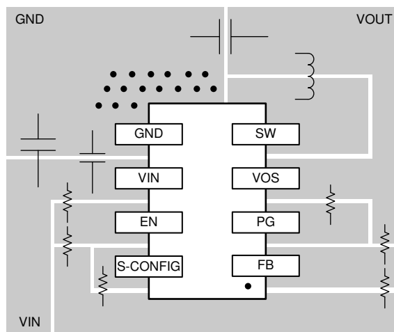
图 9-86. TPS629210-Q1 Layout
