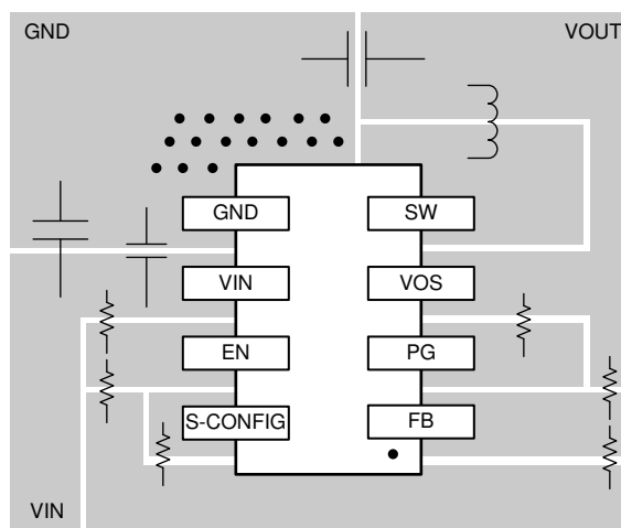
图 11-1. TPS629206 Layout
