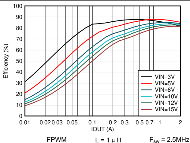
图 8-22. 效率与输出电流间的关系 V_{OUT} = 1.2V
