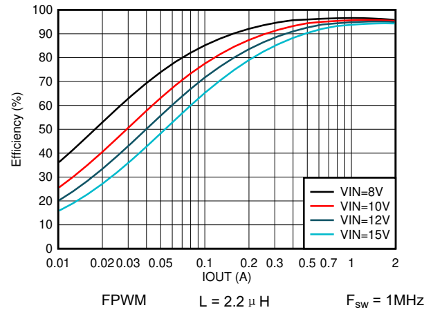
图 8-8. 效率与输出电流间的关系 V_{OUT} = 5V
