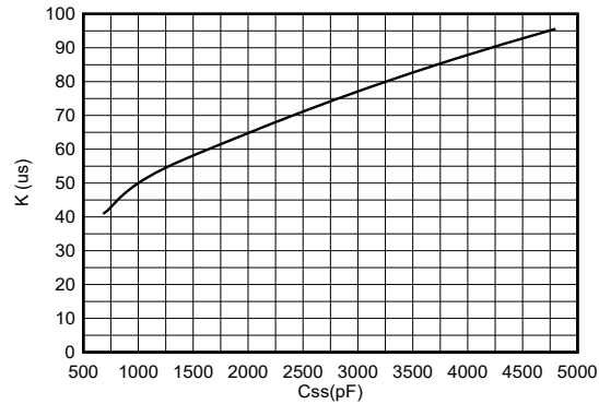
图 8-3. K 与 C_{SS} 关系曲线 (680pF-4800pF)
