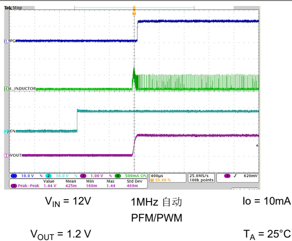
图 8-41. 启动时序
