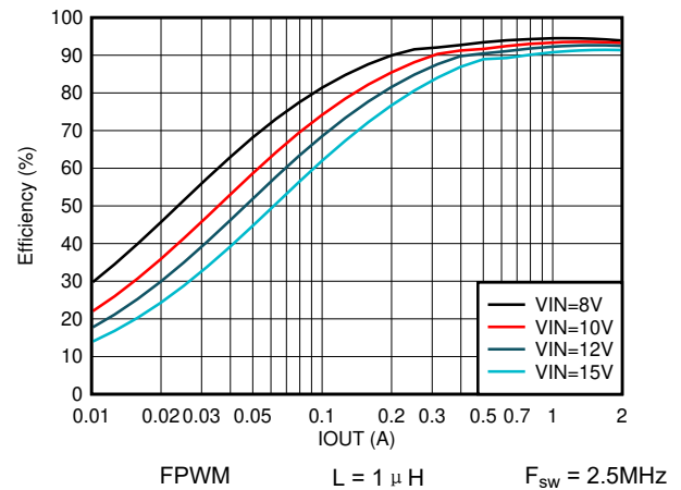
图 8-10. 效率与输出电流间的关系 V_{OUT} = 5V
