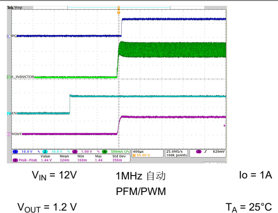
图 8-42. 启动时序
