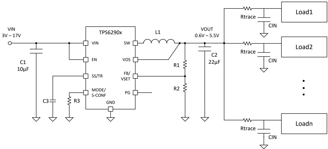
图 8-83. 多个负载
