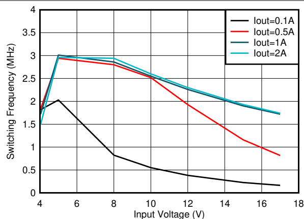
图 8-27. 开关频率与输入电压间的关系 V_{OUT} = 3.3V
