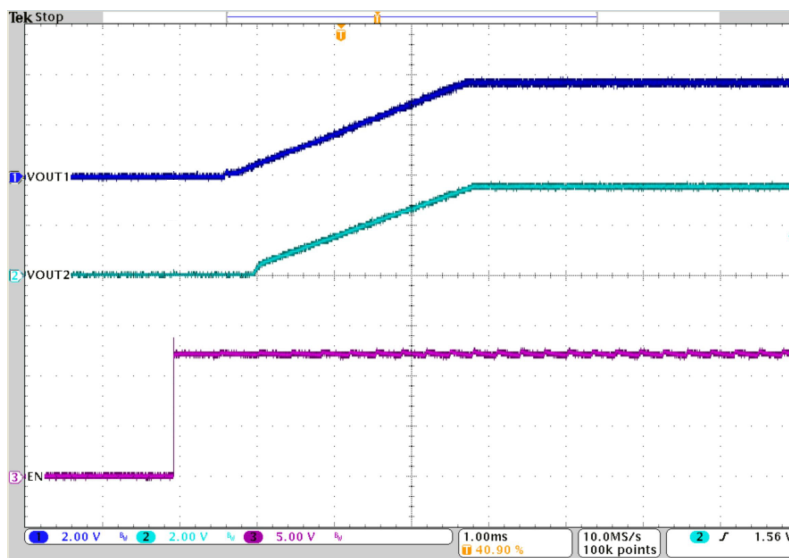
图 8-85. 跟踪
