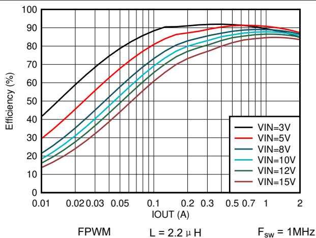
图 8-20. 效率与输出电流间的关系 V_{OUT} = 1.2V
