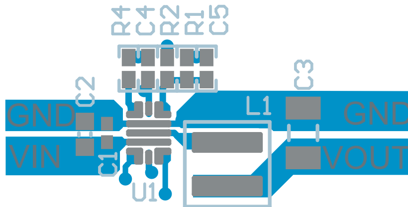
图 12-1. Layout Example
