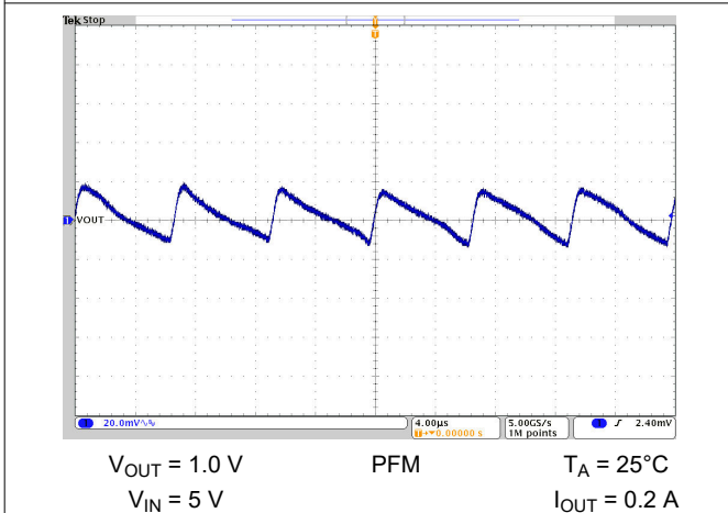
图 10-48. Output Voltage Ripple
