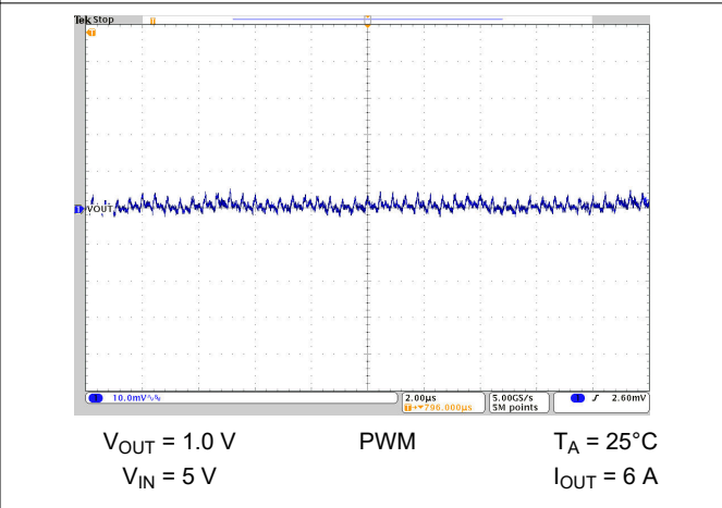
图 10-49. Output Voltage Ripple
