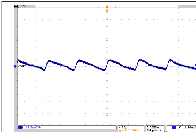
图 10-50. Output Voltage Ripple
