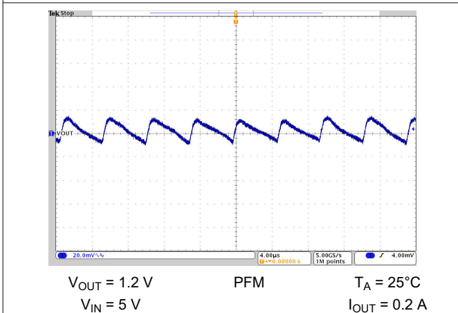
图 10-46. Output Voltage Ripple
