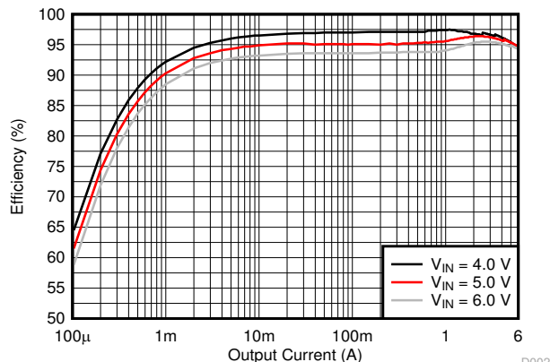
效率与输出电流间的关系； V OUT = 3.3V ; PWM/PFM ; f s = 2.25MHz
