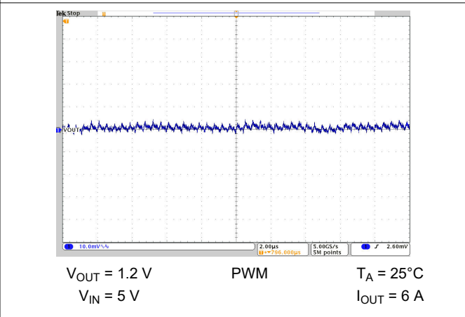
图 10-47. Output Voltage Ripple
