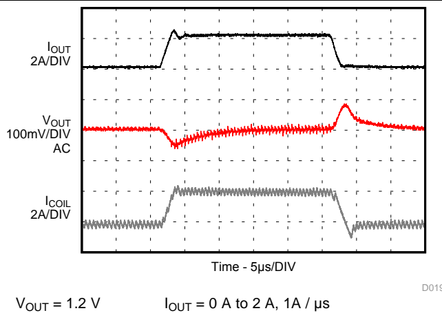
图 21. Load Transient, Forced PWM Mode (2.0MHz)
