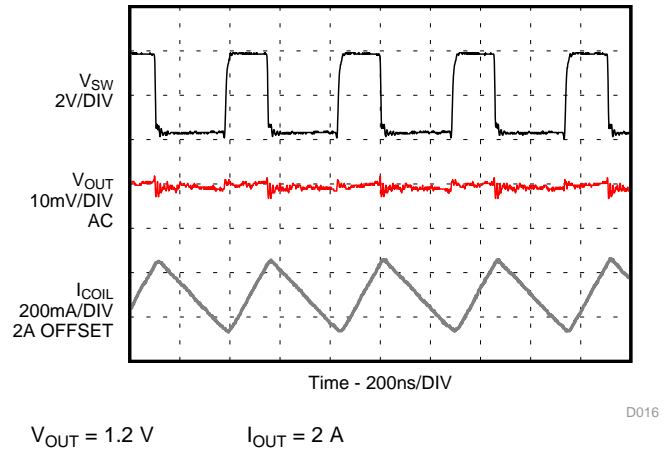
图 18. Output Ripple, PWM Operation (2.0MHz)
