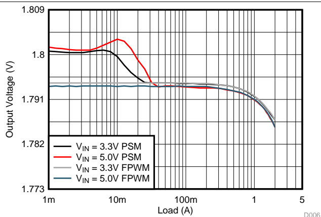
图 13. Load Regulation
