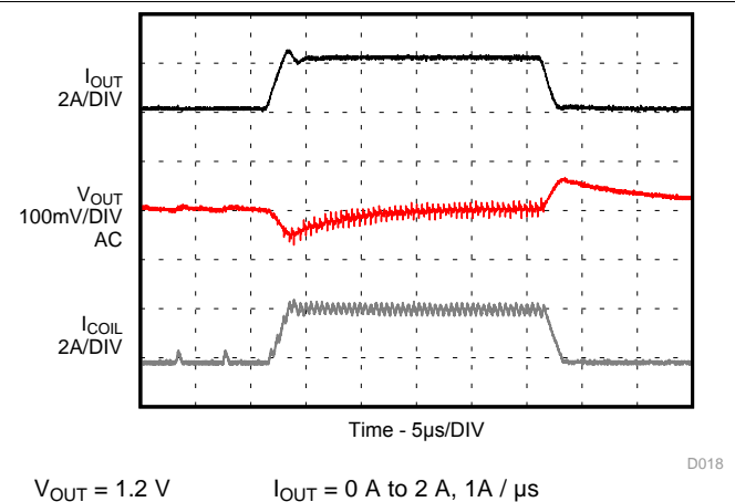
图 20. Load Transient, PWM/PSM Mode (2.0MHz)
