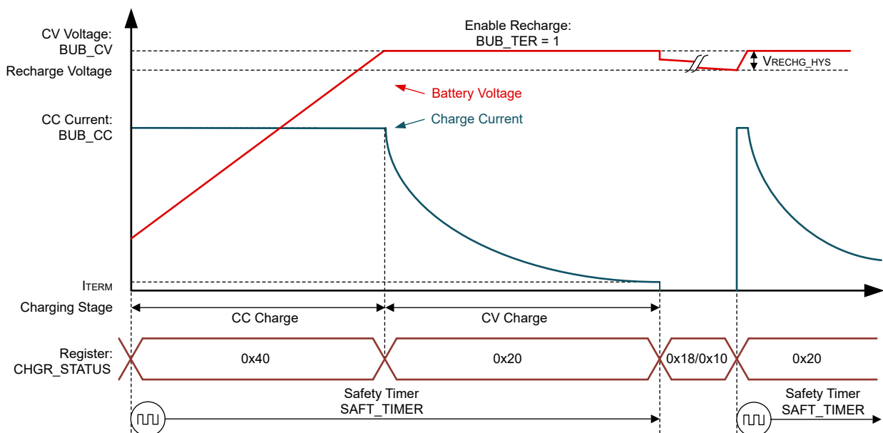
图 6-10. 超级电容器充电曲线，已启用重新充电
