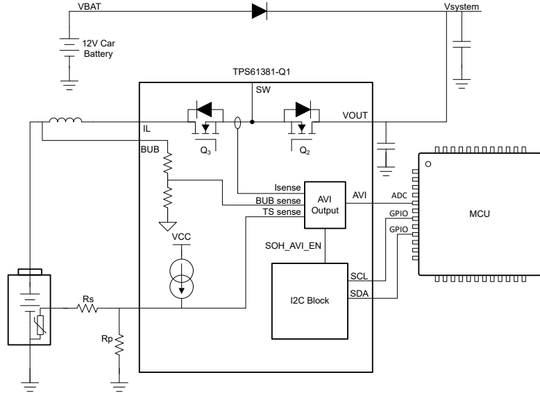
图 6-18. AVI 引脚连接
