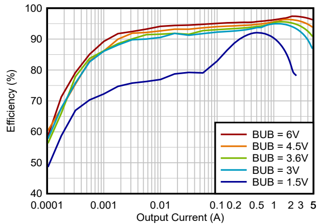
图 5-3. 升压效率与输出电流间的关系, V_{OUT} = 8V , PFM
