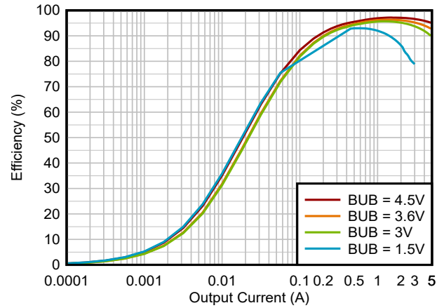
图 5-2. 升压效率与输出电流间的关系, V_{OUT} = 6.2V , FPWM
