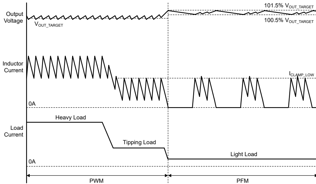
图 6-15. PWM 和 PFM 运行
