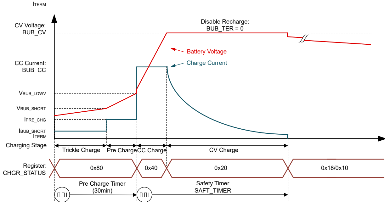
图 6-7. 禁用重新充电功能时的锂基电池充电曲线
