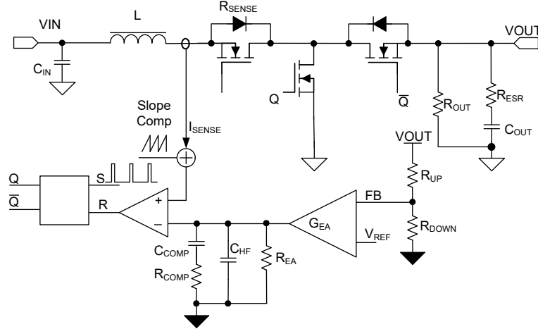
图 8-3. TPS61381-Q1 控制等效电路模型
