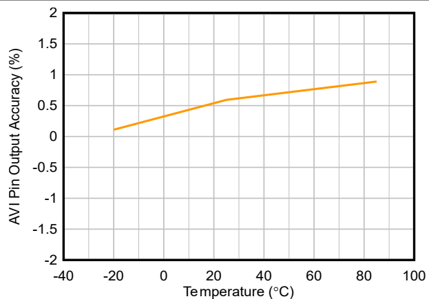
图 5-20. AVI 引脚放电电流输出精度与温度间的关系, I_{\text{discharge}} = 500\text{mA} , 比率 = 2
