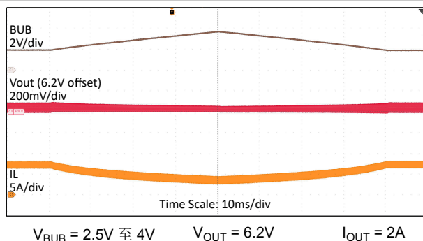
图 8-10. 升压模式下的线路扫描
