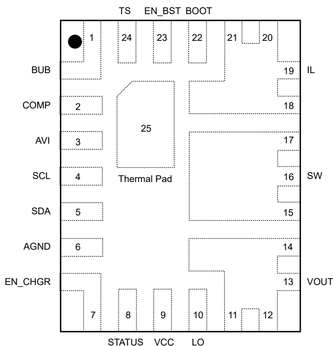
图 4-1. 可焊侧翼具有的 24 引脚 QFN 封装（顶视图）
