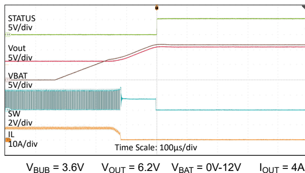
图 8-16. 切换到待机模式 (12V 电池恢复)
