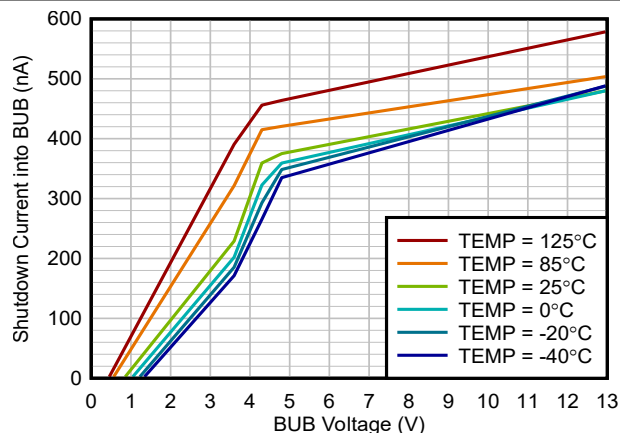
图 5-14. 流入 BUB 的关断电流与 BUB 电压间的关系, V_{OUT} = 12V
