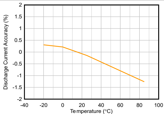
图 5-19. 放电电流精度与温度间的关系, I_{\text{discharge}} = 500\text{mA}
