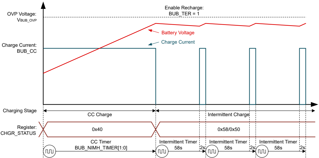
图 6-6. 启用重新充电功能时的镍氢电池充电曲线
