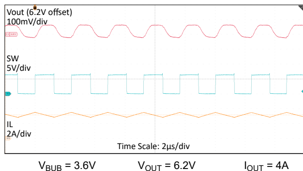
图 8-5. 重负载状态下的升压开关
