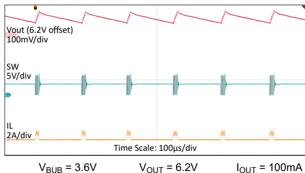
图 8-6. 轻负载状态下的升压开关
