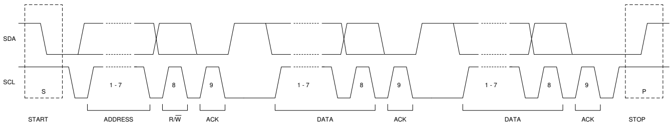
图 6-22. 从机地址和数据方向
