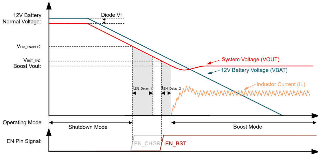
图 6-14. 手动切换到升压模式
