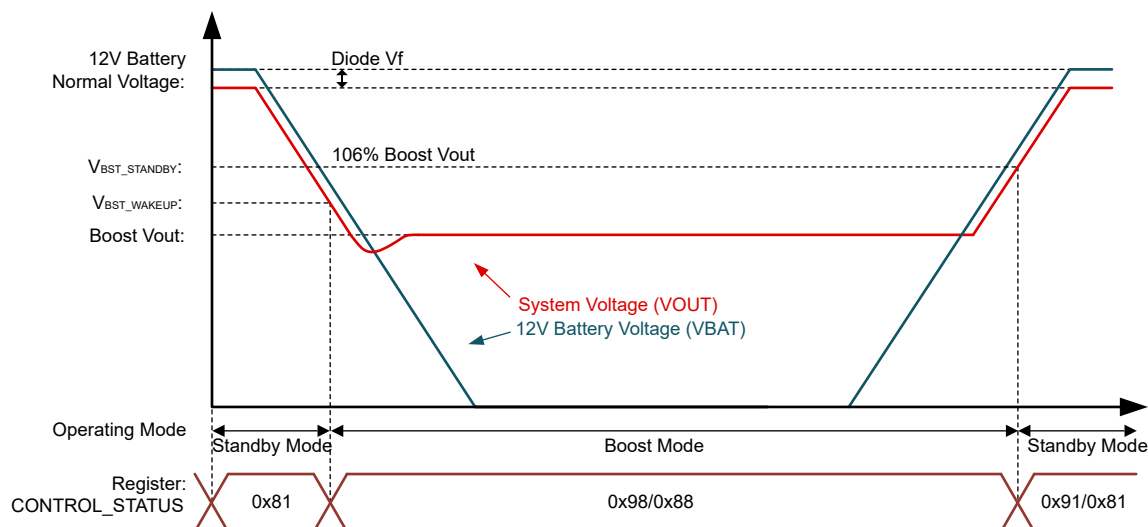
图 6-12. 案例 1： V_{\text{BST\_WAKEUP}} > \text{BST\_VOUT}
