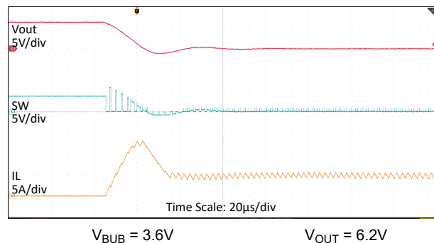
图 8-11. 升压输出短路保护
