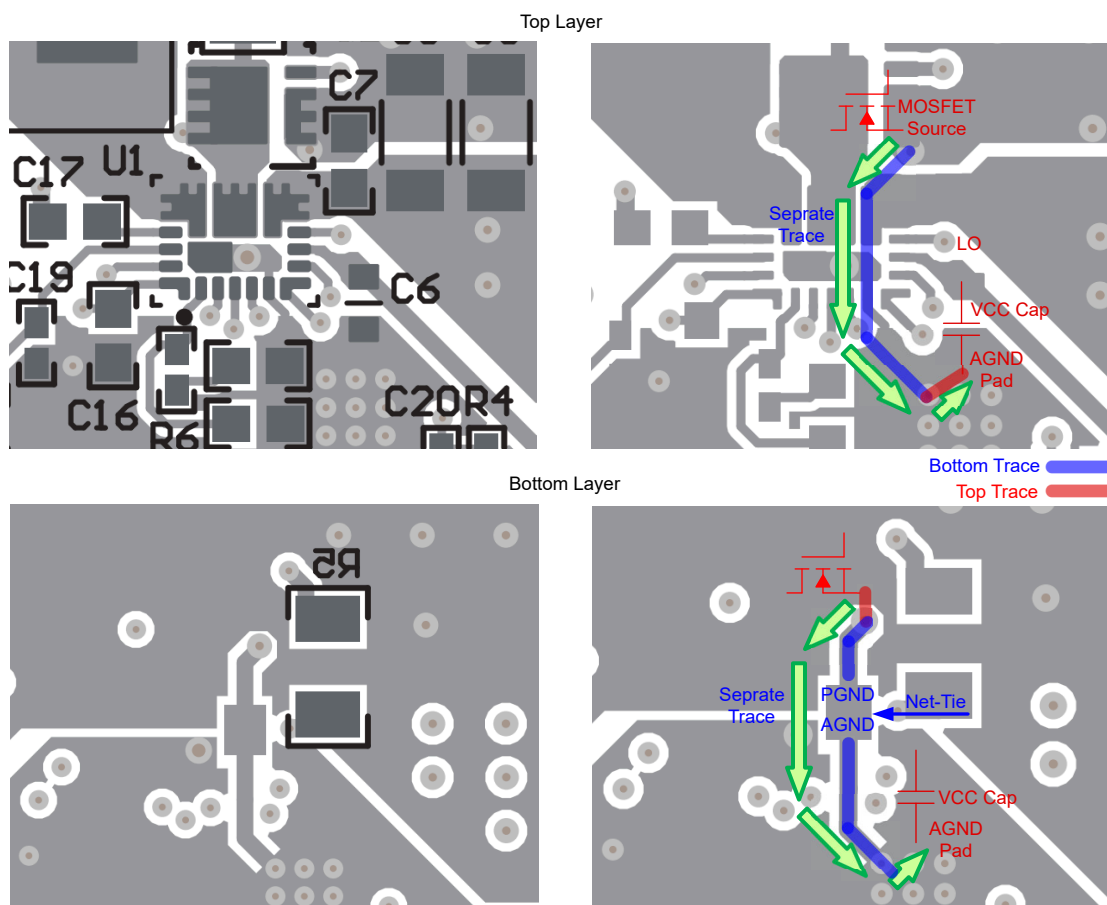
图 8-23. GND 连接布局示例
