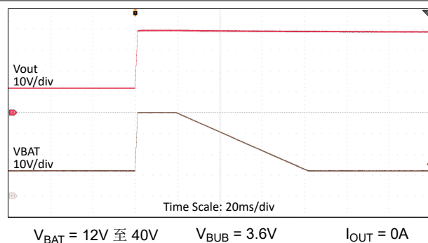
图 8-21. 12V 电池负载突降
