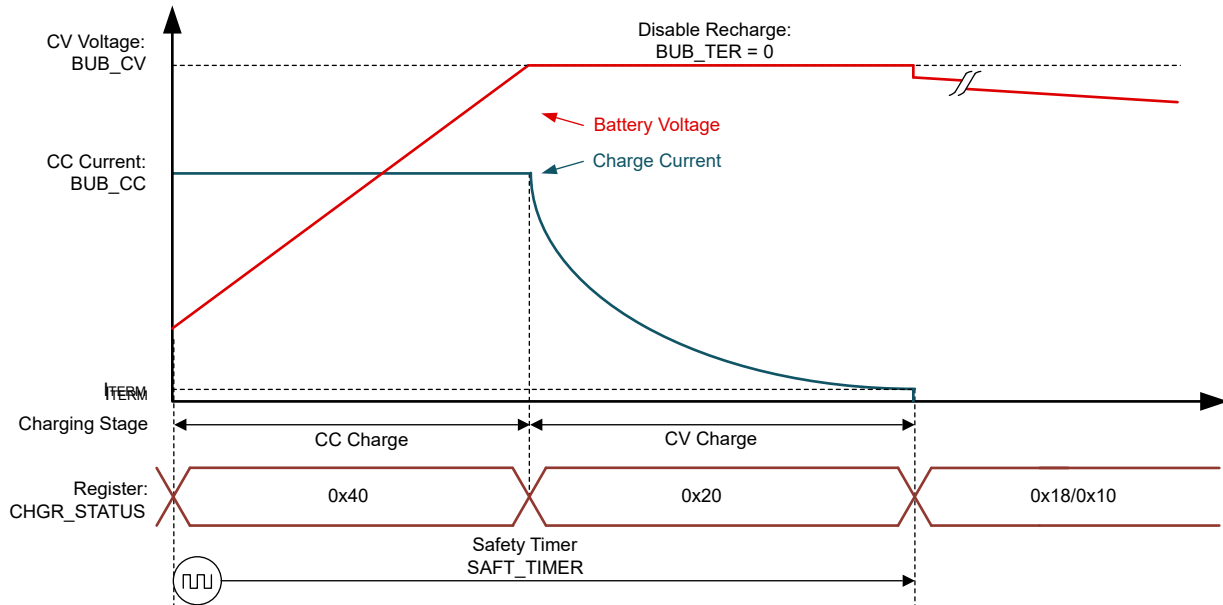
图 6-9. 超级电容器充电曲线，已禁用重新充电
