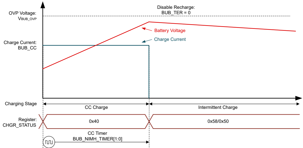
图 6-5. 禁用重新充电功能时的镍氢电池充电曲线
