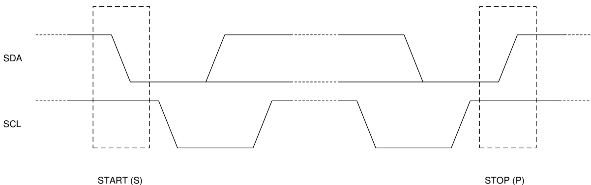
图 6-20. I 2 C START 和 STOP 条件
