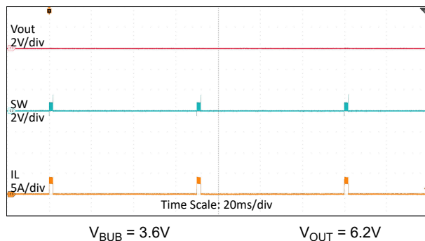
图 8-12. 升压输出短路断续
