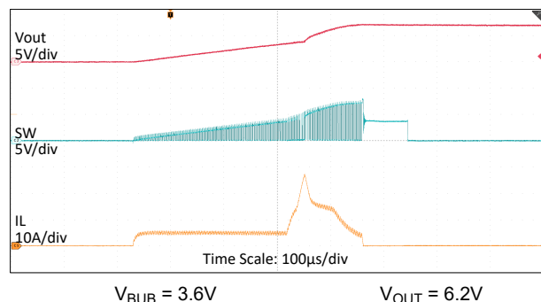
图 8-13. 升压输出短路恢复
