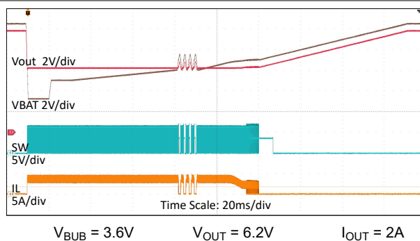
图 8-22. 12V 电池冷启动
