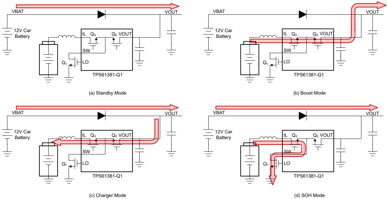
图 6-1. TPS61381-Q1 工作模式
