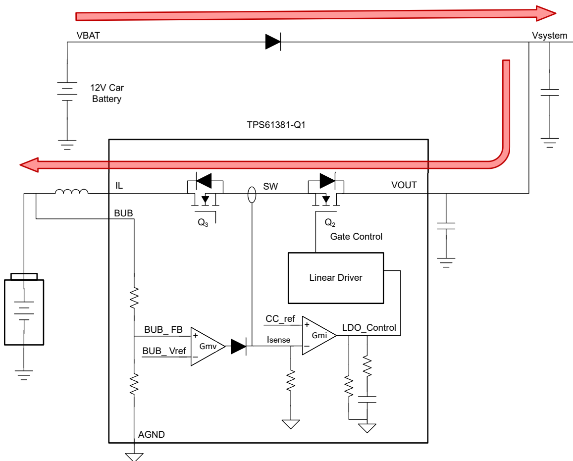
图 6-4. 线性充电器结构
