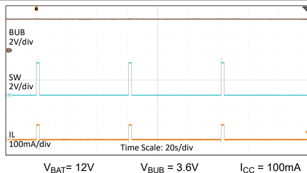
图 8-19. 镍氢电池间歇充电
