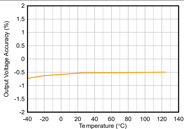
图 5-11. 输出电压精度与温度间的关系, FPWM, V_{BUB} = 3.6V , V_{OUT} = 6.2V
