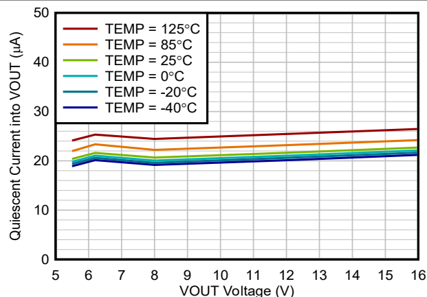
图 5-13. 流入 VOUT 的静态电流与 VOUT 电压间的关系, V_{BUB} = 3.6V
