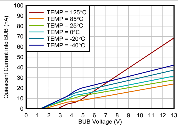
图 5-12. 流入 BUB 的静态电流与 BUB 电压间的关系, V_{OUT} = 12V
