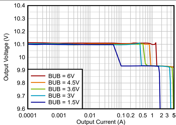
图 5-9. 输出电压与输出电流间的关系, V_{OUT} = 10V , PFM
