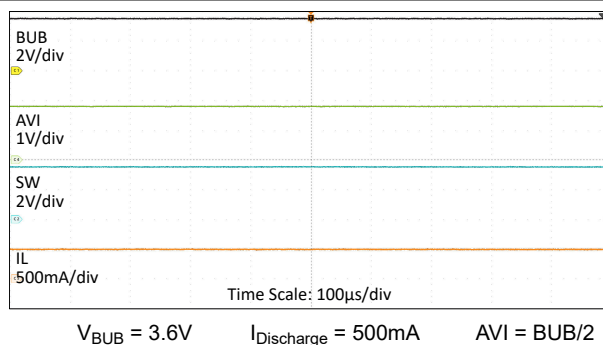
图 8-20. SOH 稳定状态
