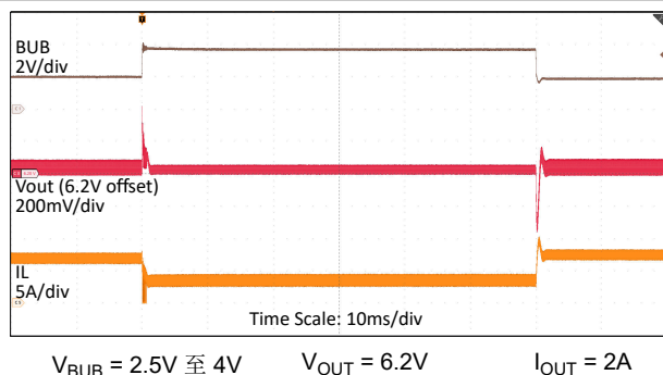
图 8-9. 升压模式下的线路瞬态
