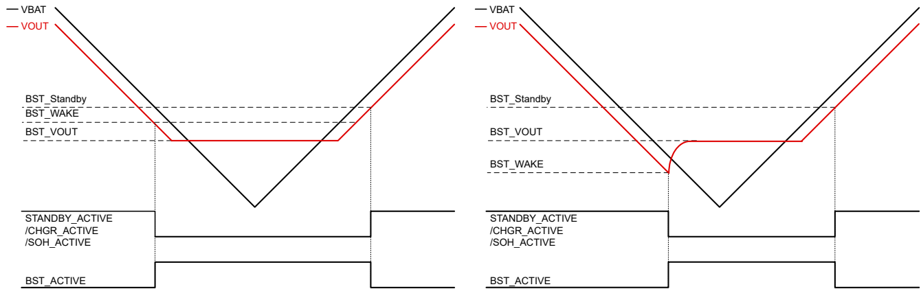
图 6-3. 自动升压和待机/充电器/SOH 切换逻辑
