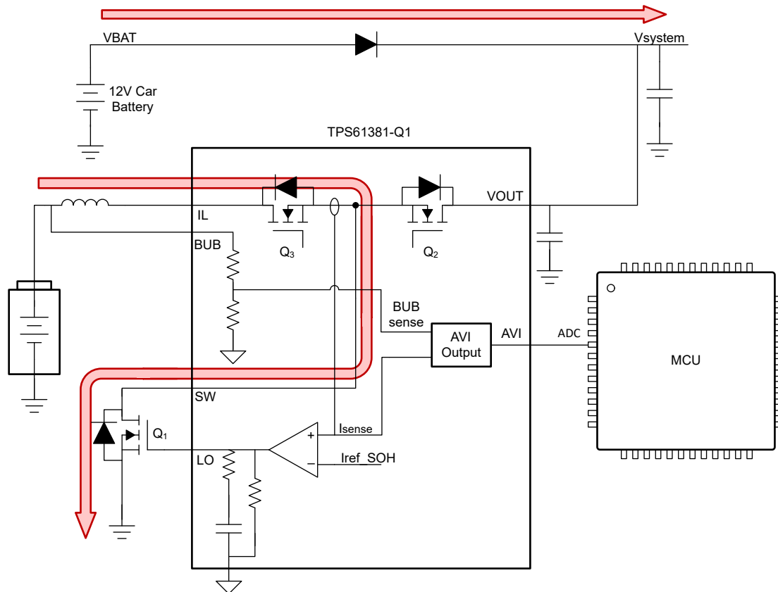
图 6-17. SOH 的典型操作
