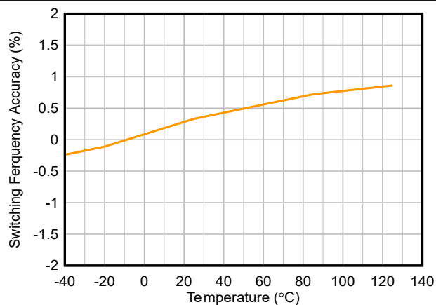
图 5-10. 开关频率与温度间的关系, FPWM, V_{BUB} = 3.6V , V_{OUT} = 6.2V
