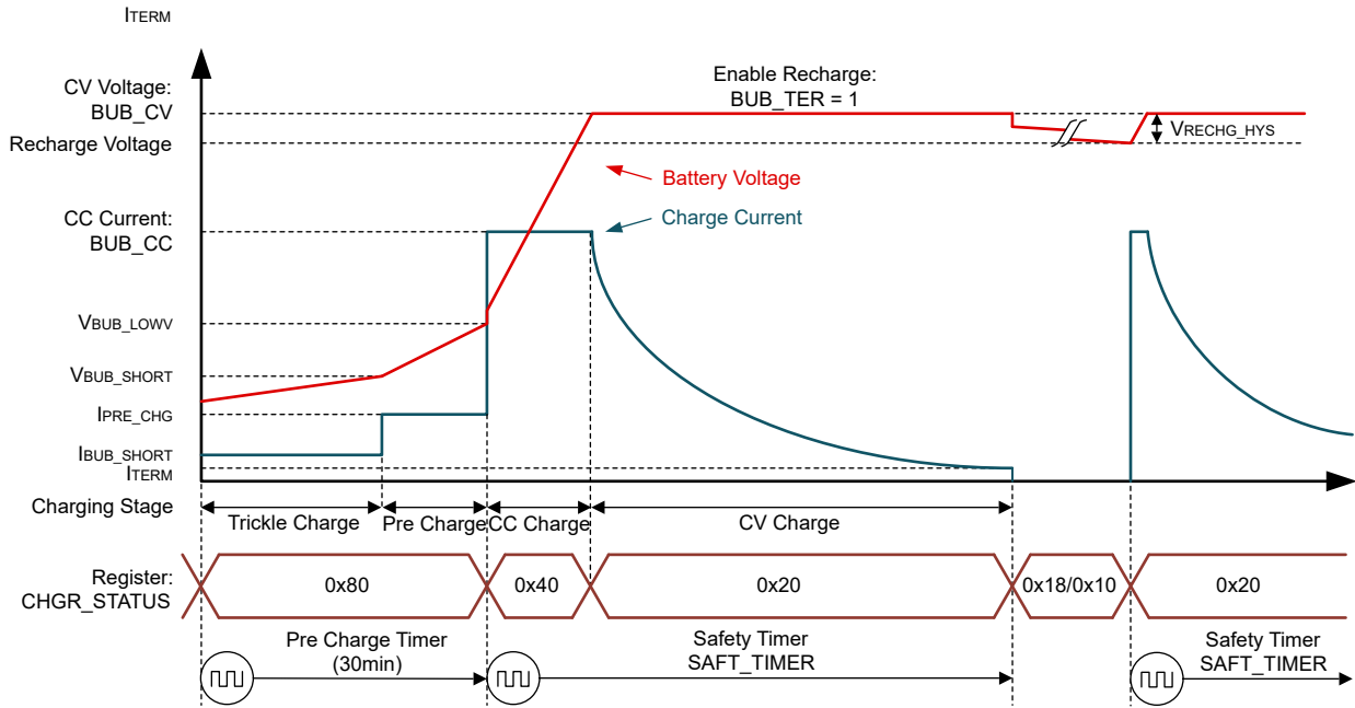
图 6-8. 启用重新充电功能时的锂基电池充电曲线
