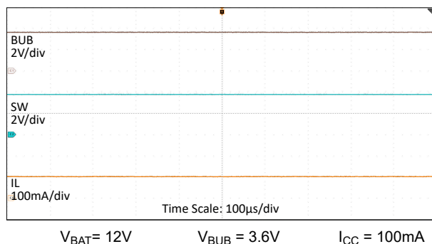
图 8-18. 充电器稳定状态
