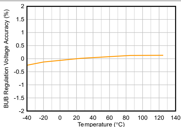
图 5-16. 电池调节电压精度与温度间的关系, I_{charge} = 100mA
