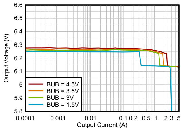
图 5-7. 输出电压与输出电流间的关系, V_{OUT} = 6.2V , PFM
