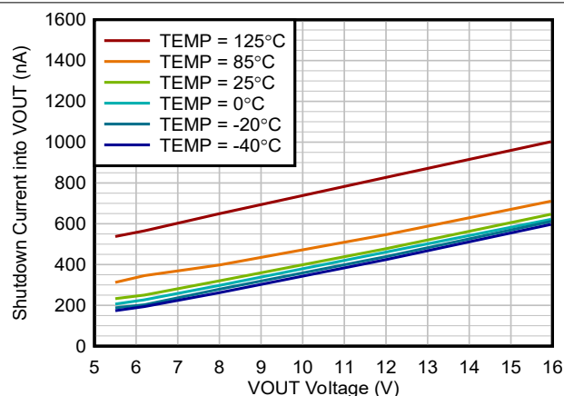
图 5-15. 流入 VOUT 的关断电流与 VOUT 电压间的关系, V_{BUB} = 3.6V
