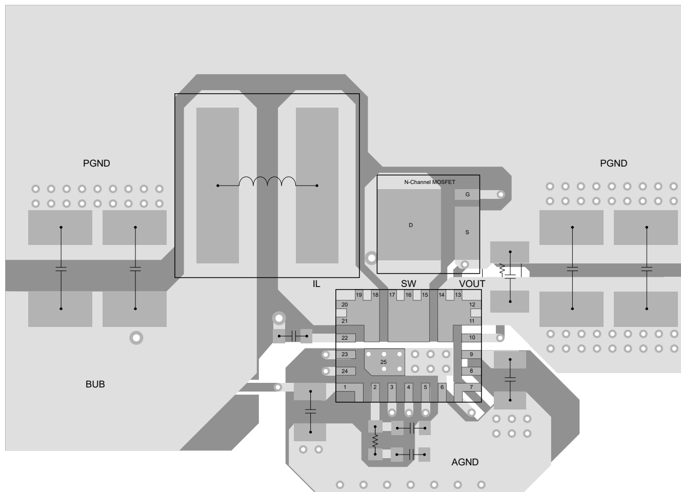
图 8-24. TPS61381Q 常见布局顶层
