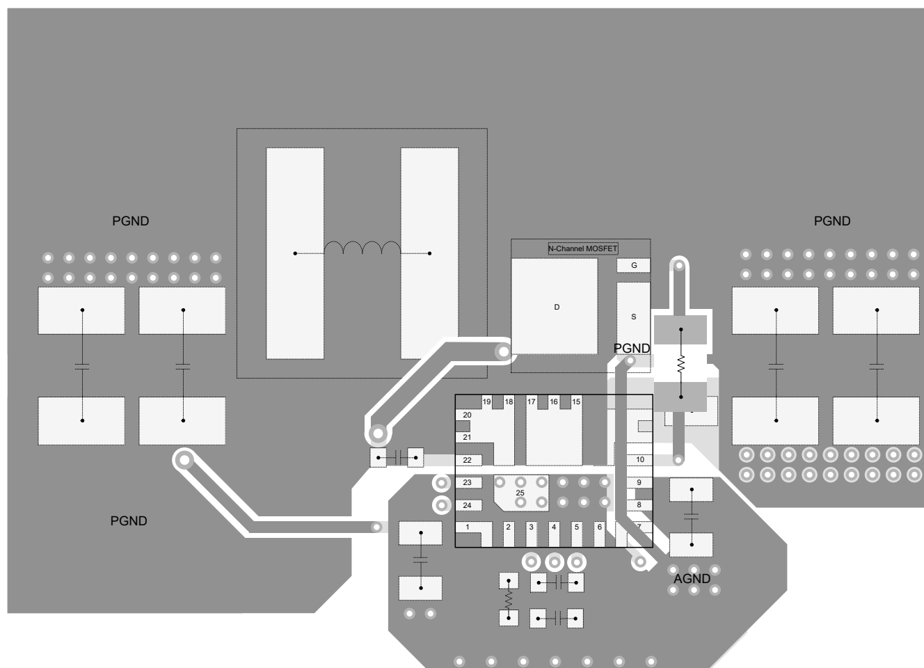
图 8-25. TPS61381Q 常见布局顶层到底层
