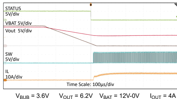
图 8-15. 切换到升压模式 (12V 电池中断)
