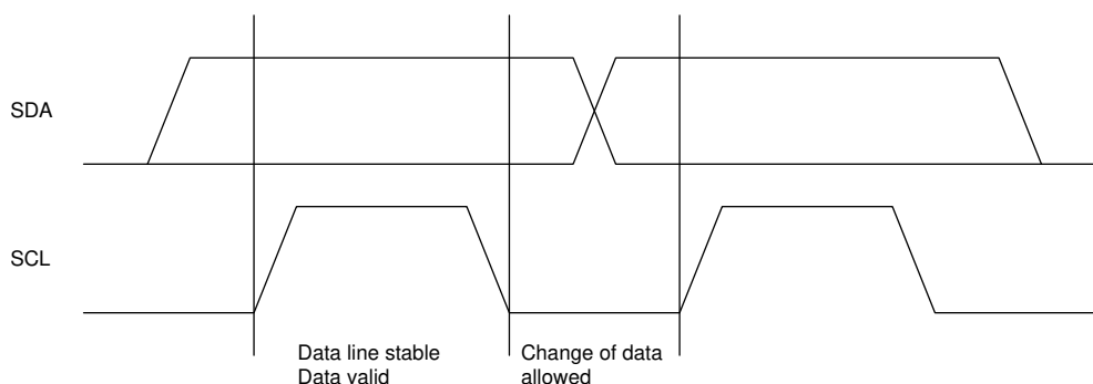
图 6-19. I 2 C 数据有效性
