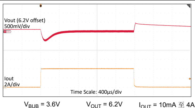
图 8-7. 升压模式下的负载瞬态
