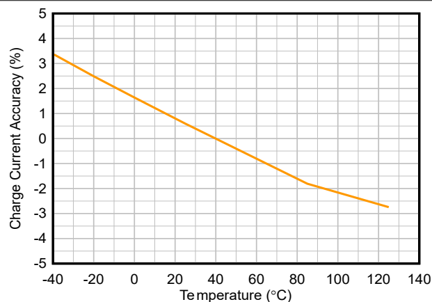
图 5-17. 充电电流精度与温度间的关系, I_{charge} = 100mA
