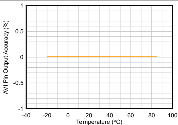
图 5-21. AVI 引脚 BUB 电压输出精度与温度间的关系, 比率 = 1
