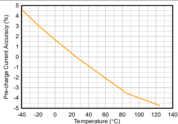
图 5-18. 预充电电流精度与温度间的关系
