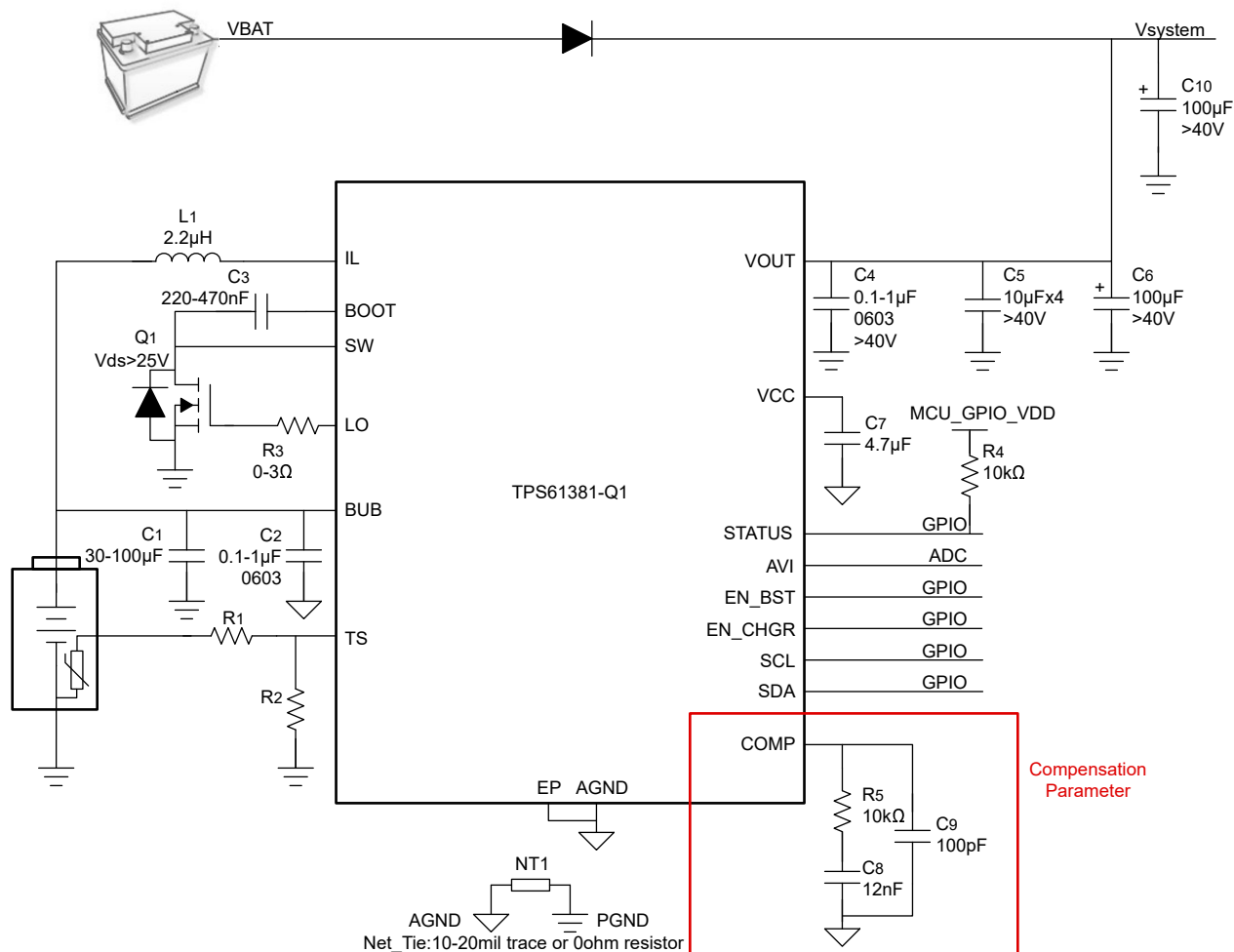
图 8-2. TPS61381-Q1 补偿设计
