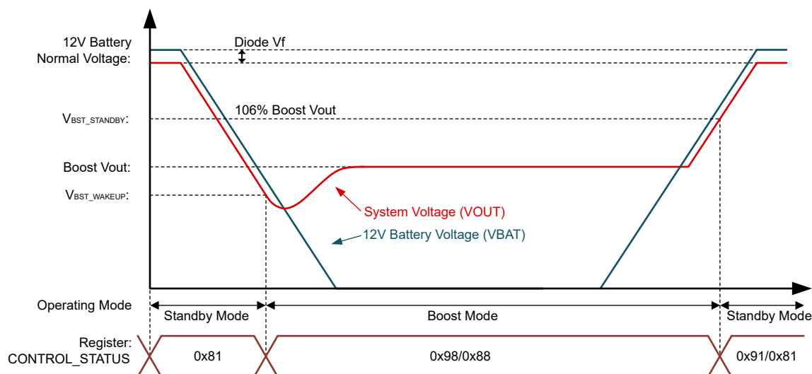
图 6-13. Case2： V_{\text{BST\_WAKEUP}} < \text{BST\_VOUT}
