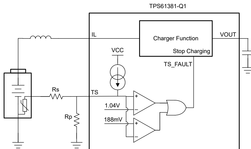
图 6-11. 用于修改后温度窗口的 TS 电阻网络
