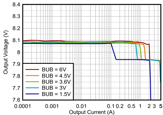
图 5-8. 输出电压与输出电流间的关系, V_{OUT} = 8V , PFM
