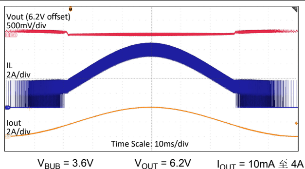
图 8-8. 升压模式下的负载扫描
