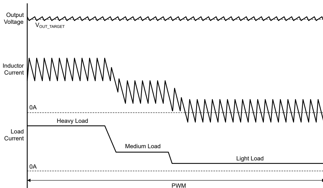
图 6-16. PWM 和 PFM 运行
