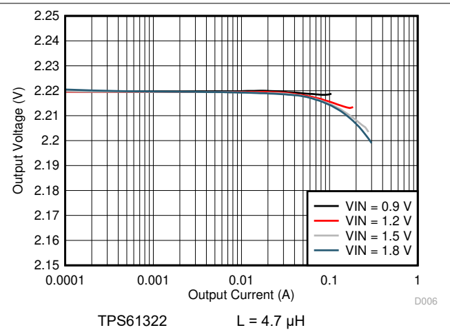
图 6-2. Load Regulation
