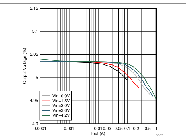
图 6-4. Load Regulation
