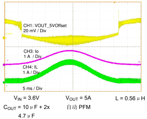
图 8-5. 负载扫描
