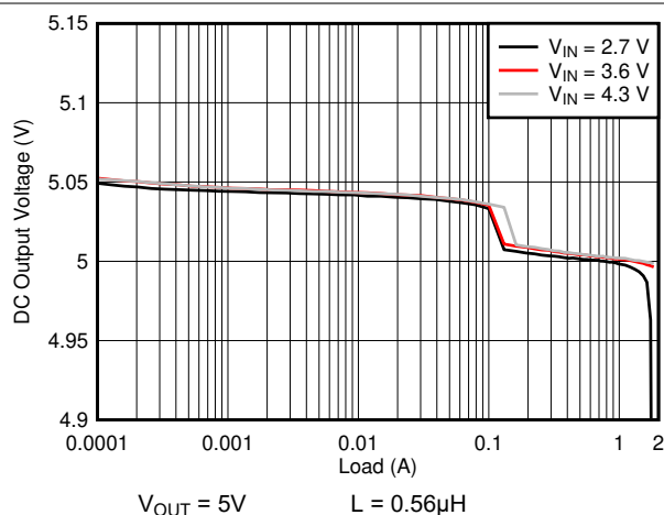
图 6-3. DC 输出电压与负载间的关系
