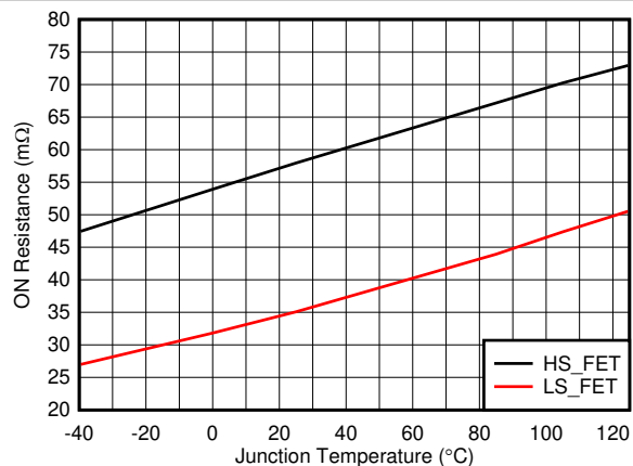
图 6-5. R_{DS(ON)} 与温度间的关系
