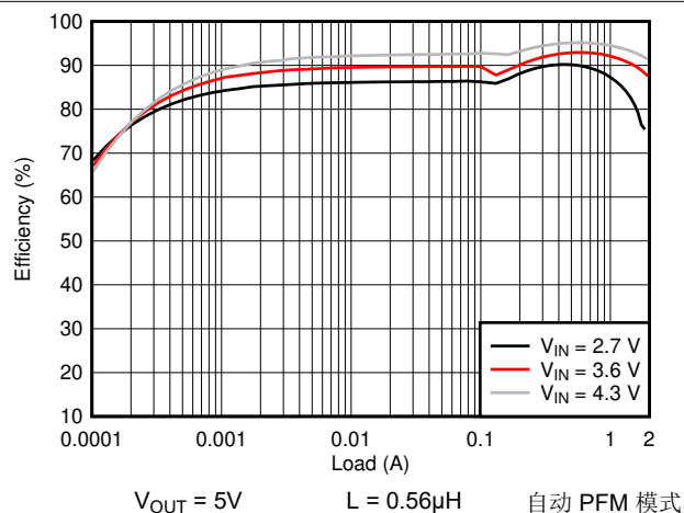
图 6-1. 效率与负载间的关系
