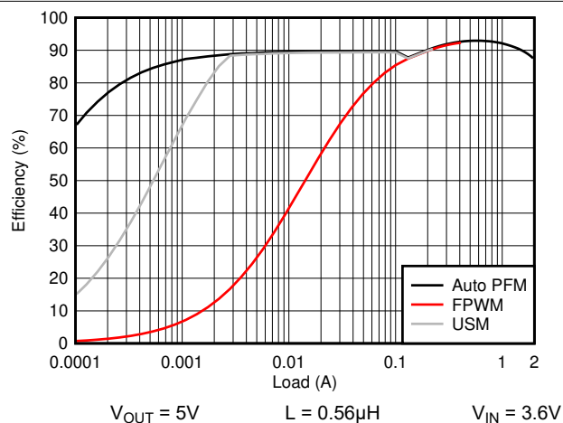
图 6-2. 效率与负载间的关系
