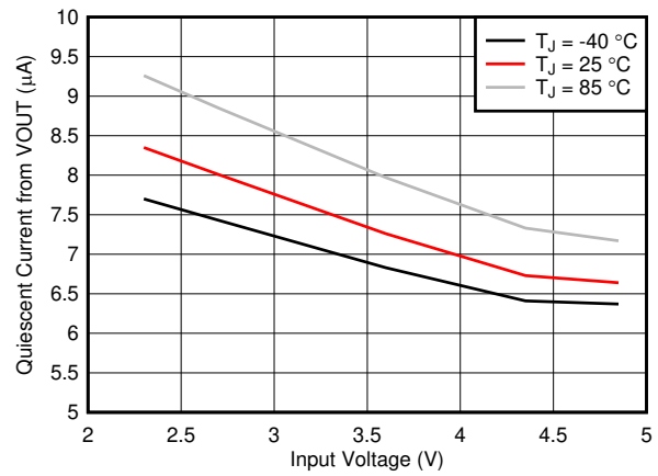
图 6-8. 静态电流 (来自 VOUT) 与输入电压间的关系
