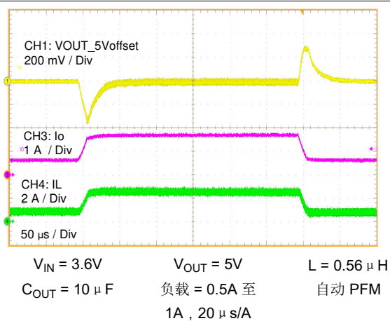
图 8-8. 10 \mu F C_{OUT} 的负载瞬态
