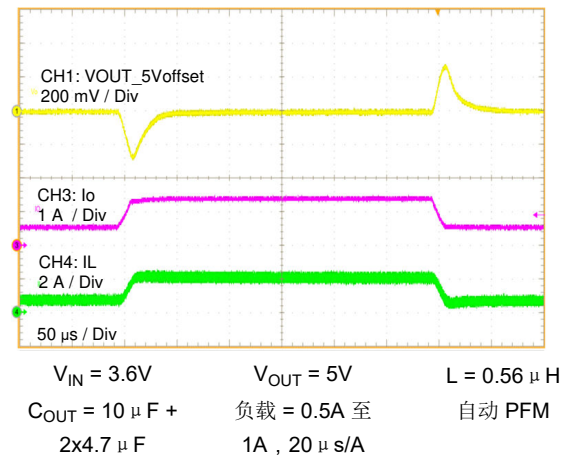
图 8-7. 负载瞬态
