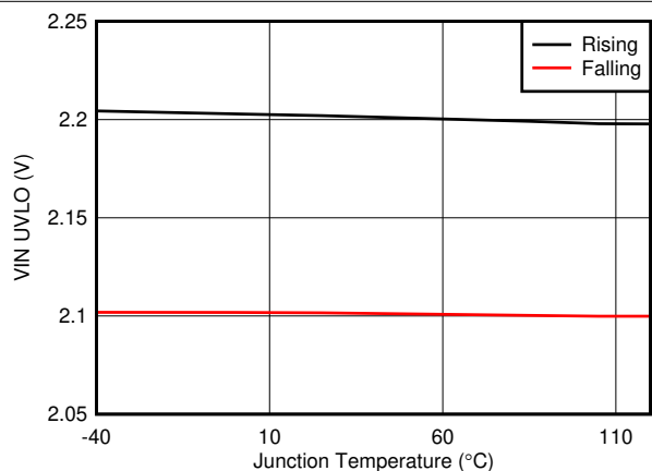
图 6-16. VIN UVLO 与温度间的关系
