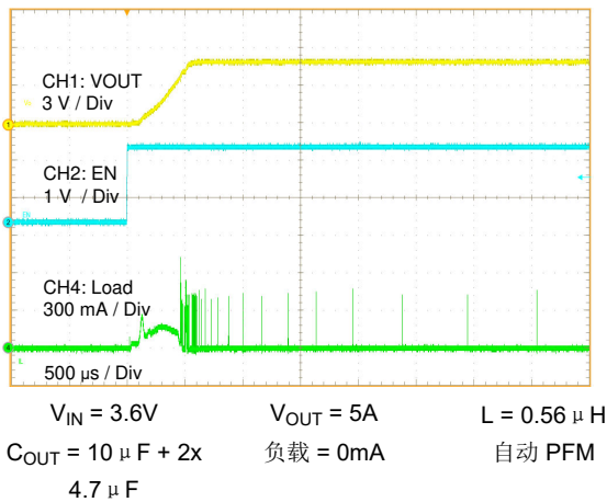
图 8-6. 由 EN 启动
