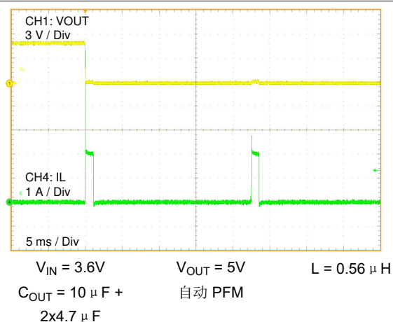
图 8-9. 短路输出
