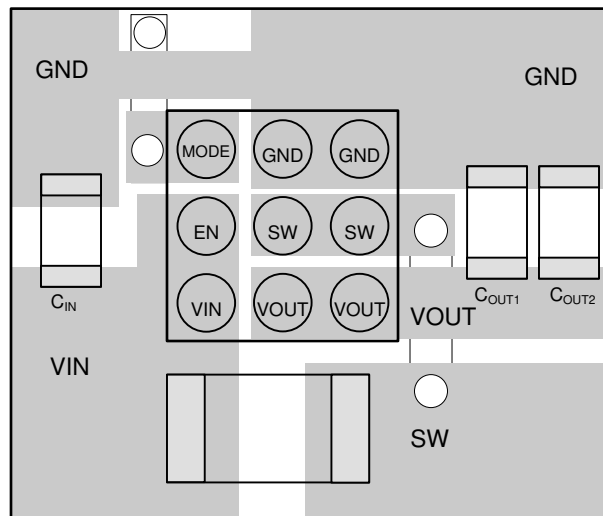
图 8-11. 建议布局
