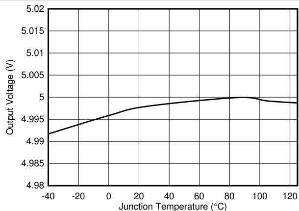
图 6-6. V_{OUT} 与温度间的关系
