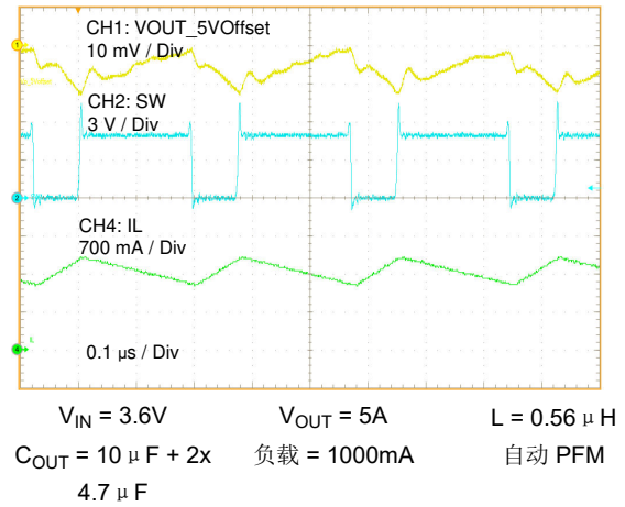
图 8-3. 稳定 1000mA
