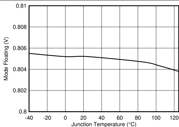
图 6-15. 模式悬空与温度间的关系
