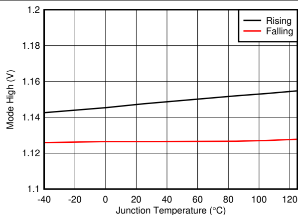
图 6-13. 模式高电平上升/下降与温度间的关系
