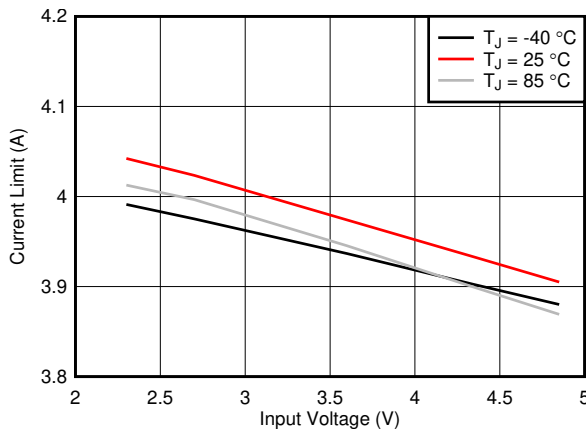
图 6-11. 电流限制 (强制 PWM) 与输入电压间的关系
