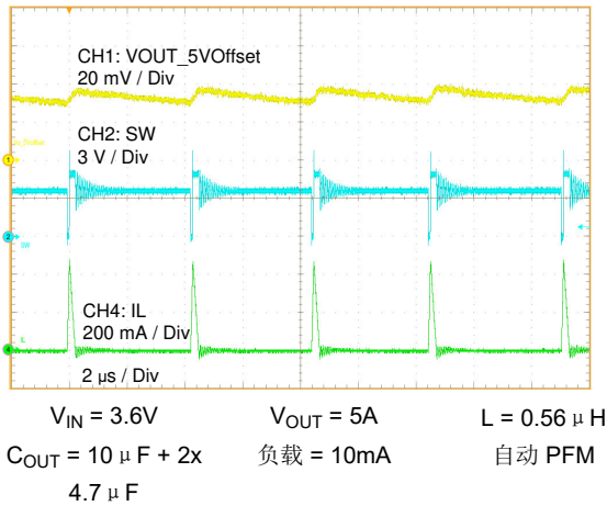
图 8-2. 稳定 10mA
